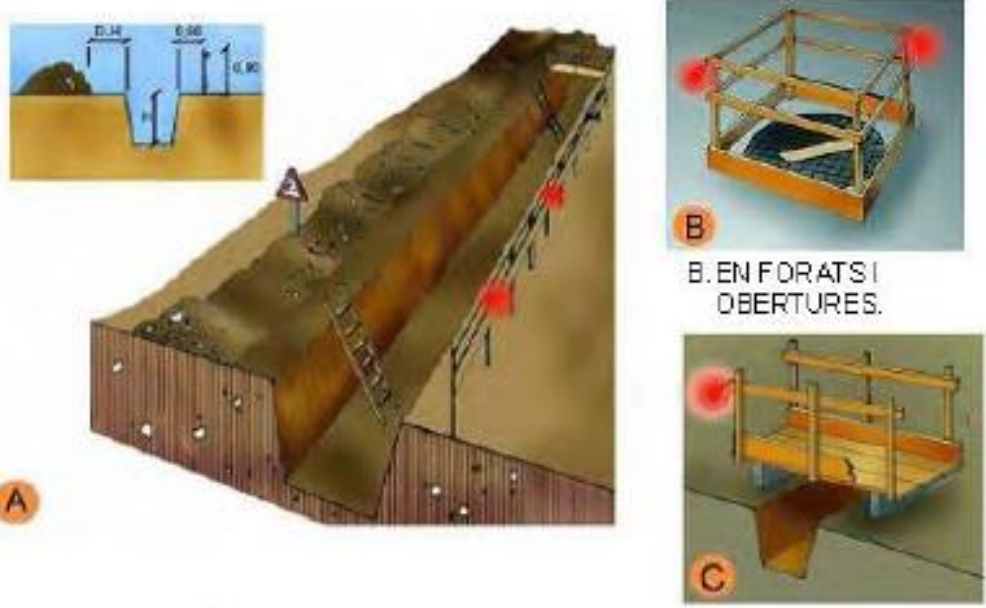
A. PROTECCIÓ EN RASES. B. EN FORATS I OBERTURES. C. DETALL PASARELLA VIANANTS.
