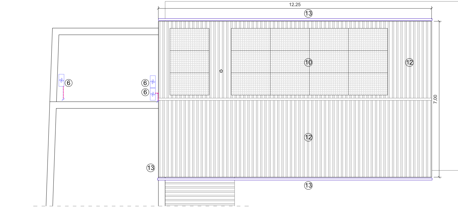
COBERTA
