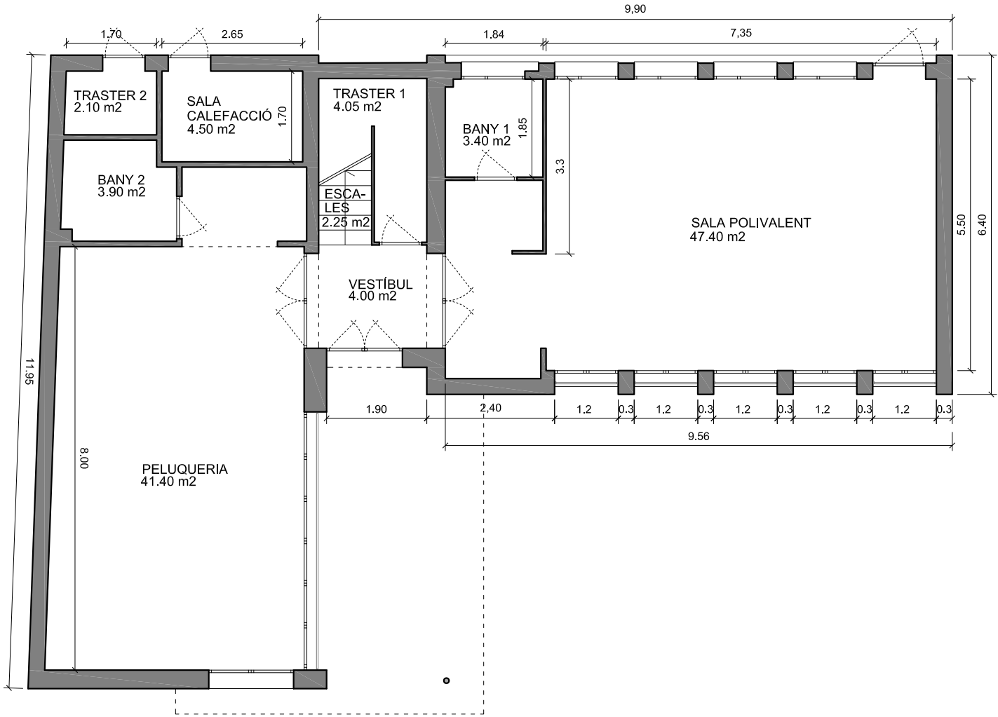
PLANTA BAIXA
