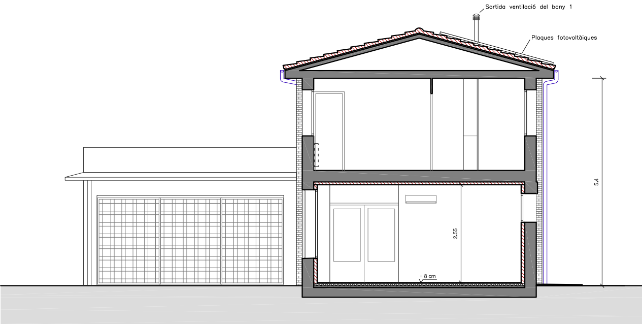
SECCIÓ
