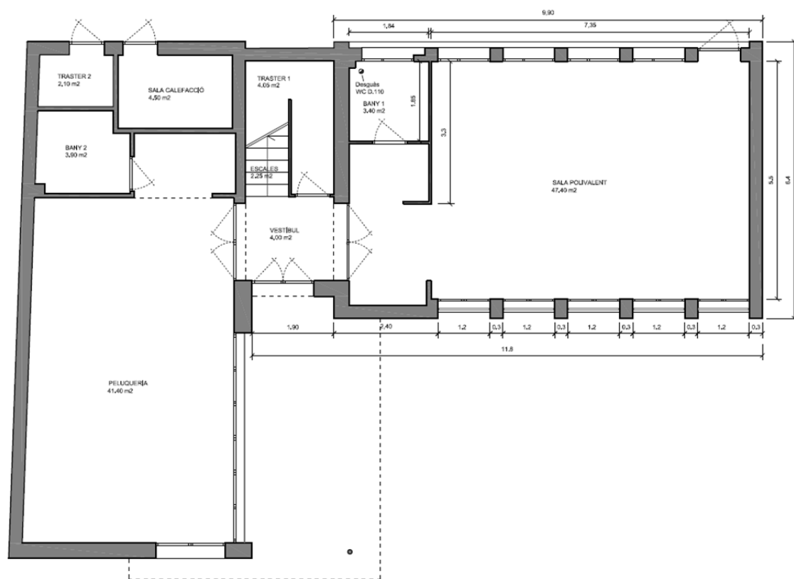
PLANTA BAIXA
