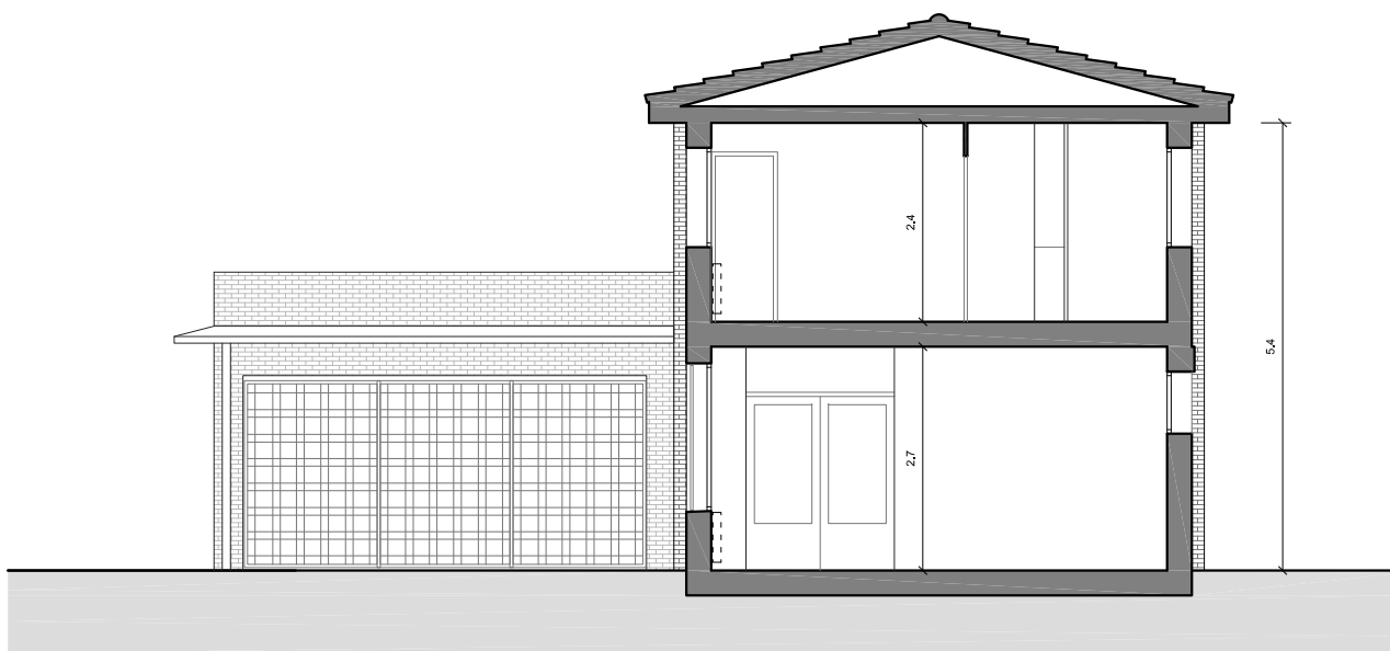
SECCIÓ
