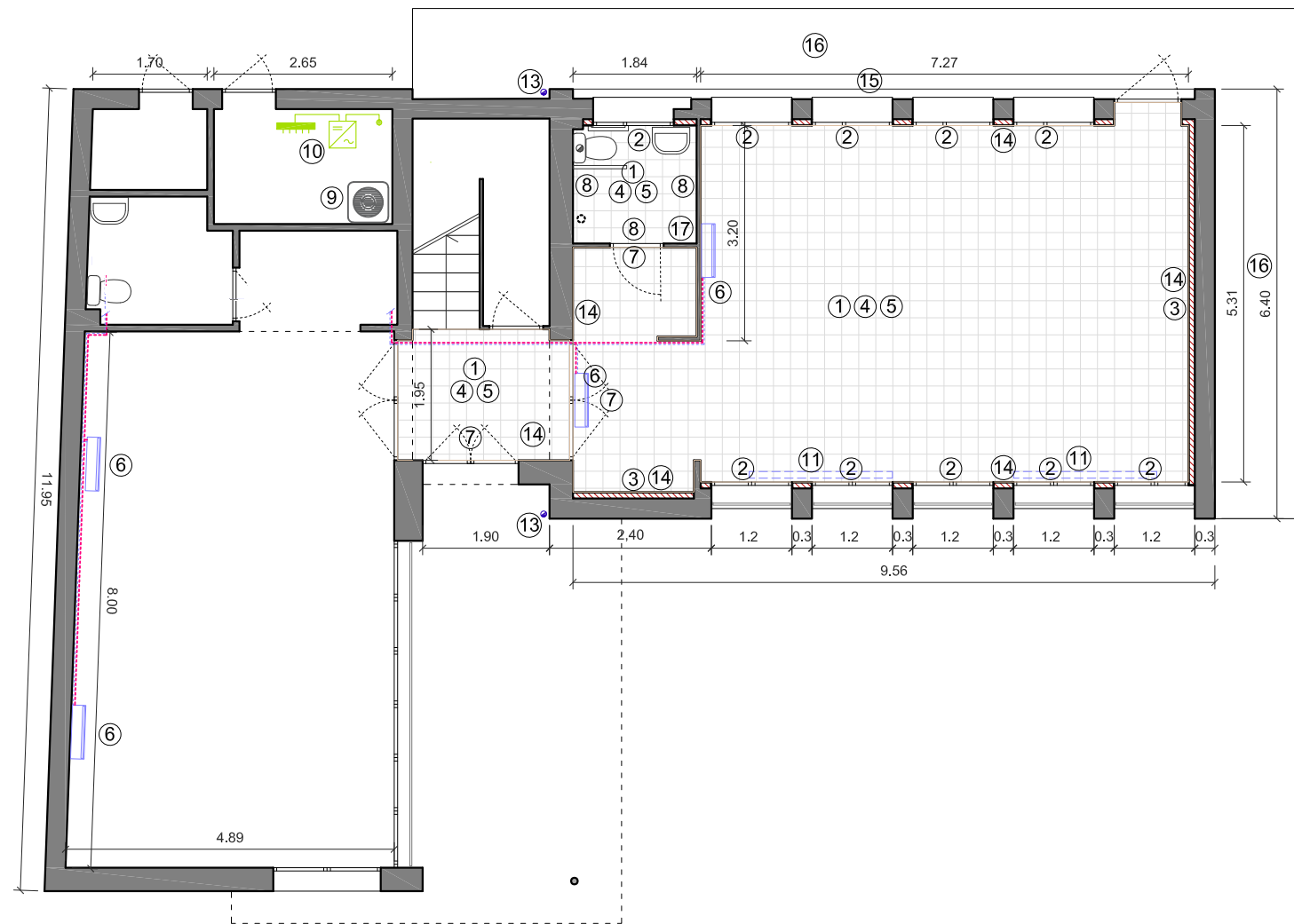
PLANTA BAIXA
