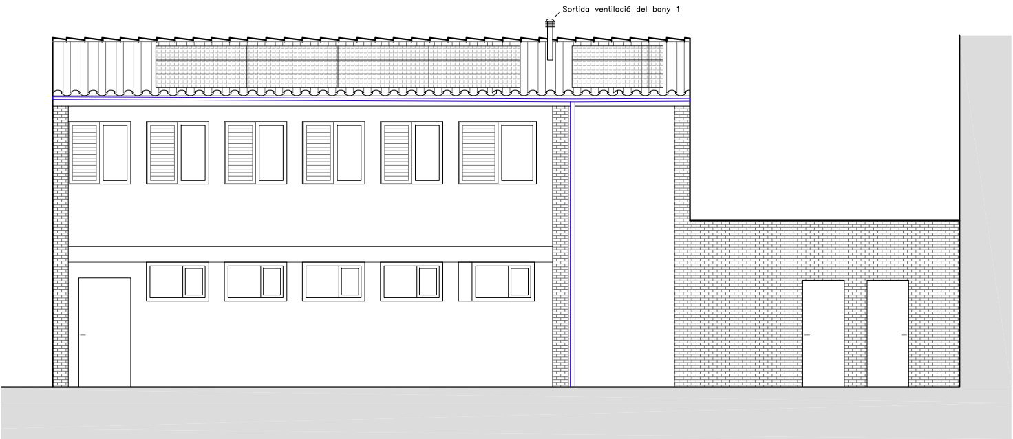
ALÇAT POSTERIOR
