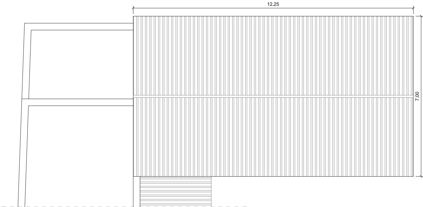
COBERTA
