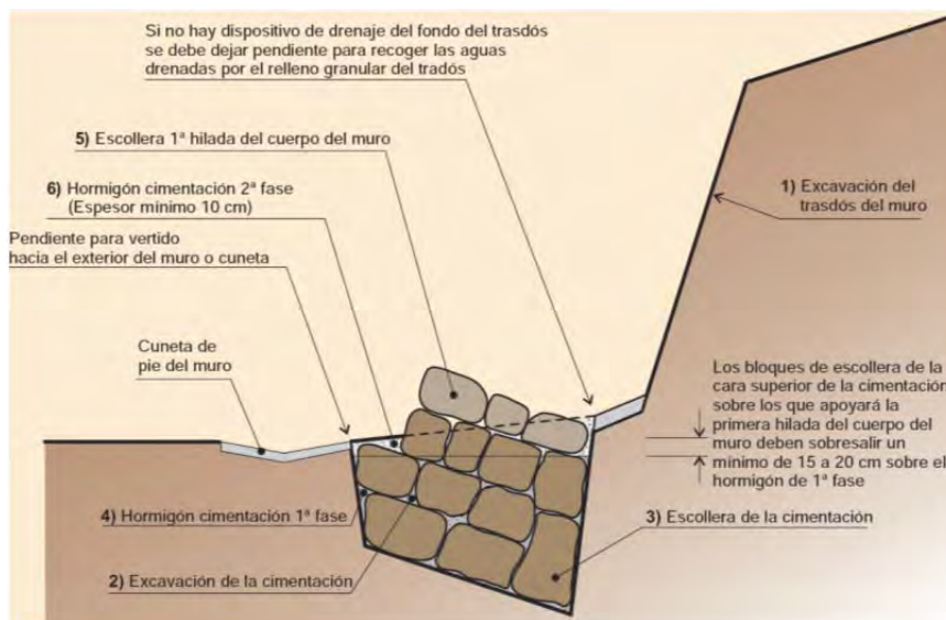
Fases d'execució dels fonaments
