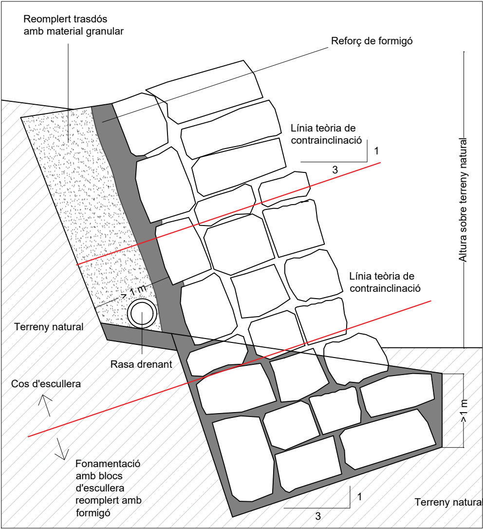
Detall Mur d'escullera E: 1/50
