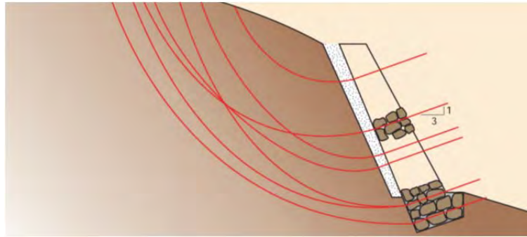
Reomplert cos del mur. Exemple de superfície de lliscament per l'anàlisi de l'estabilitat.
