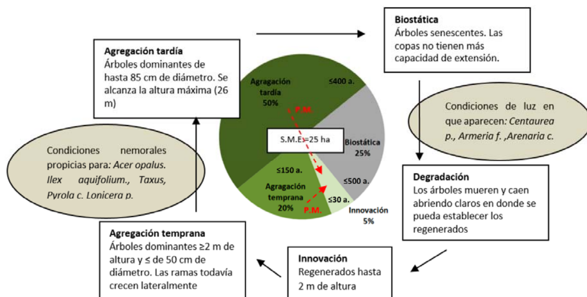
Figura 1. Model de cicle forestal per a boscos de Pinus nigra subsp. salzmannii a l'espai i el temps amb indicació de les fases que el componen, els criteris utilitzats per definir-les i el nínxol de les espècies acompanyants objecte de conservació. Els sectors del gràfic circular són proporcionals a la representació superficial de cada fase del cicle. SME = Superfície mínima d'equilibri; PM = Pertorbacions menors que renoven el vol i escurcen el cicle. S'indica per a cada fase l'edat màxima dels arbres a partir de la qual passarien a la fase següent, p.e. Fase d'innovació arbres de menys de 30 anys. (adaptat a partir de Tíscar, 2015).
