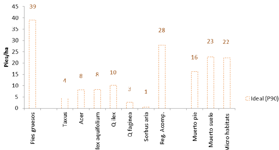
Figura 2. Valors llindars per a cadascun dels elements estructurals d'interès per a la maduresa i la naturalitat forestal establerta a partir de l'anàlisi de 14 rodals forestals a la zona del Parc Natural dels Ports.
