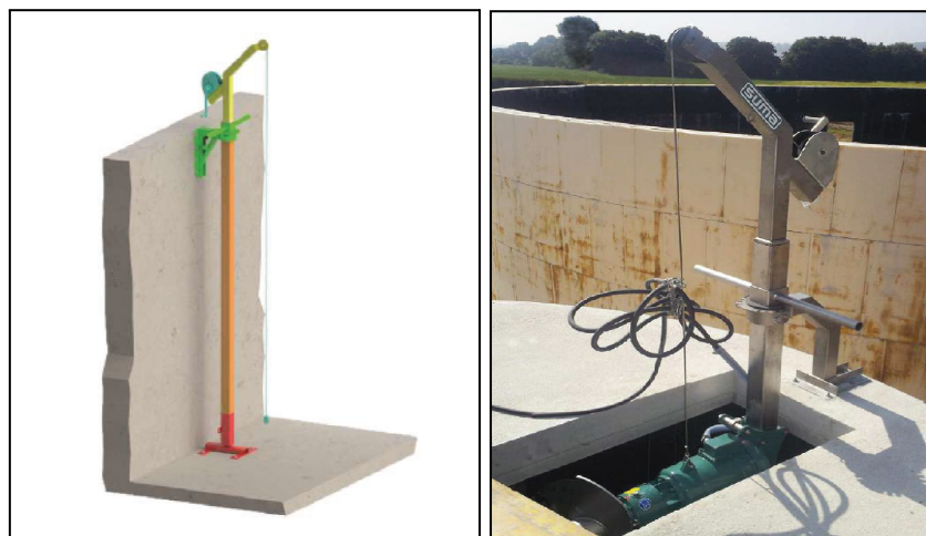
Imatge 4.- Exemple de fixació en mur lateral per a dipòsits elevats.
