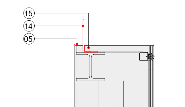
DETALL BARANA PERÍMETRE
