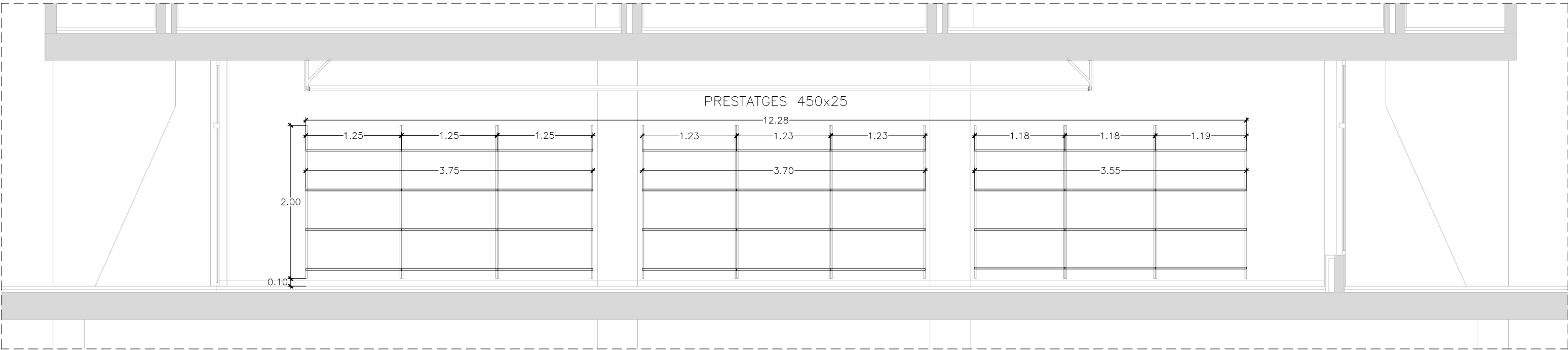
PRESTATGES CRÈMALLERA ZONA TAULES TALLER
