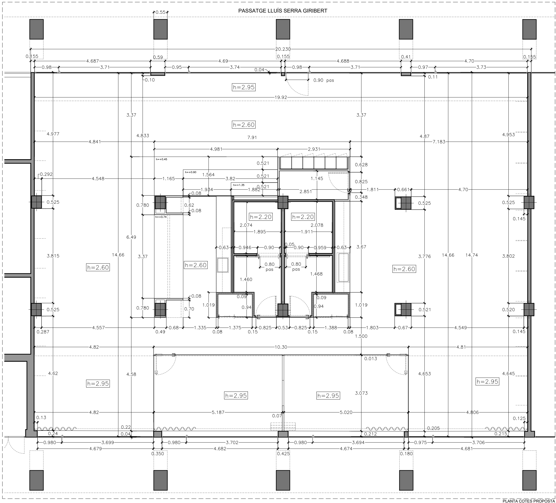
PLANTA COTES PROPOSTA
