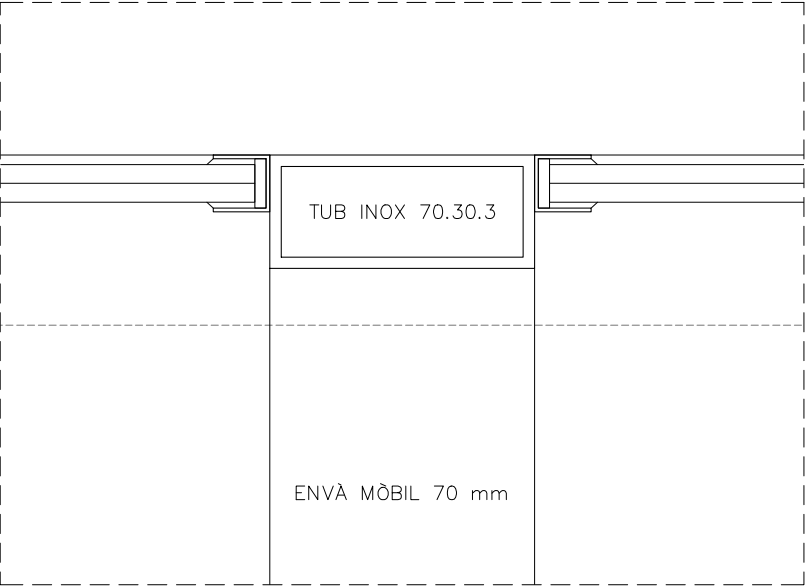
PLANTA DETALL VIDRE SEPARACIÓ OFFICE 1:2
