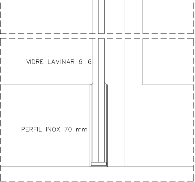
SECCIÓ DETALL VIDRE SEPARACIÓ OFFICE 1:2
