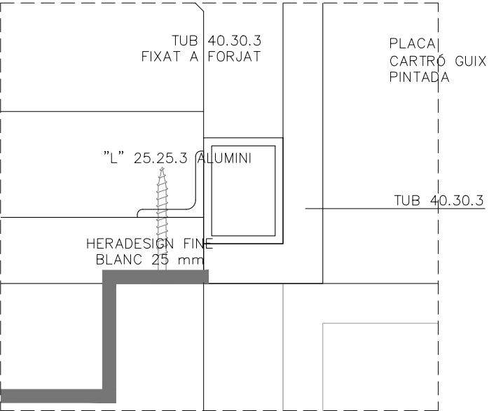
SECCIÓ DETALL TABICA PLADUR-HERADESIGN 1:2
