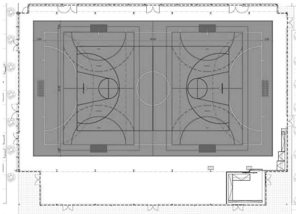
Plànol de la pista de joc. Font: Santamaria Arquitectes
