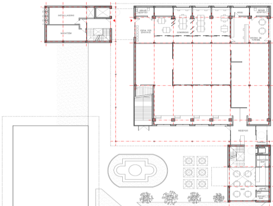
Planta baixa Edifici Tabaris.
