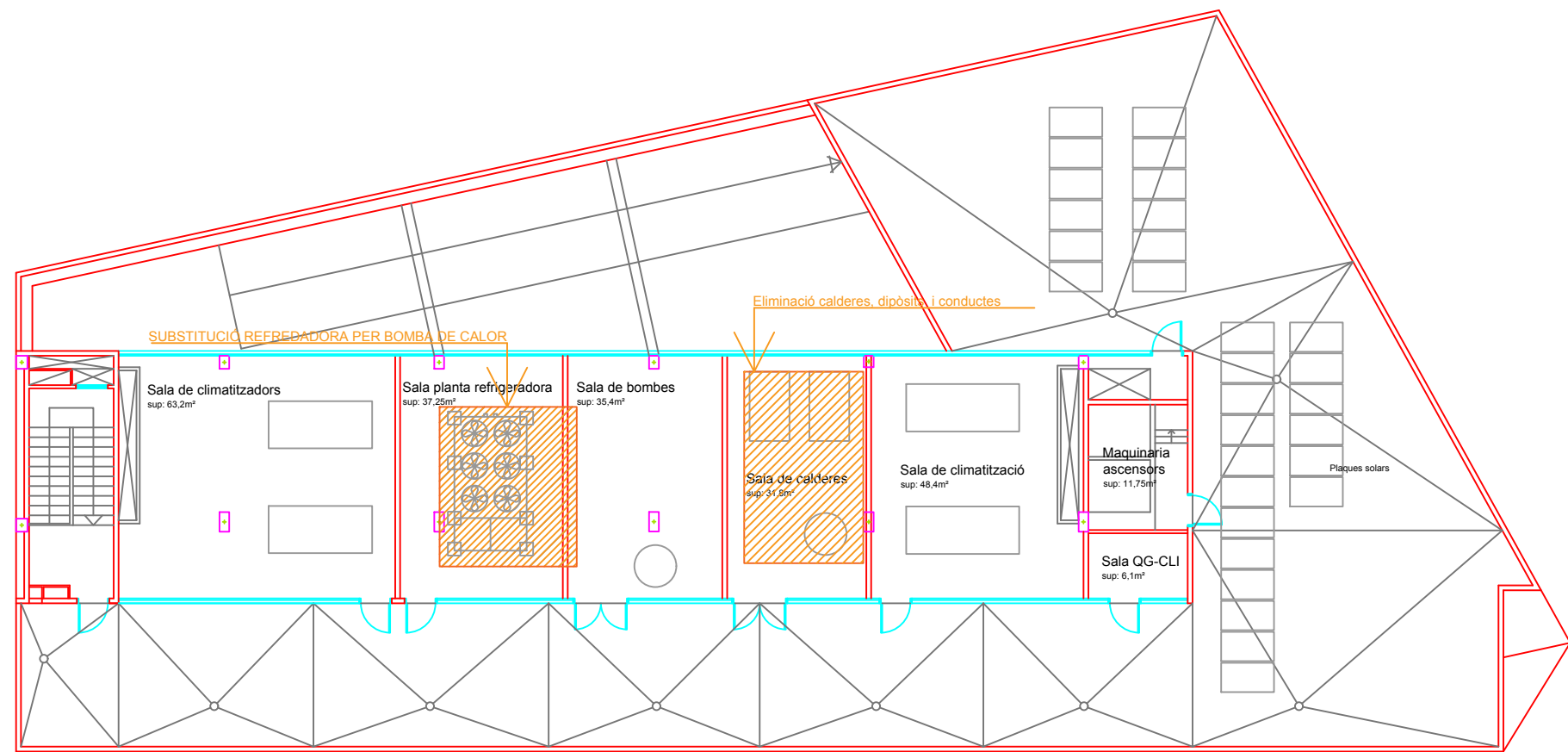
Planta instal·lacions
