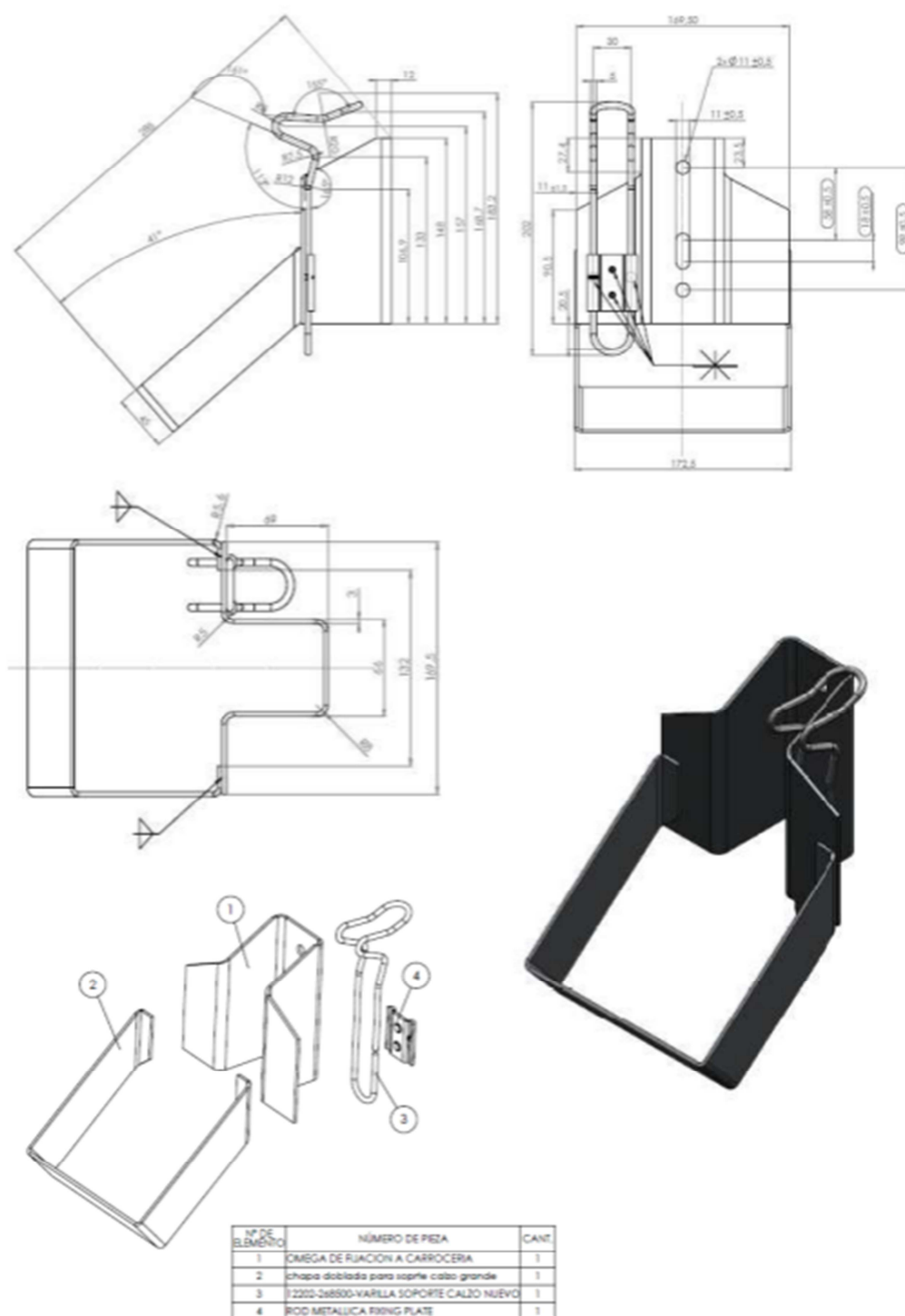
Figura 5. Soporte calzo
