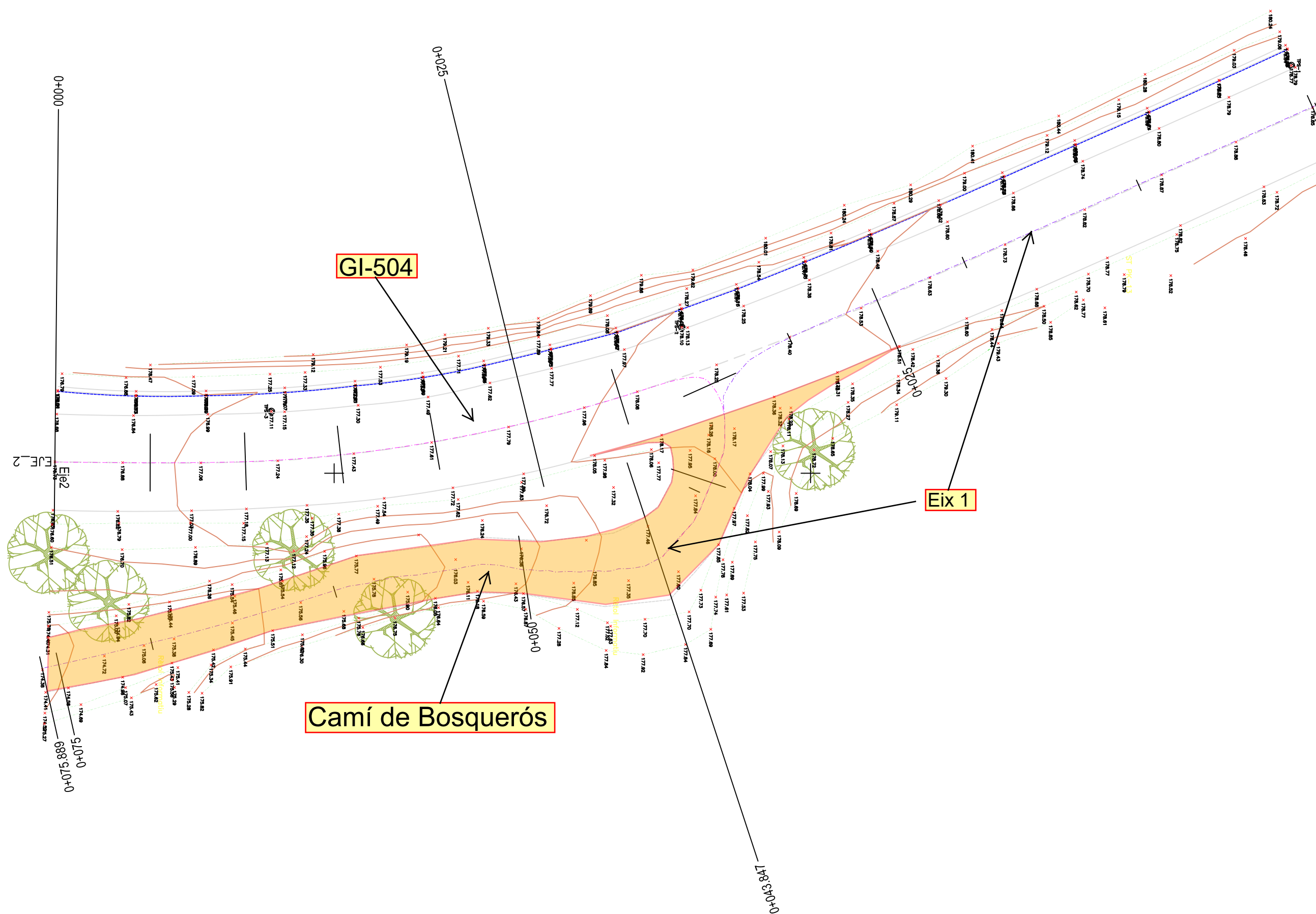
Planta traçat accés camí de Bosquerós a la carretera GI-504
