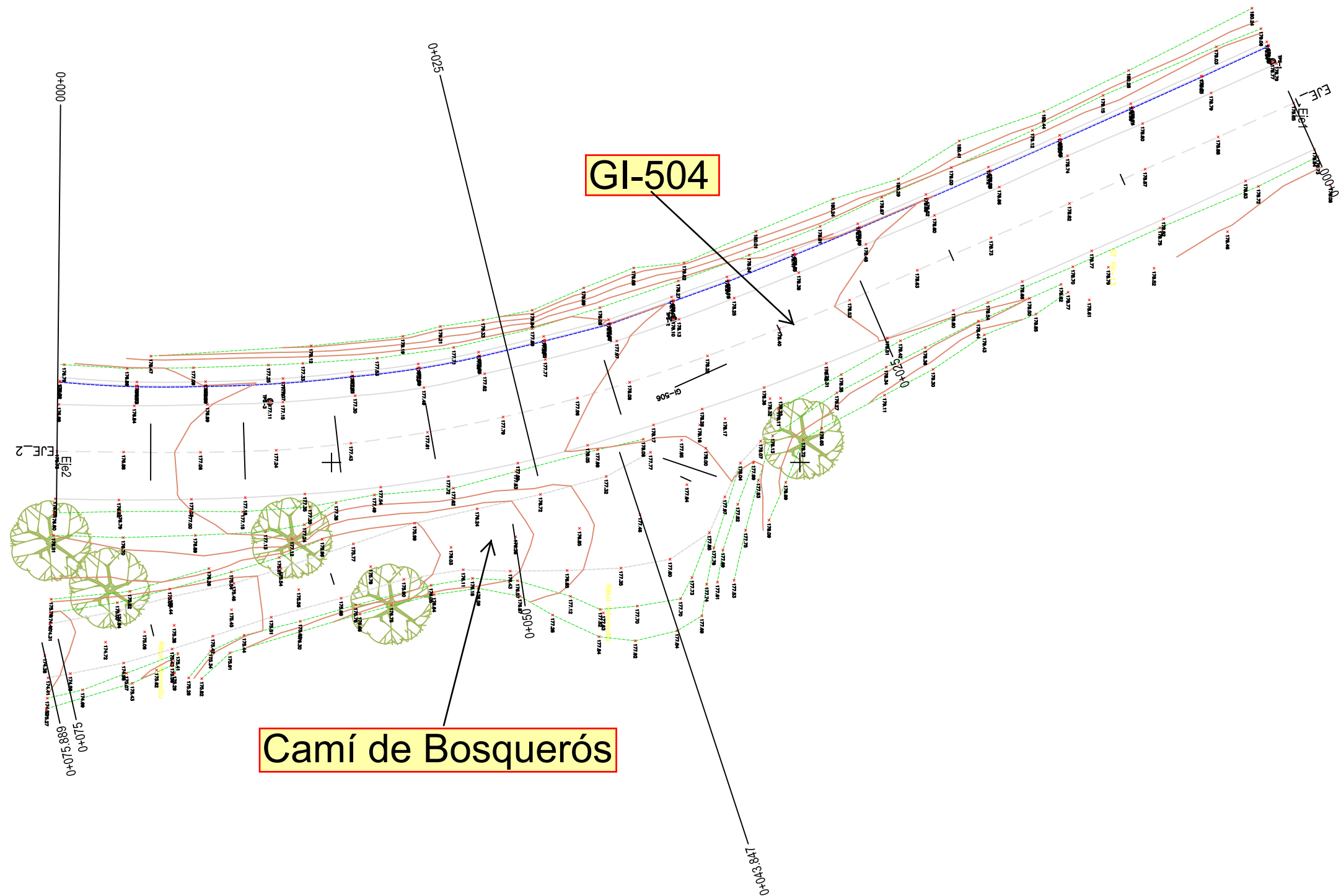
Topogràfic estat actual de l'accés del camí de Bosquerós a la carretera GI-504
