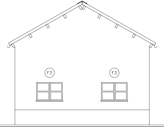
FAÇANA NORD
