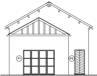
ALÇATS PROPOSTA
