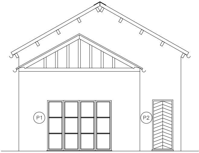
FAÇANA SUD
