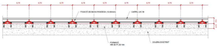
SECCIÓ LONGITUDINAL E. A1 1/15 E. A3 1/30
