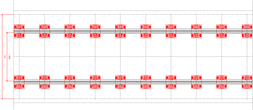
PLANTA E. A1 1/15 E. A3 1/30
