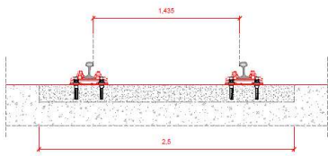
SECCIÓ TRANSVERSAL E. A1 1/15 E. A3 1/30
