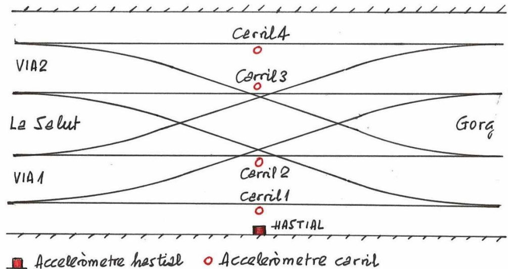
Fig. 1 - Col·locació dels acceleròmetres a la bretelle
