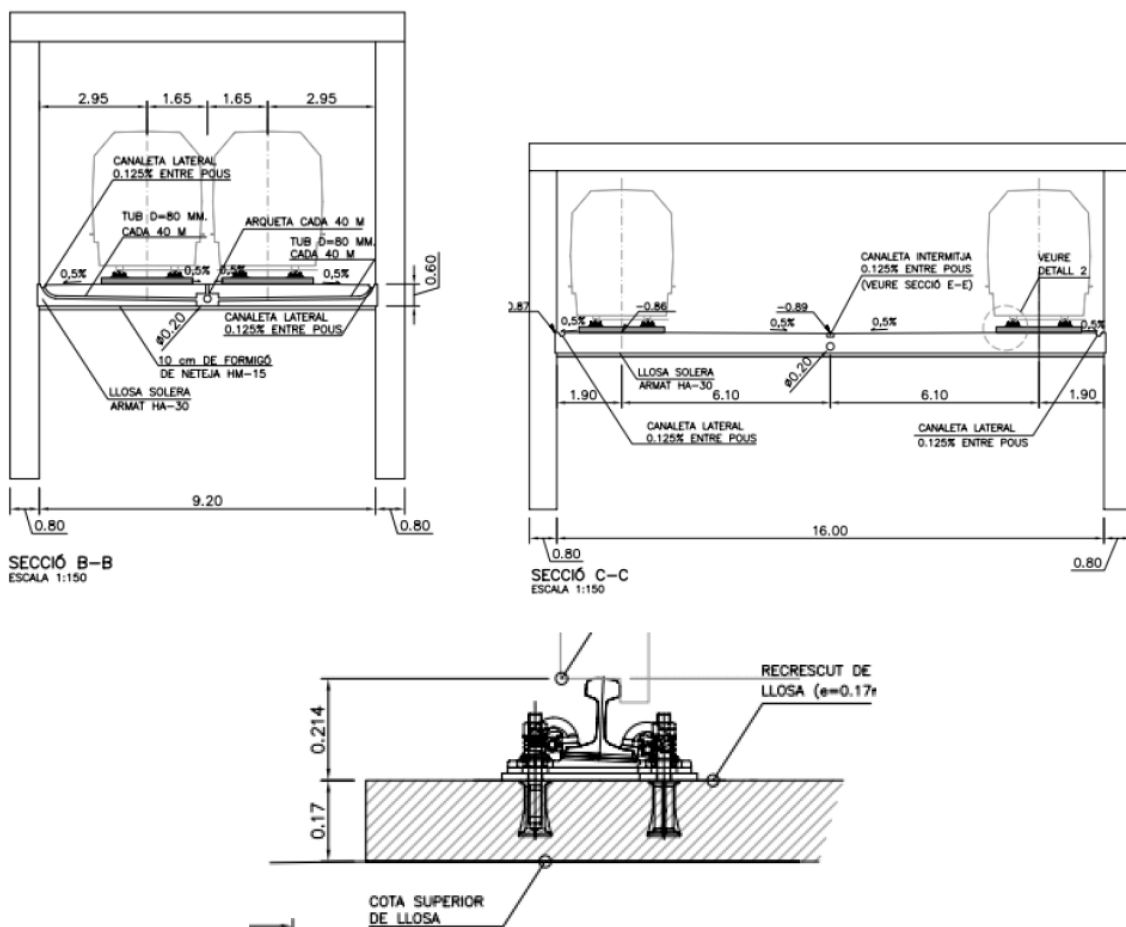
Secció de superestructura en la zona de projecte. Font: TM-00509.3 O.E.
