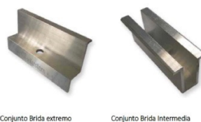
Figura 1. Detalle Bidas Fijación Placas PV
