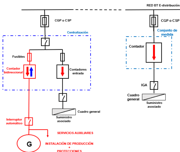
Esquema tipus 15 de la Guia NRZ105 Endesa Distribución,SLU
