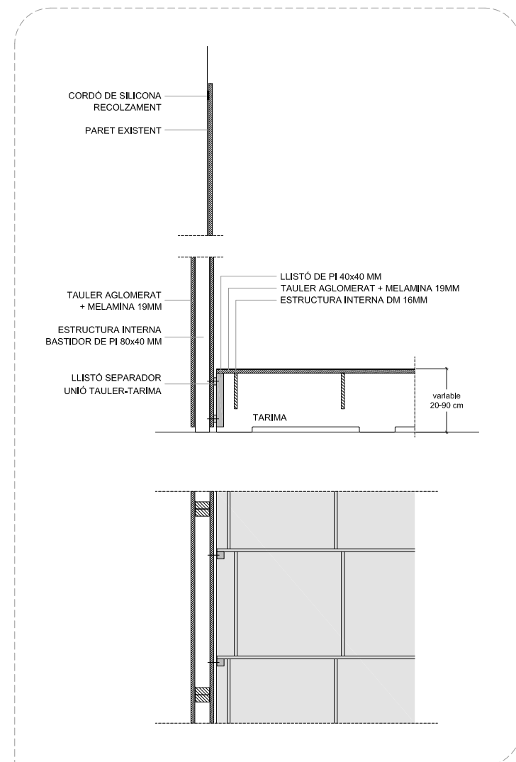
DETALL SUBJECCIÓ PARAMENTS I REVESTIMENTS A TARIMES
