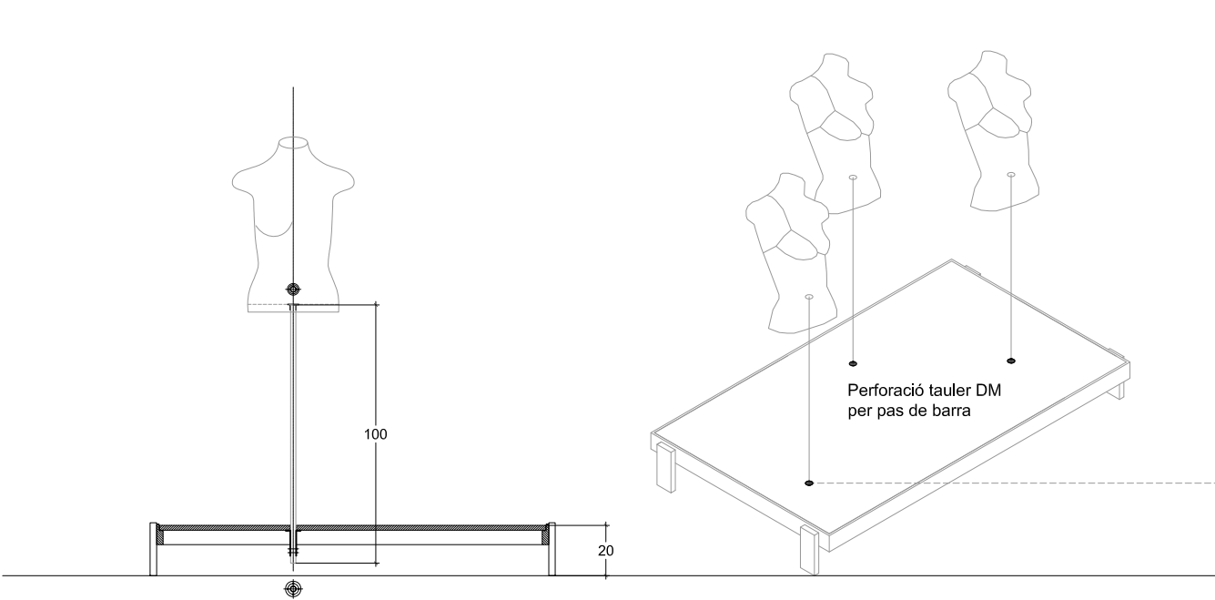
ÀMBIT 2 CONJUNT PECES (A I B) PER A SUBJECCIÓ BARRA MANIQUÍ EXISTENT DIÀMETRE 20MM.
