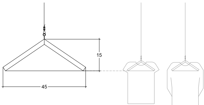
ÀMBIT 2 PENJADOR PER SAMARRETA I JERSEI AMB SISTEMA DE SUBJECCIÓ A SOSTRE TÈCNIC. LLISTÓ DE FUSTA DE FAIG BLANC 2.5x1 CM.
