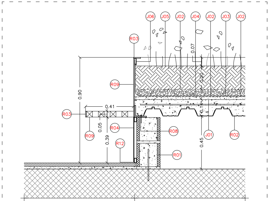
SECCIÓ H-H'
