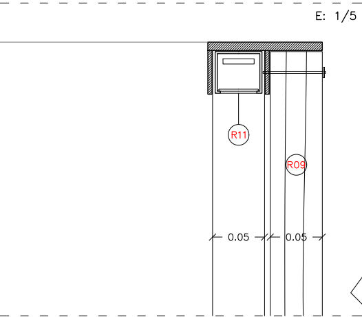
DETALL D03
