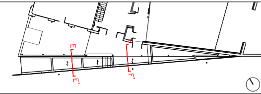
DETALL D04
