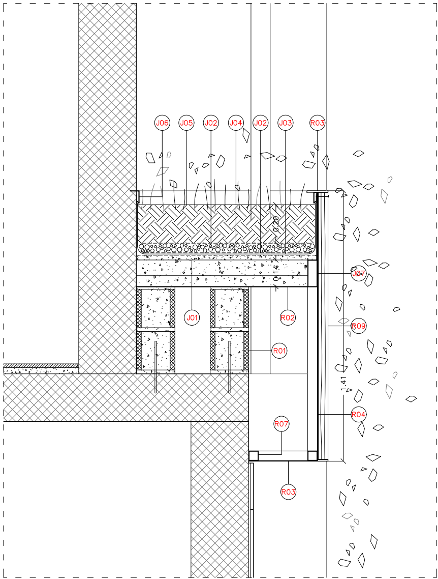
SECCIÓ H-H'
