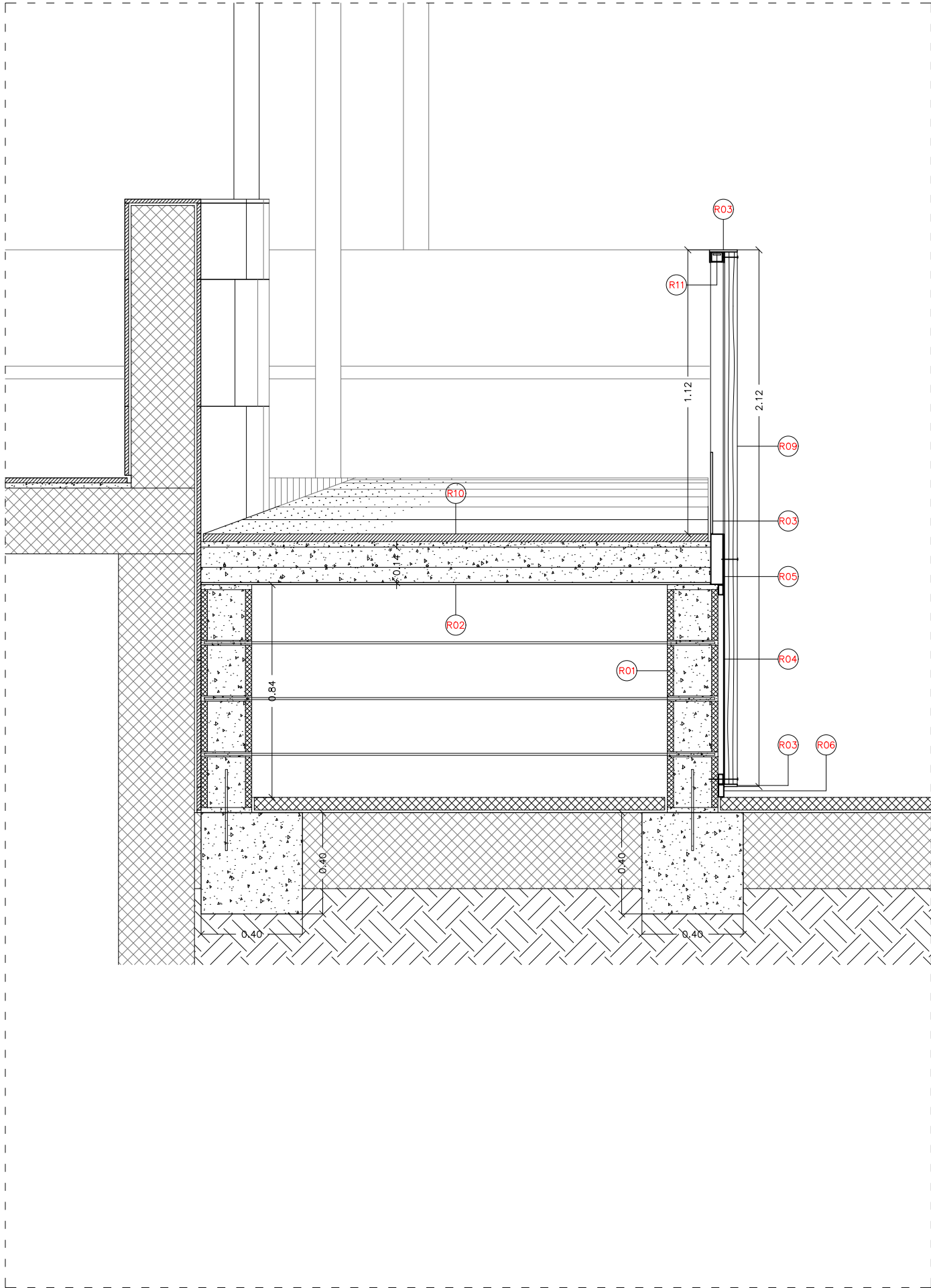
SECCIÓ E-E'
