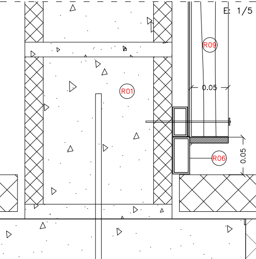
DETALL D04
