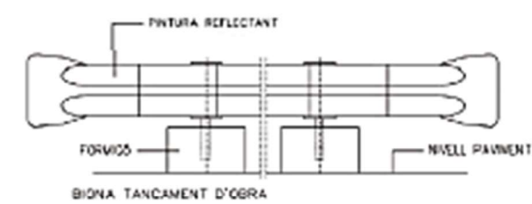
VISTA LATERAL
