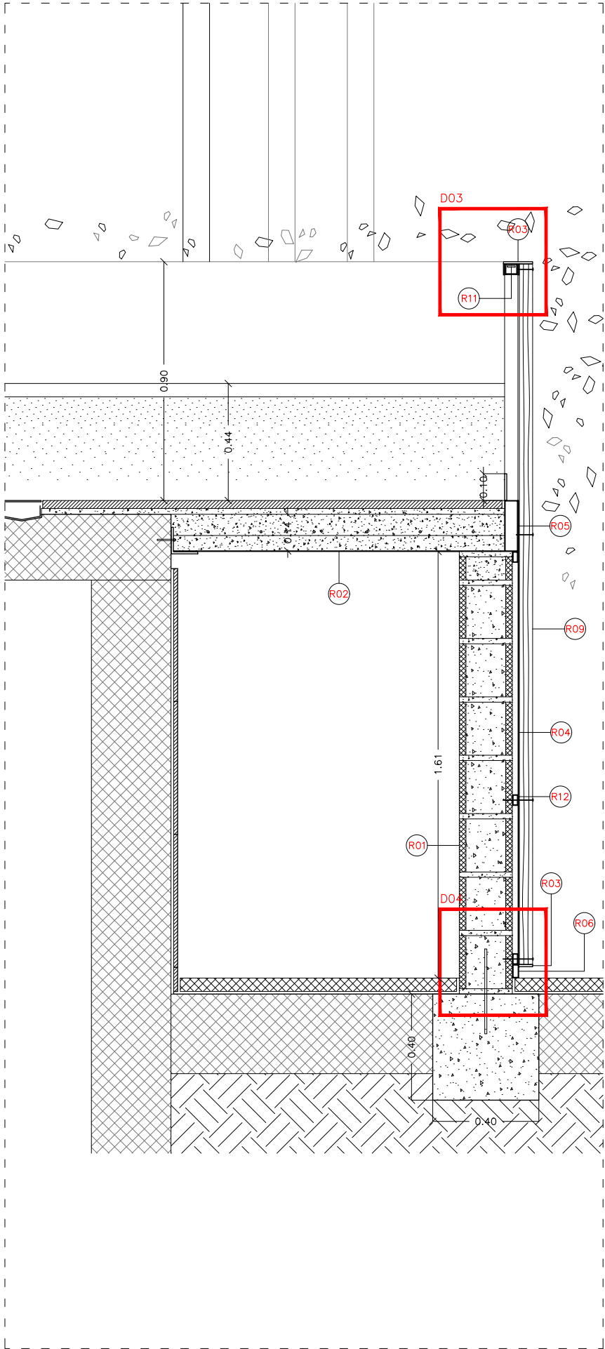
SECCIÓ F-F'
