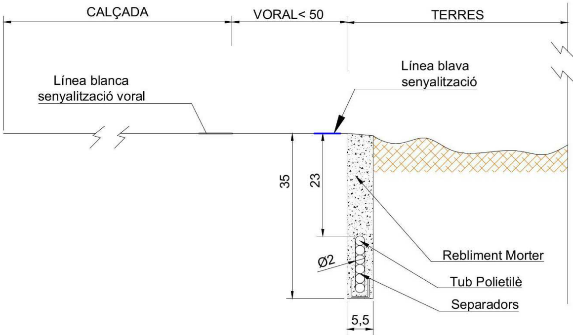
SECCIÓ TRANSVERSAL ST3a Secció constructiva de Micro-rasa en berma plana, al límit de la plataforma
