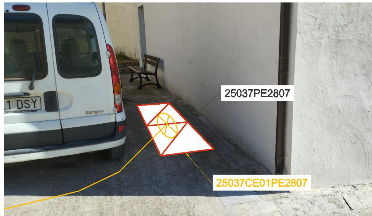
Fig 31. Instal·lació caixa d'empalmament 25037CE01PE2807.
