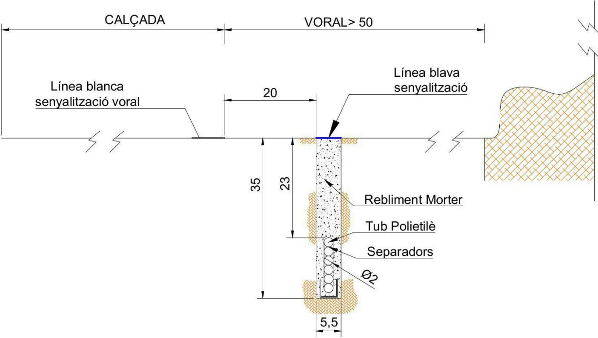
SECCIÓ TRANSVERSAL ST1 Secció constructiva de Micro-rasa sota voral superior a 50 centímetres
