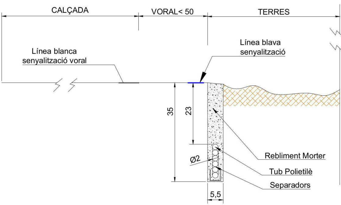
SECCIÓ TRANSVERSAL ST2a Secció constructiva de Micro-rasa en sota cuneta transitable de formigó existent
