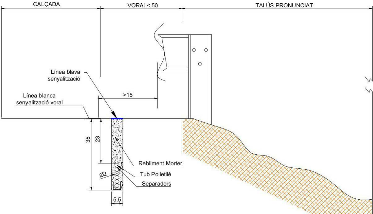
SECCIÓ TRANSVERSAL ST4 Secció constructiva de micro-rasa en zones amb voral molt estret, amb biona
