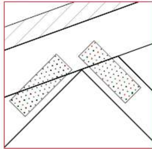
DETALL B E 1:10
