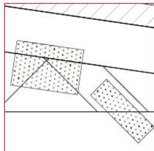
DETALL F E 1:10
