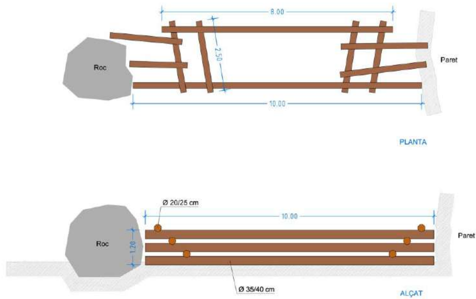
Imatge 2. Estructura de fusta d'elaboració pròpia per a la construcció d'un dic
