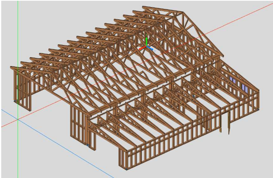
Imatge 7. Estructura 3d a Cadwork
