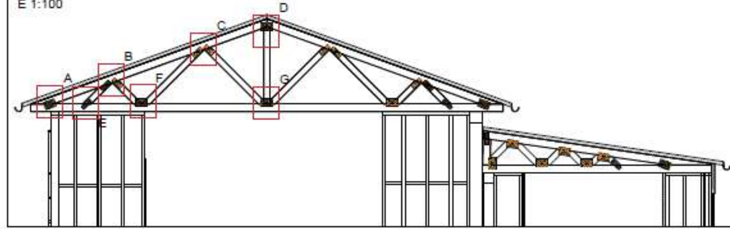
SECCIÓ CAVALLS E 1:100
