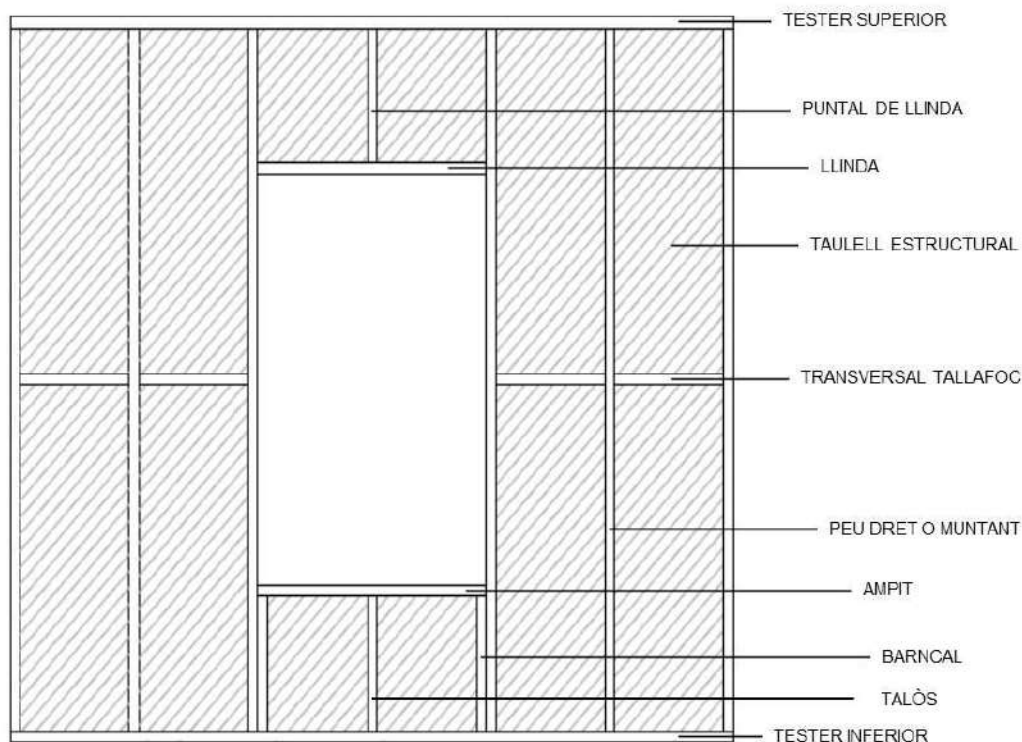
Fig 1. Esquema d'entramat lleuger
