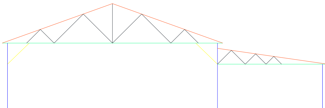
Imatge 4. Disseny de bàrfres 2d en cad
