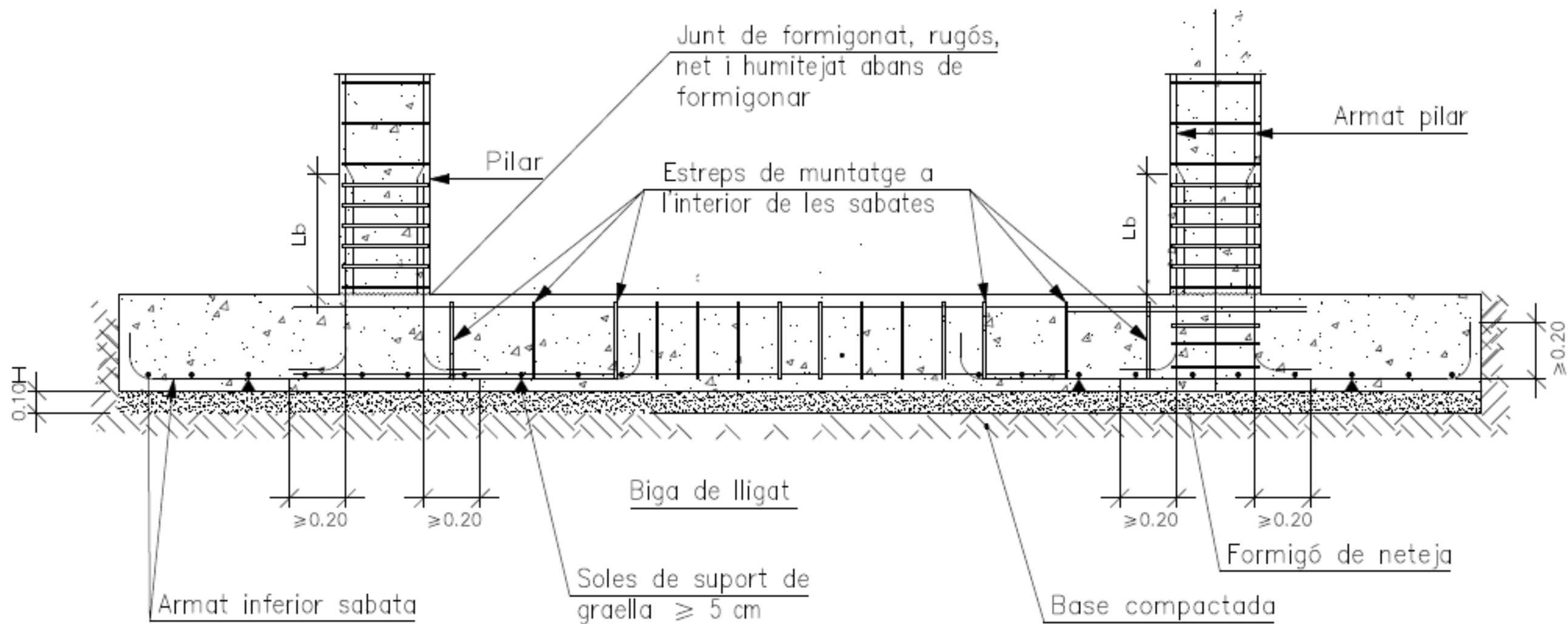
DETALL BIGA DE LLIGAT E 1:20
