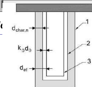
Figura E.1. Definició de la secció residual i efectiva.
