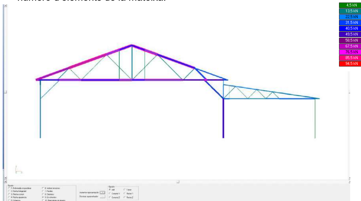
Imatge 9. Diagrama d'axils de l'estructura
