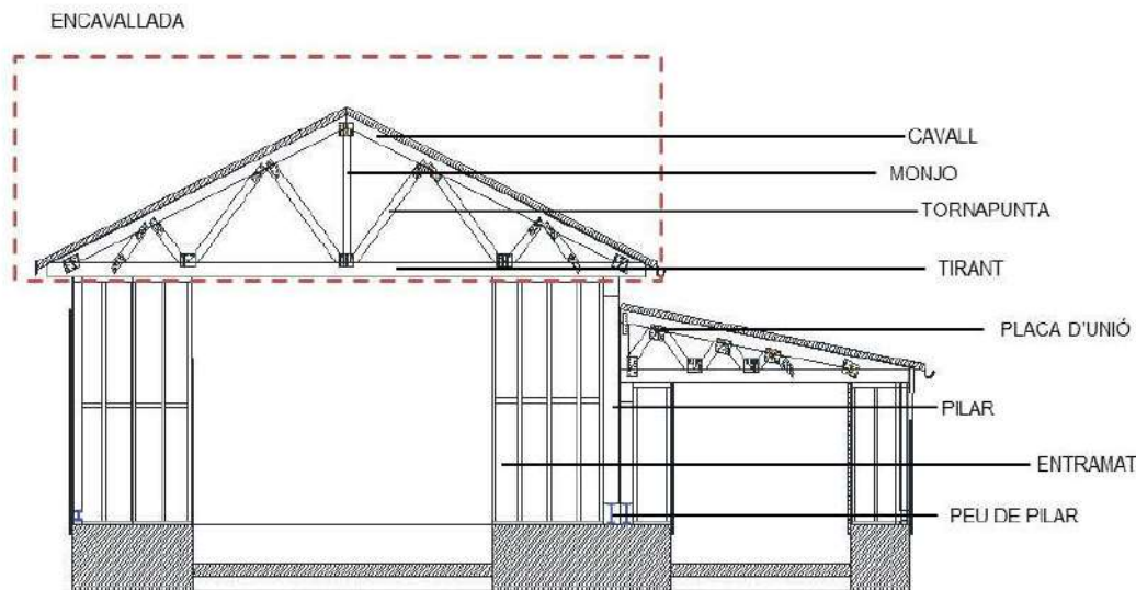
Fig 2. Estructura de fusta
