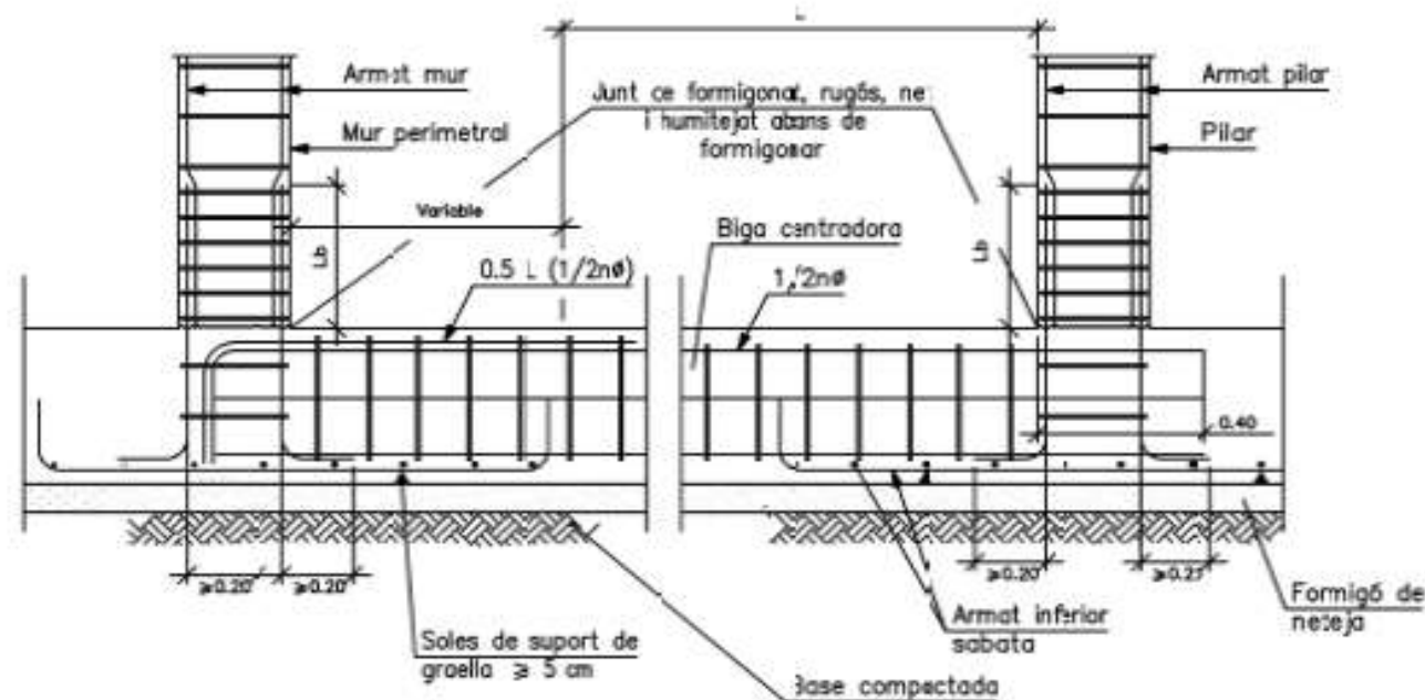
DETALL A BIGA CENTRADORA E 1:20
