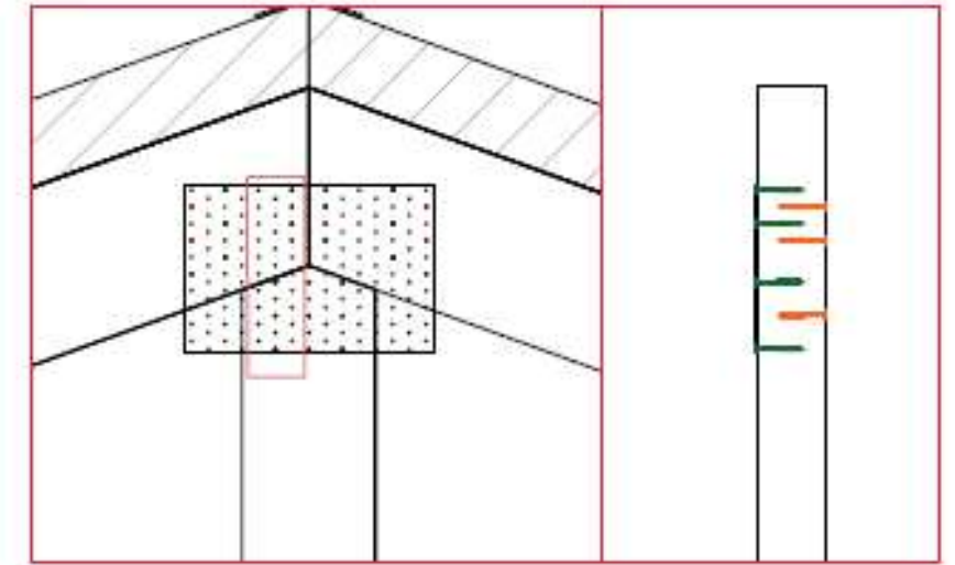
DETALL D E 1:10
