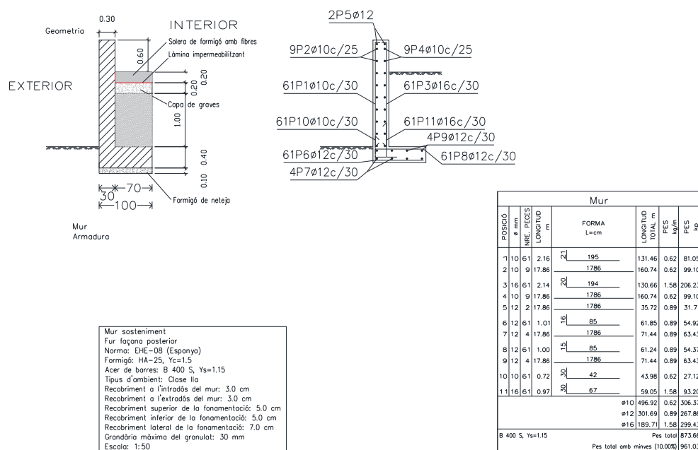
Imatge 10. Exportació en .dxf de CYPE del mur de la façana posterior
