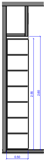
Armaris a mida Secció
