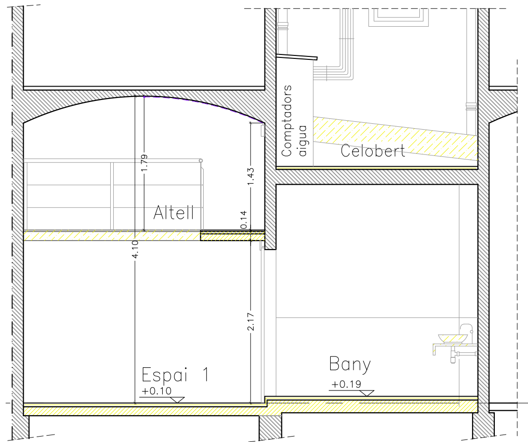
SECCIÓ TRANSVERSAL ST-1 ESTAT ACTUAL E: 1/50
