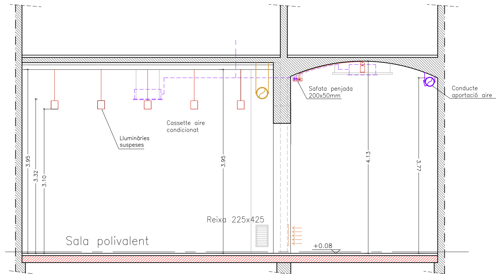
SECCIÓ TRANSVERSAL ST-2 INTERVENCIÓ E: 1/50
