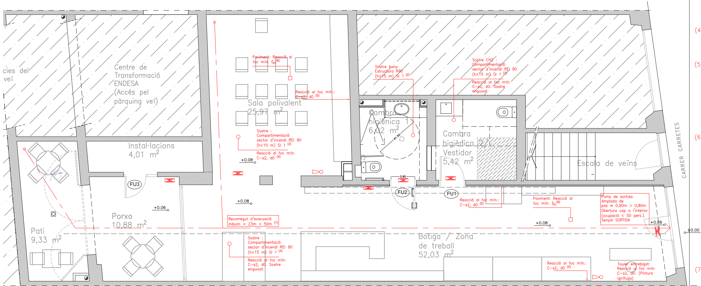
PLANTA BAIXA E: 1/75
