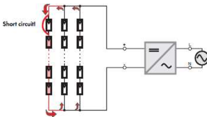
FALTA EN UNA DELS MÒDULS D'UNA DELS ESBRANQUES CONNECTADES EN PARAL·LEL
