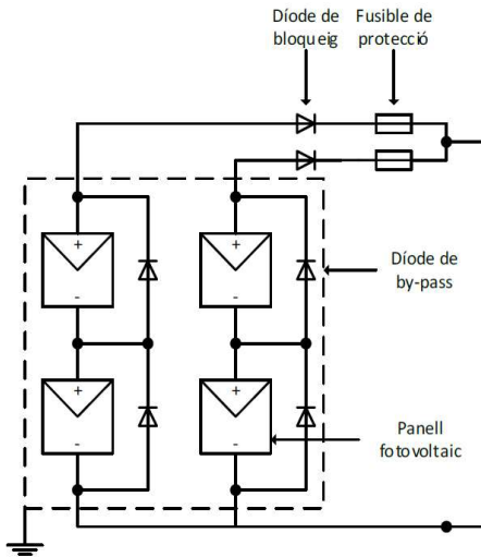
Circuit general de proteccions dels panells fotovoltaics
