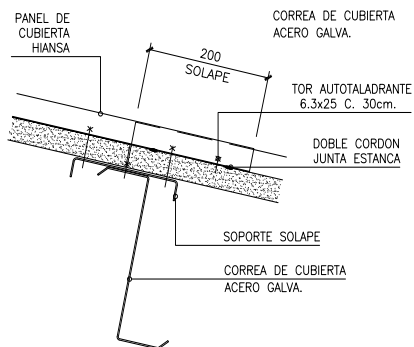
SECCIÓN SOLAPE
