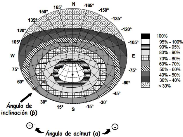
Figura 3.3 del CTE-HE 2007
