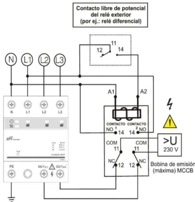
(Figura 1: Esquema de connexió del protector V-CHECK 4RPT amb relé de doble contacte per a actuació amb disparo extern)
