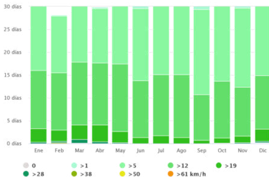
Gràfic 3: Frequència i Velocitat (km/h) del vent, per mes
