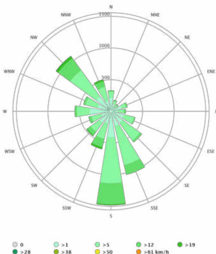
Gràfic 2: Vents dominants
