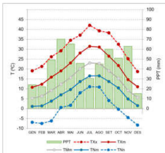
Gràfic 1: Normals climàtiques (període de referència 2007-2016)
