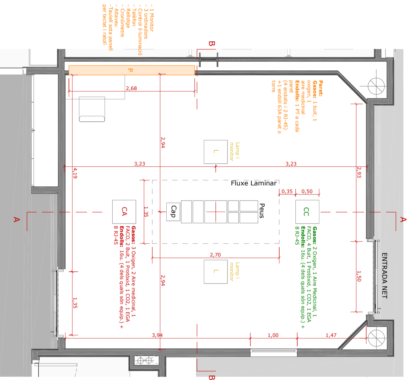
Planta quiròfan
