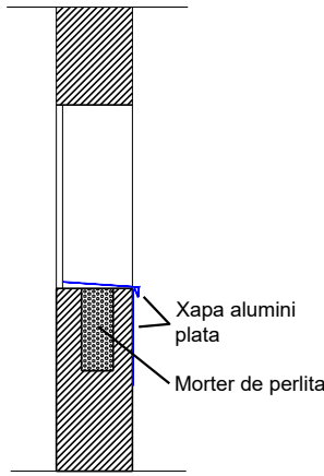
SECCIÓ ESTAT PROPOSTA
