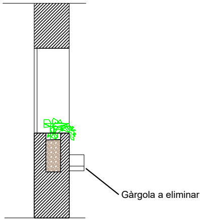
SECCIÓ ESTAT ACTUAL
