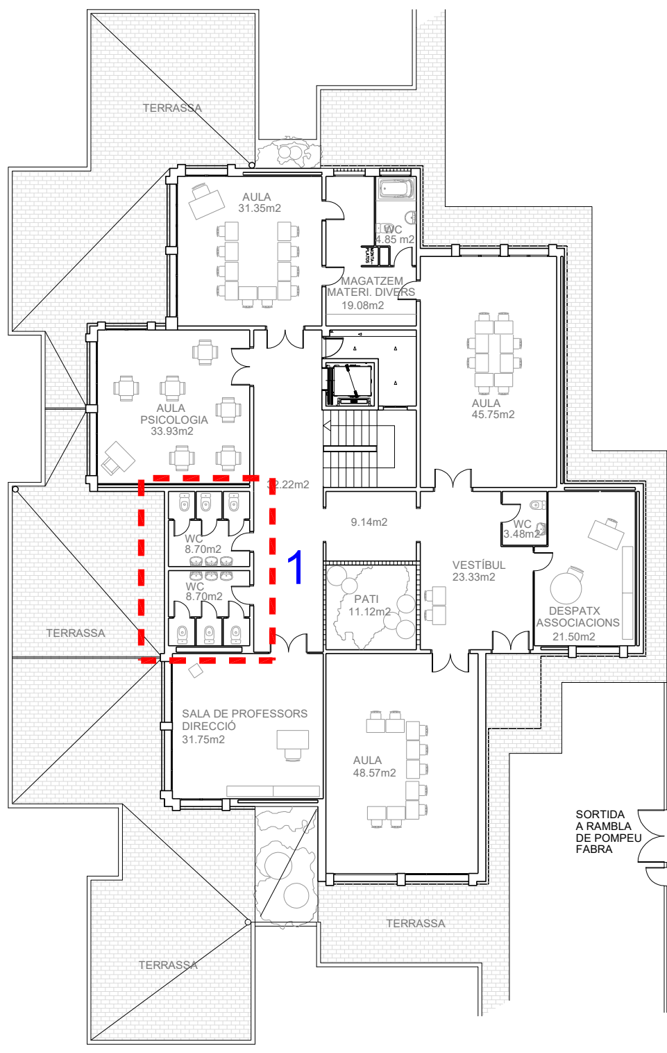
PLANTA PRIMERA
