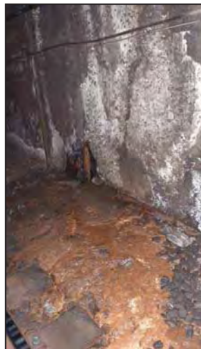
Foto 9: Filtració contravolta PK 105+975 v1.
