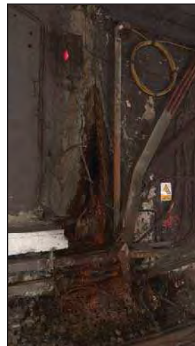
Foto 14: Filtració pantalla PK 106+215 v2.
