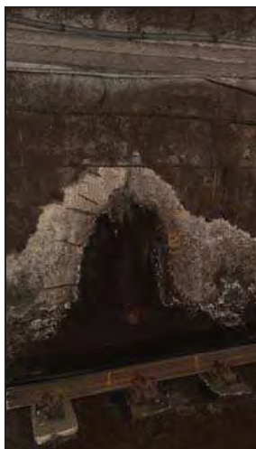
Foto 15: Filtració pant.- cvolta PK 106+330 v2.
