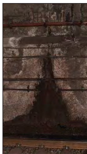
Foto 24: Filtració pantalla PK 106+880 v2.
