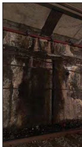
Foto 6: Filtració pantalla-volta PK 105+750 v2.
