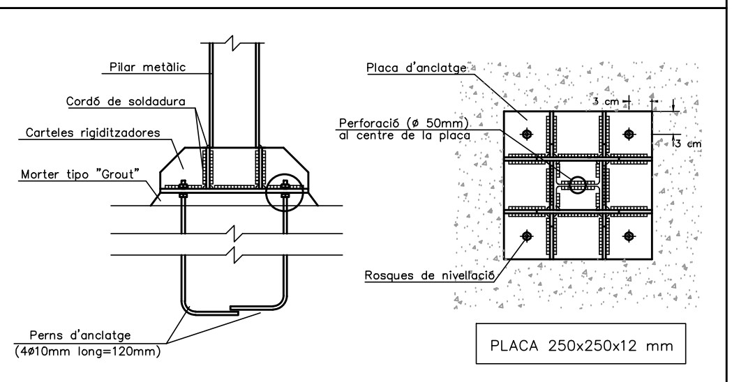
DETALL ANCLATGE DE PILAR METÀL·LIC AMB CARTEL·LES
