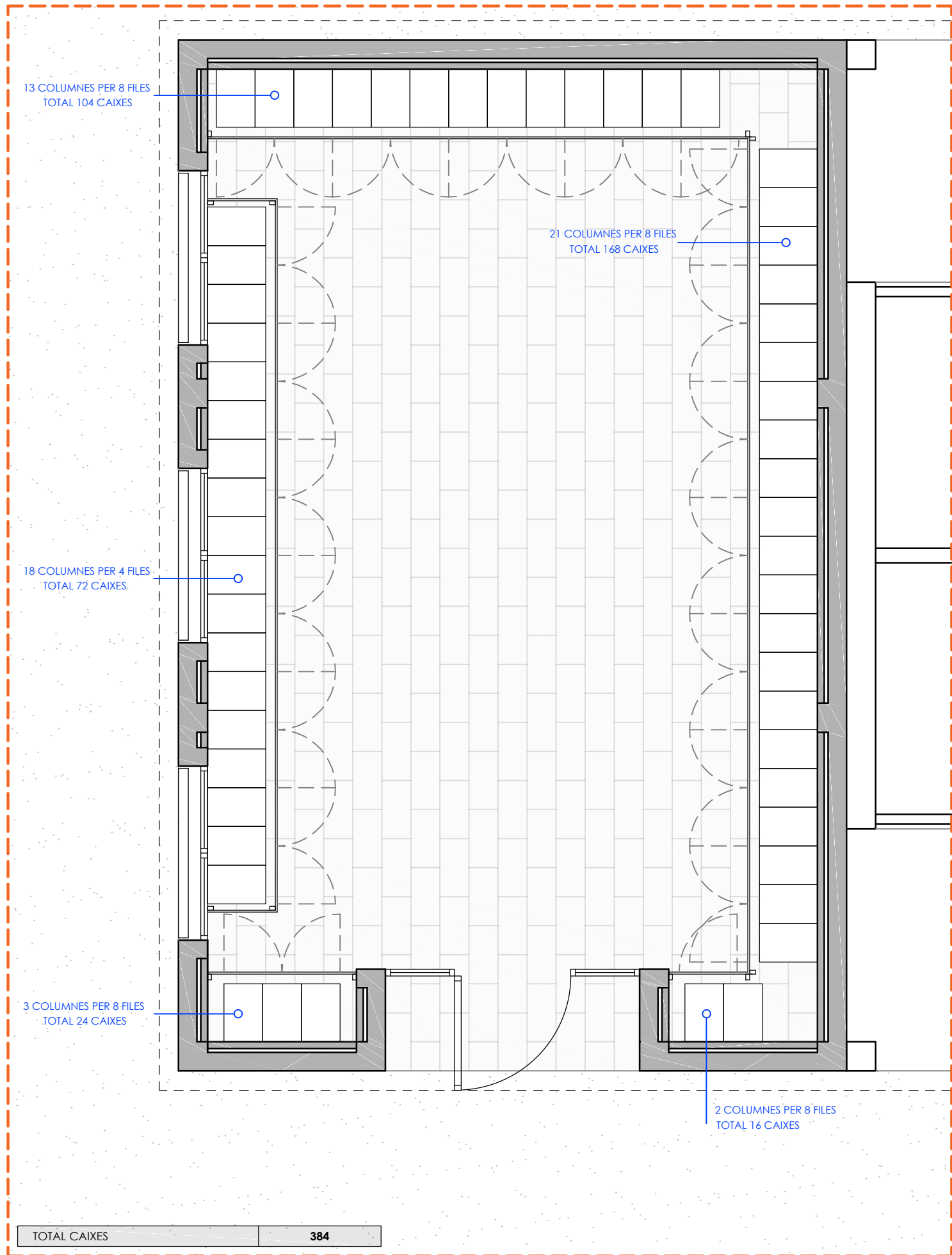
PLANTA DISTRIBUCIÓ
