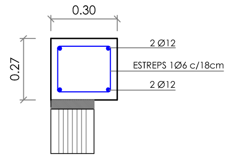
CÈRCOL SOBRE MUR C-1 30x27
