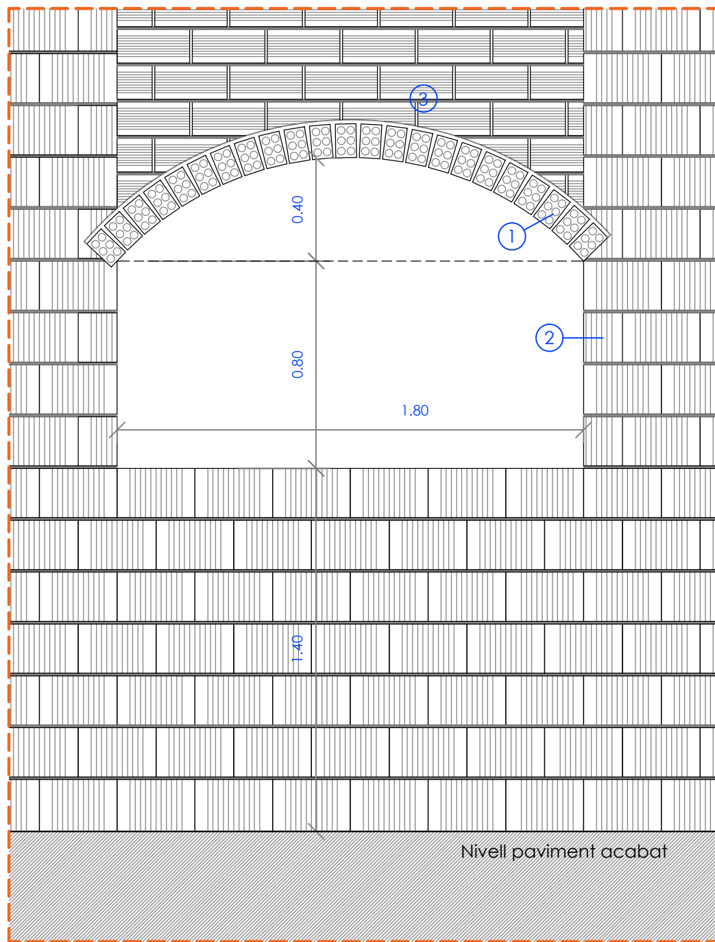
DETALL CONSTRUCTIU DELS ARCS 01
