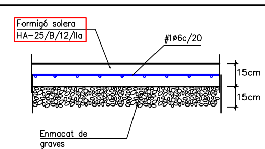
DETALL SOLERA DE FONAMENTACIÓ
