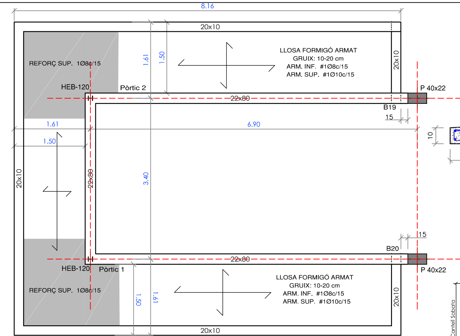
PLANTA INTERMITJA - VOLADIU
