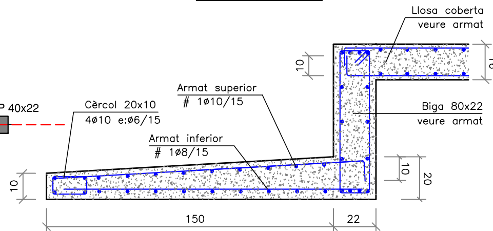
DETALL VOLADIU
