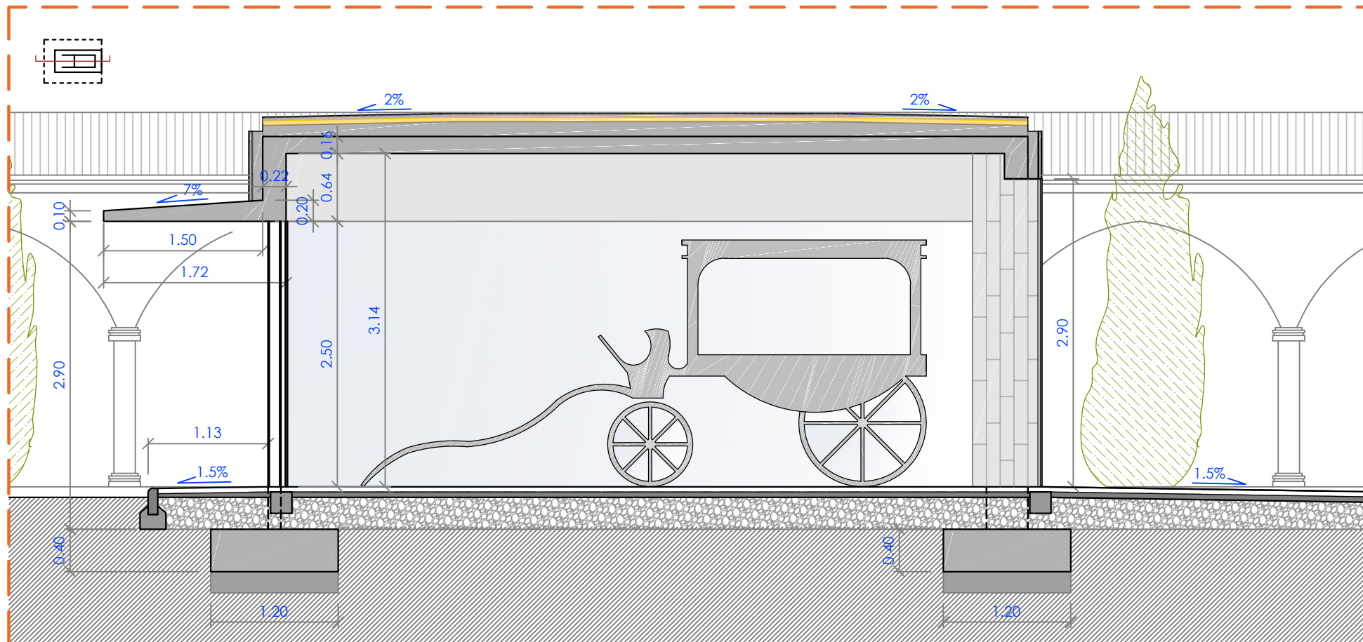
SECCIÓ AA'
