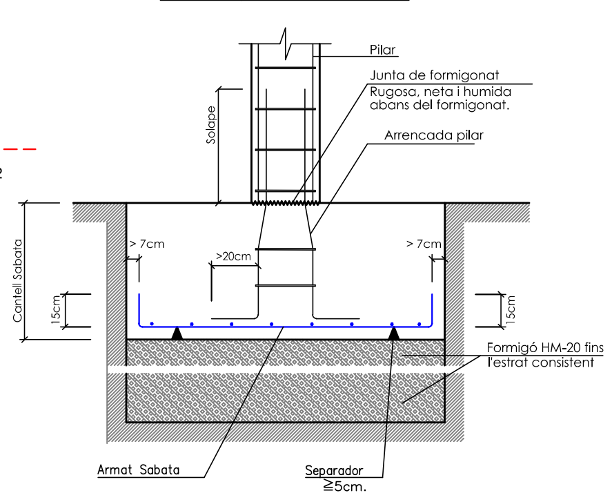
DETALL SABATA AILLADA
