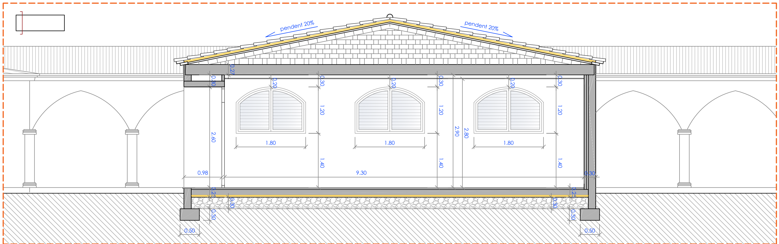
SECCIÓ AA'
