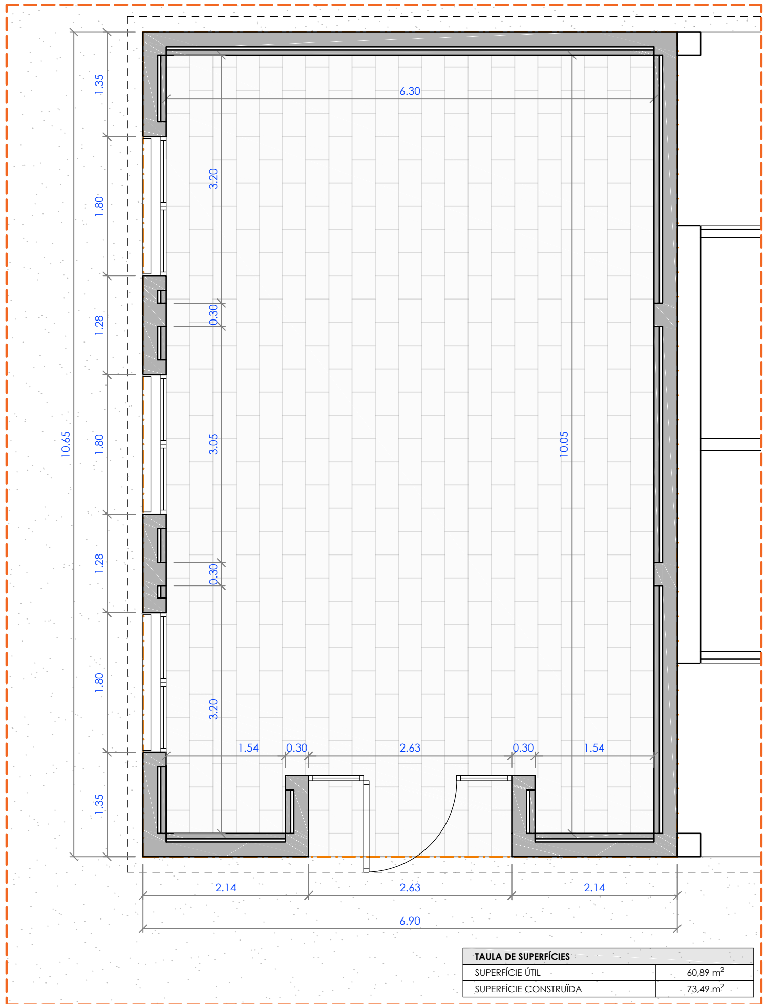
PLANTA COTES
