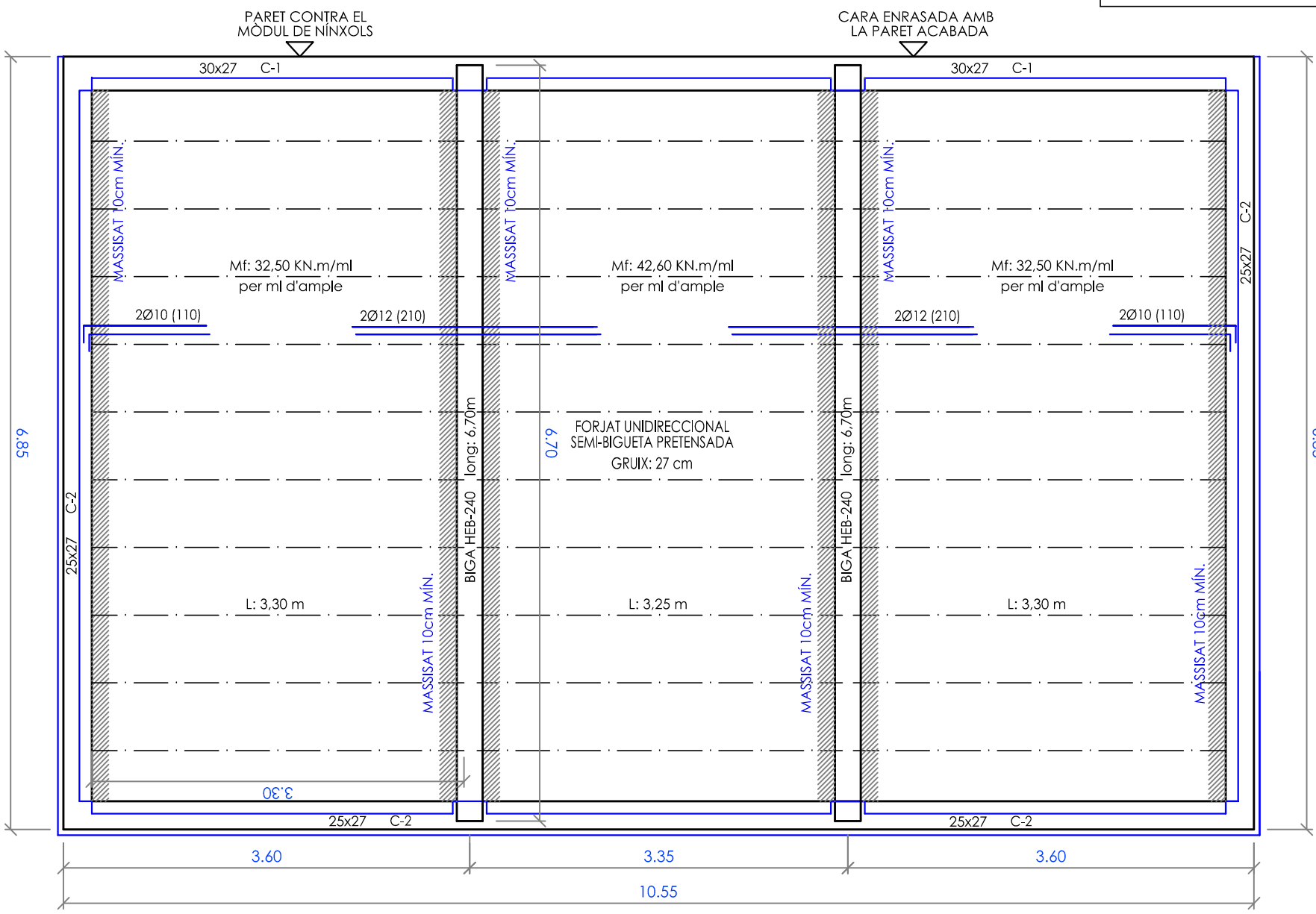
PLANTA - FORJAT
