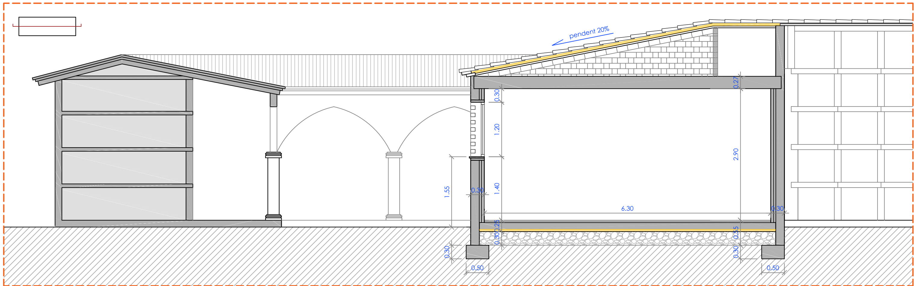
SECCIÓ BB'
