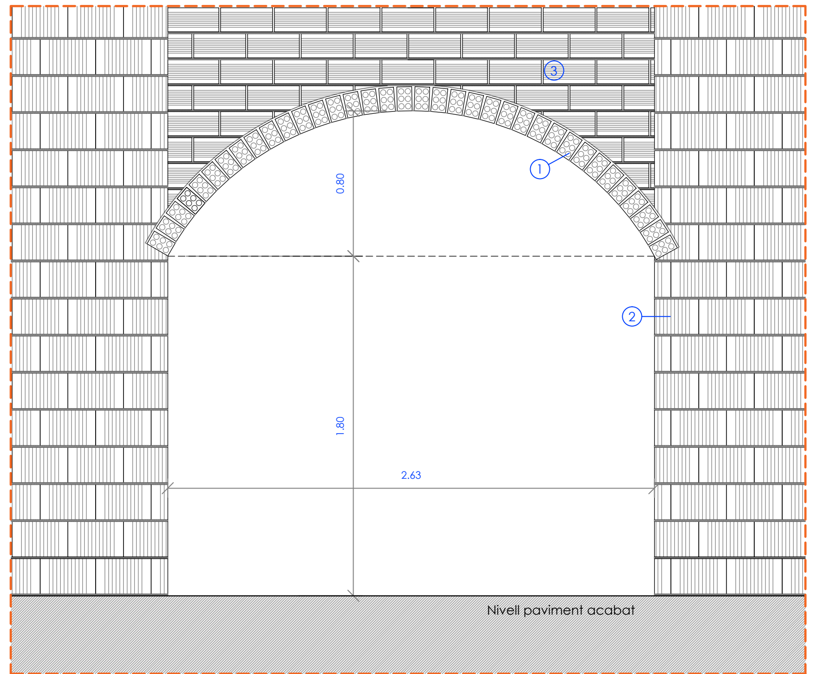
DETALL CONSTRUCTIU DE L'ARC 02
