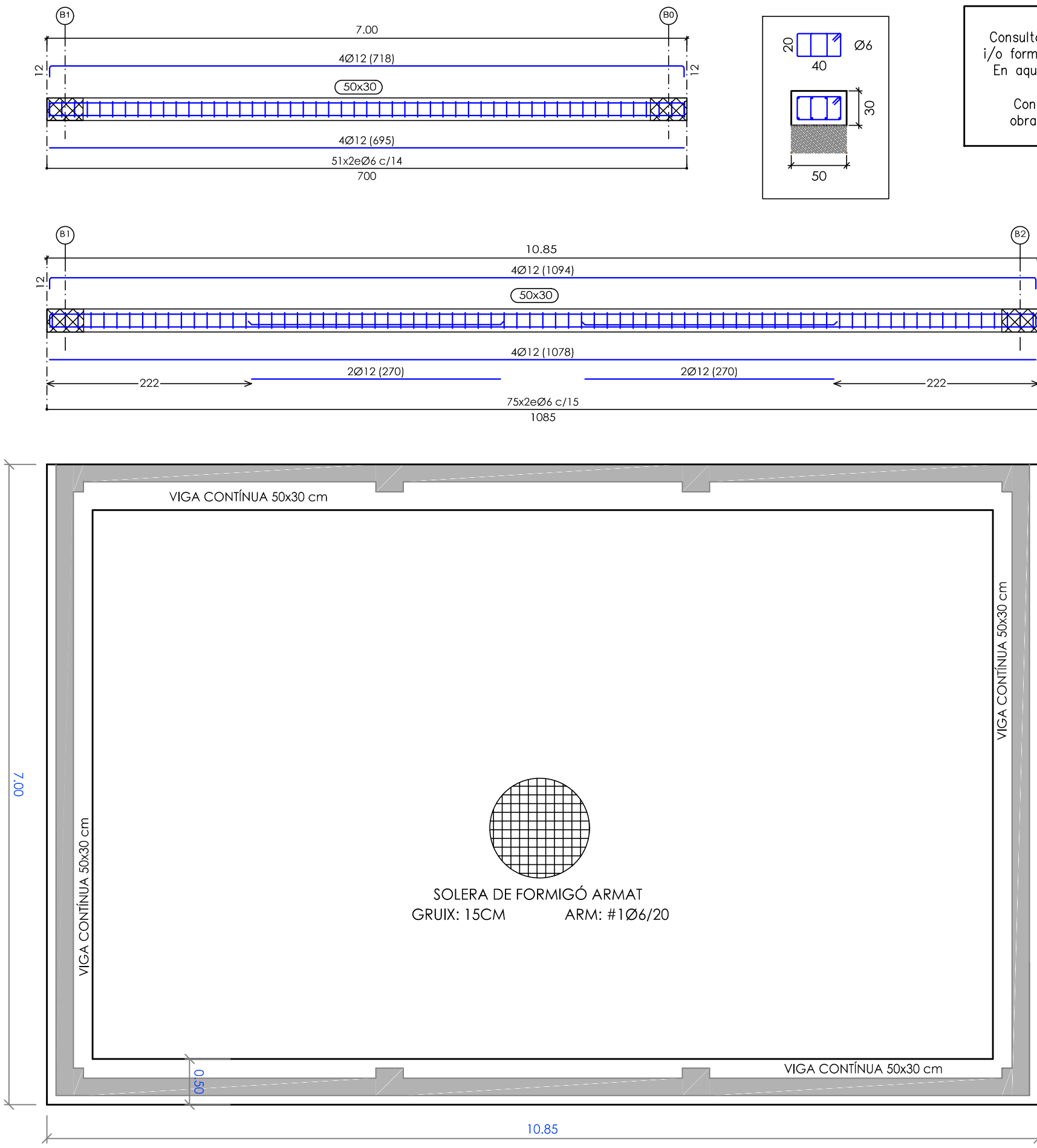
PLANTA - FONAMENTS
