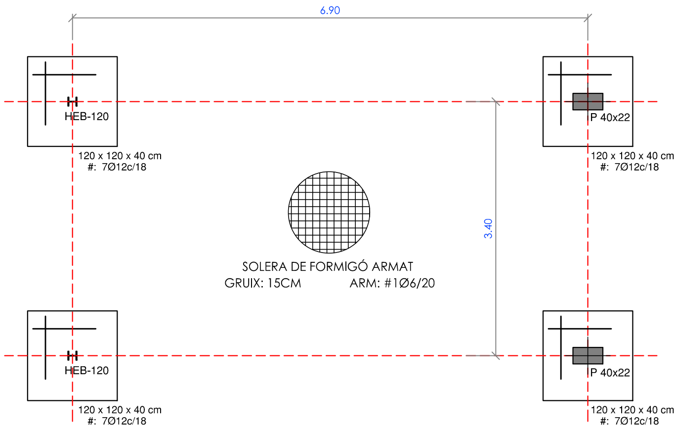
PLANTA - FONAMENTS
