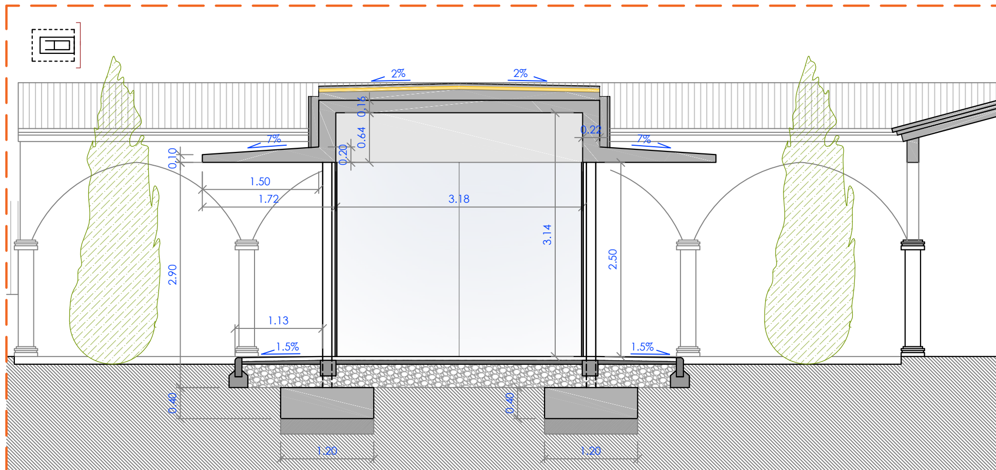
SECCIÓ BB'
