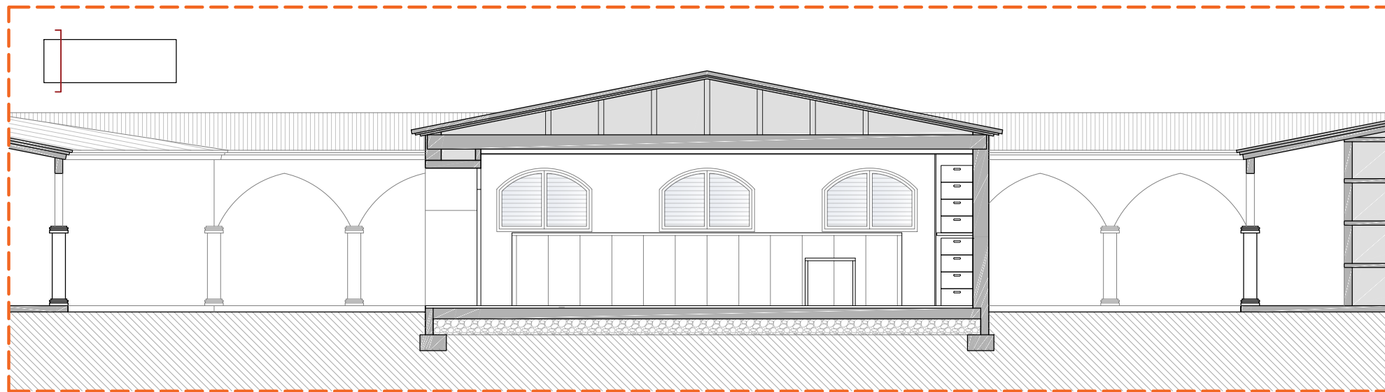
SECCIÓ AA'
