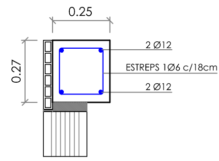
CÈRCOL SOBRE MUR C-2 25x27
