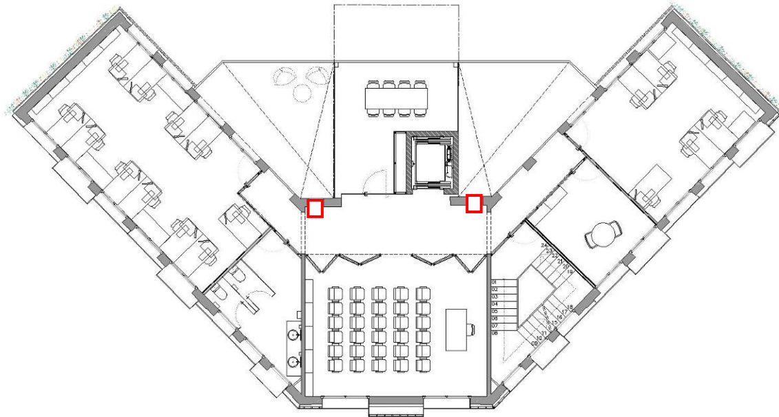
Planta primera. Situació contenidors emmagatzematge immediat
