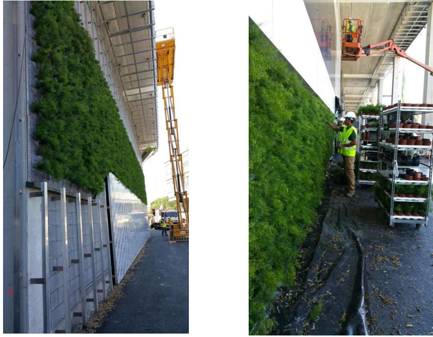
Sistemes d'elevació 2. Instal·lació de sistemes de panells amb vegetació directament sobre rastrells.
