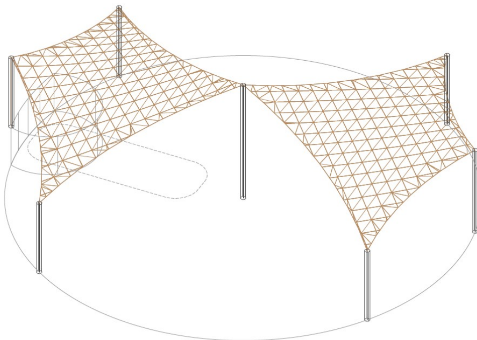
Simulació aproximada geometria tendals
