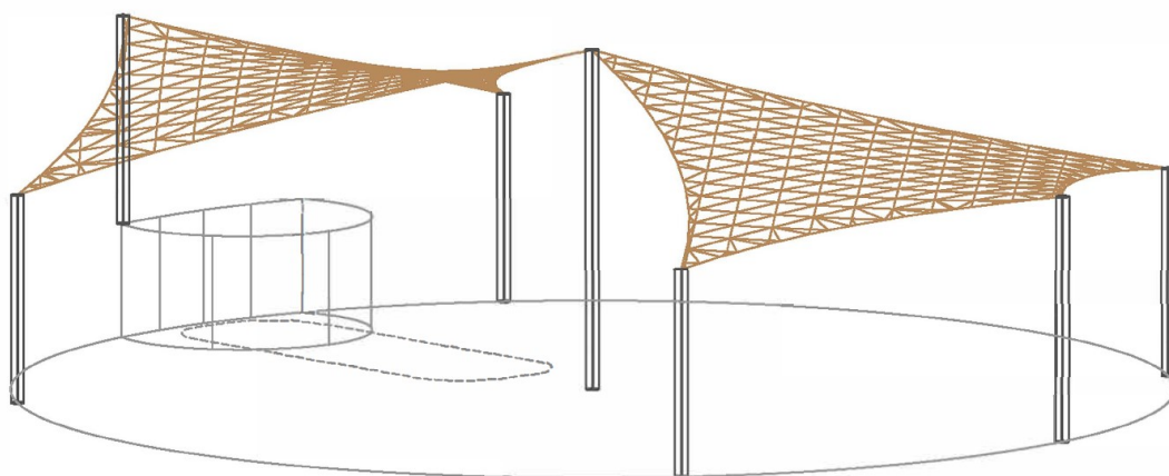
Simulació aproximada geometria tendals
