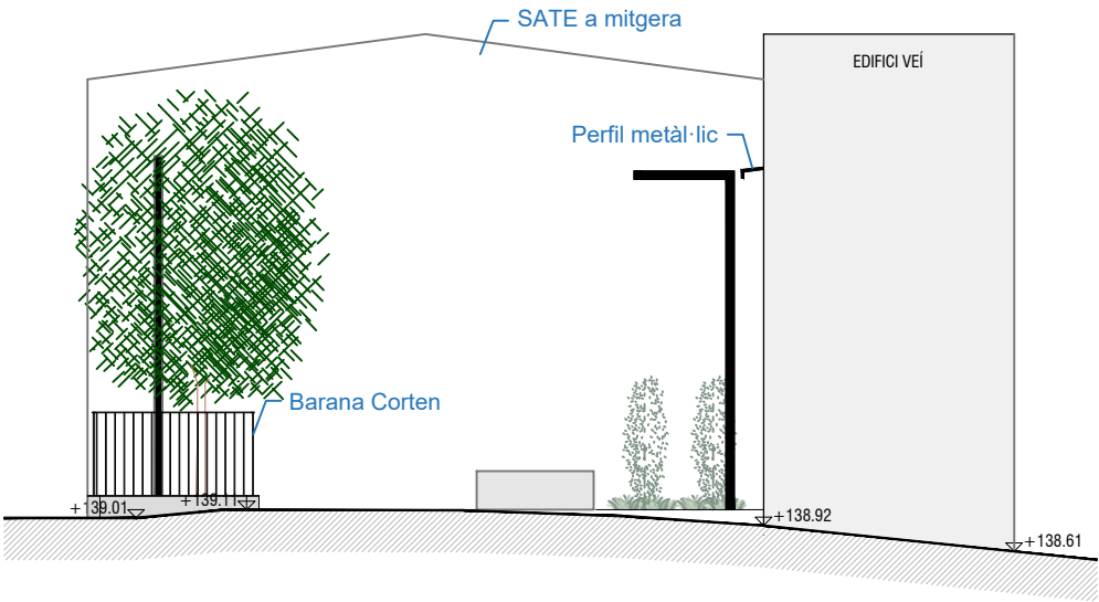
ALÇAT CARRER SANT FELIP NERI
