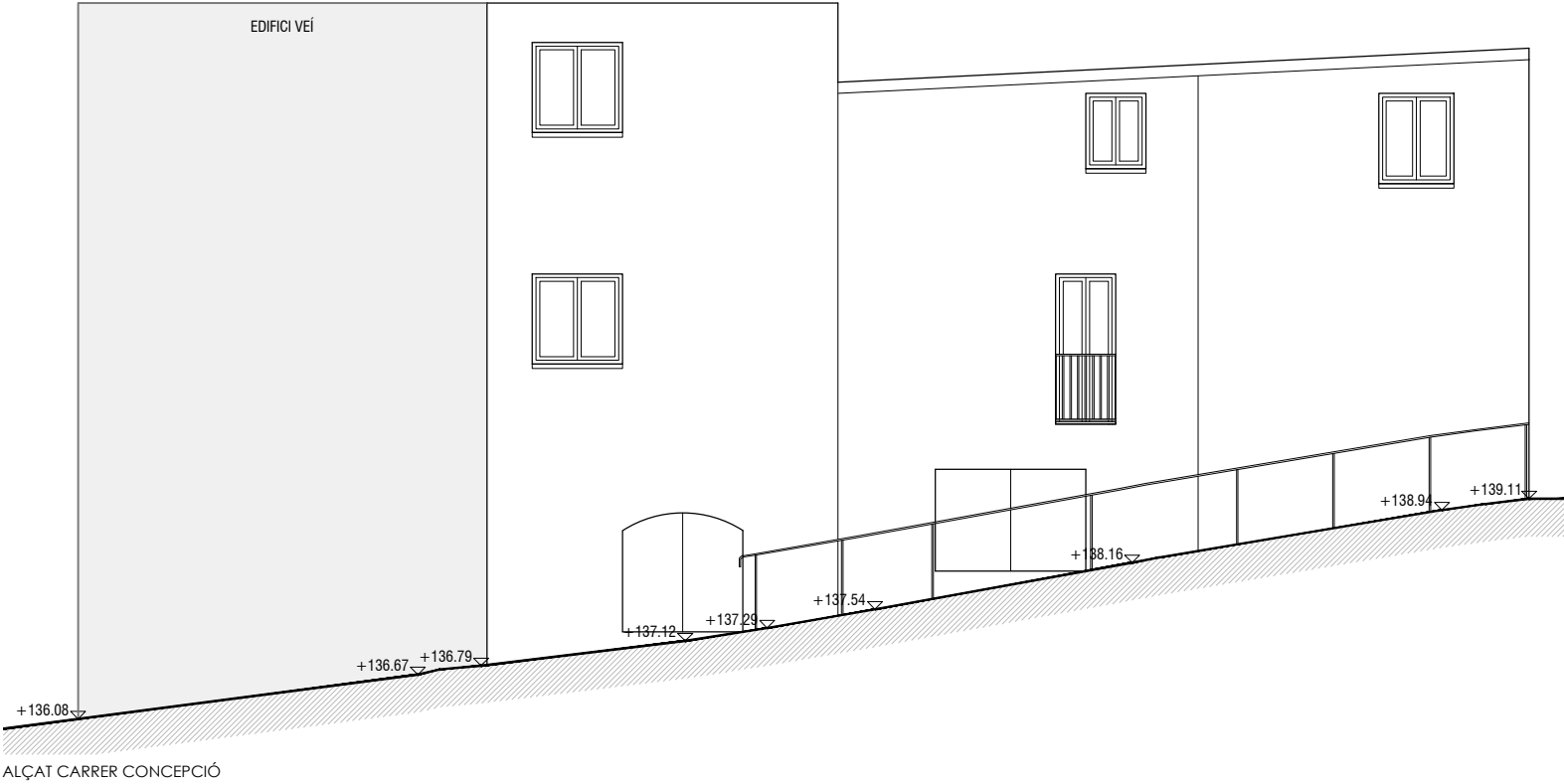
ALÇAT CARRER CONCEPCIÓ
