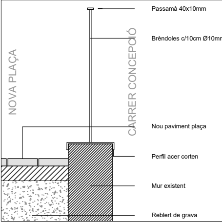
DETALL CONSTRUCTIU E 1/25
