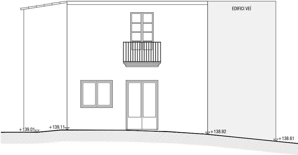
ALÇAT CARRER SANT FELIP NERI
