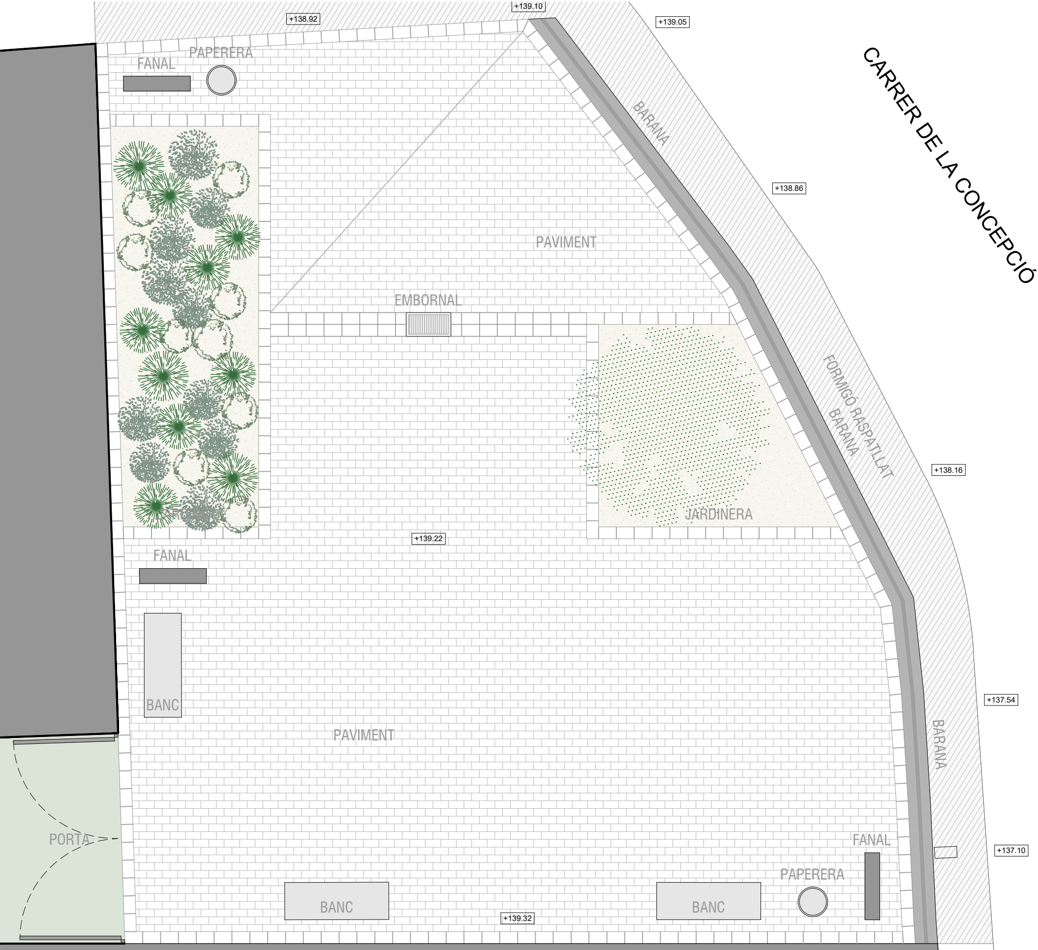
PROPOSTA | PLANTA DETALL
