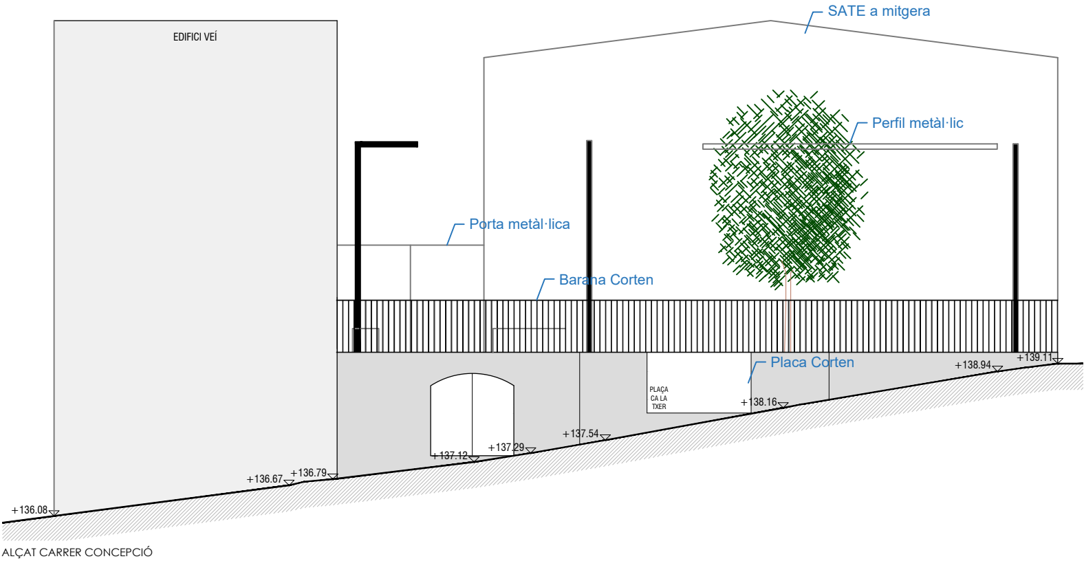
ALÇAT CARRER CONCEPCIÓ
