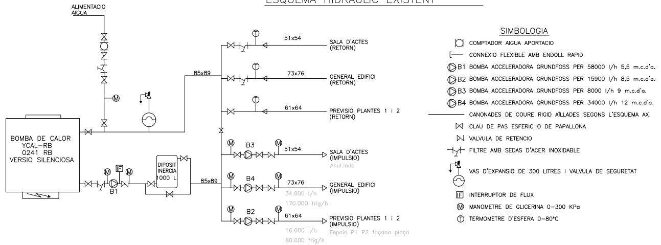
ESQUEMA HIDRAULIC EXISTENT
