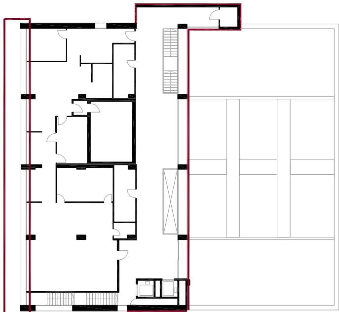
PLANTA SEGONA. ESCALA 1/400
