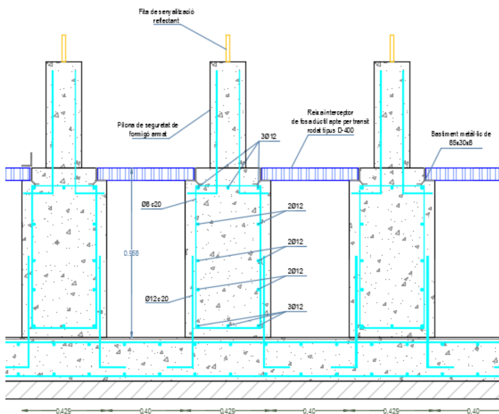
Esquema estructural llosa i canals.
