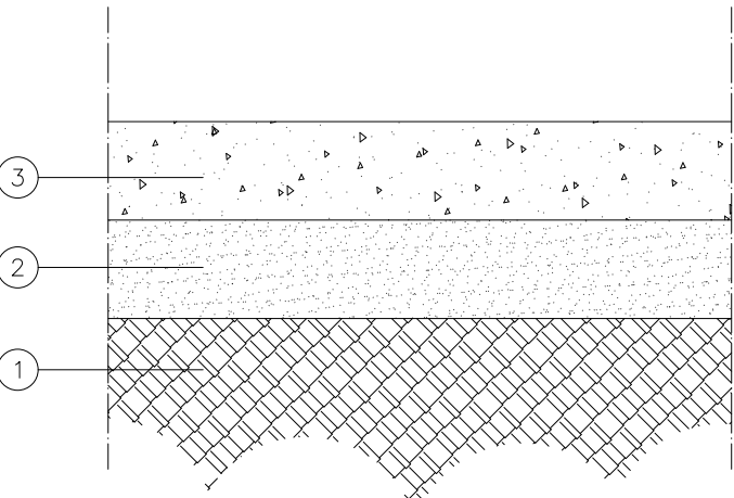
Detall paviment
