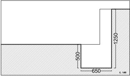
rasa tipo 2
