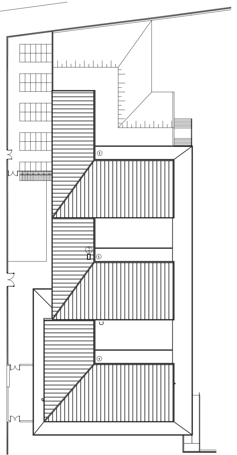
PLANTA COBERTA
