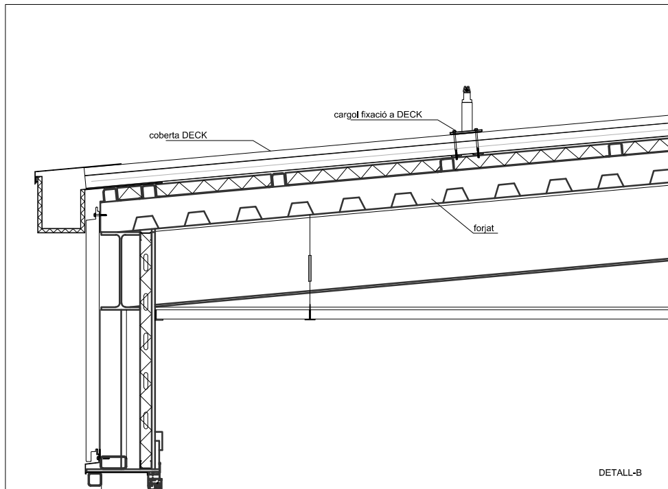
DETALL-A
