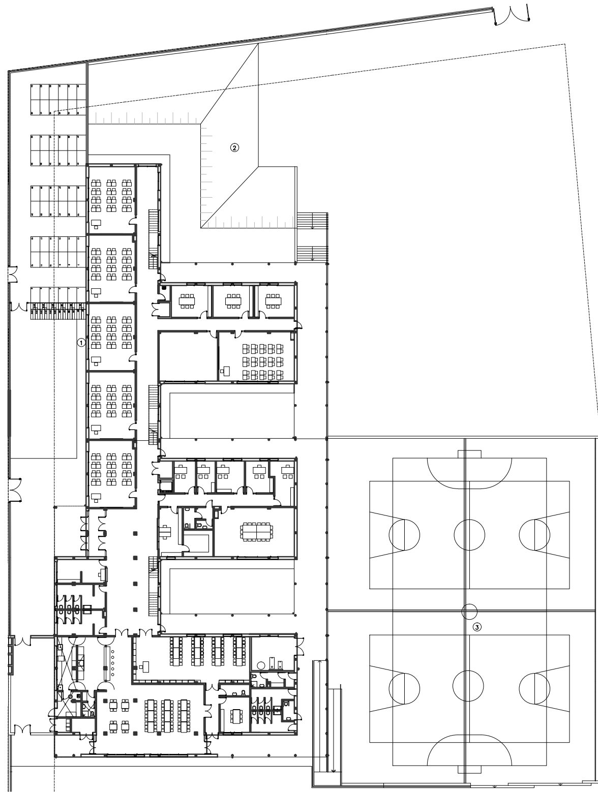
PLANTA BAIXA
