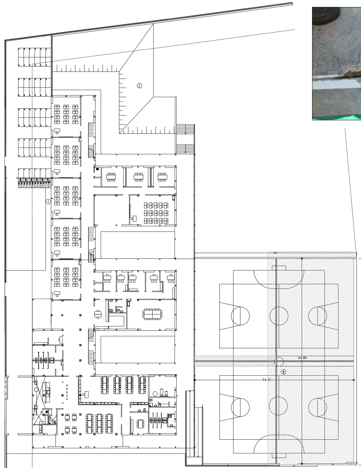
PLANTA BAIXA
