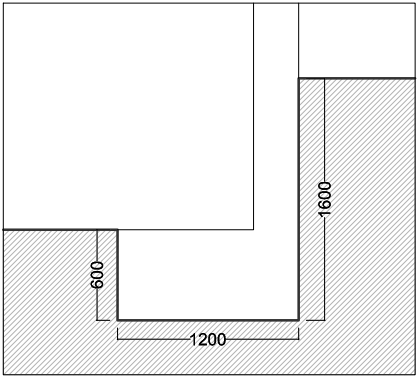
rasa tipo 1
