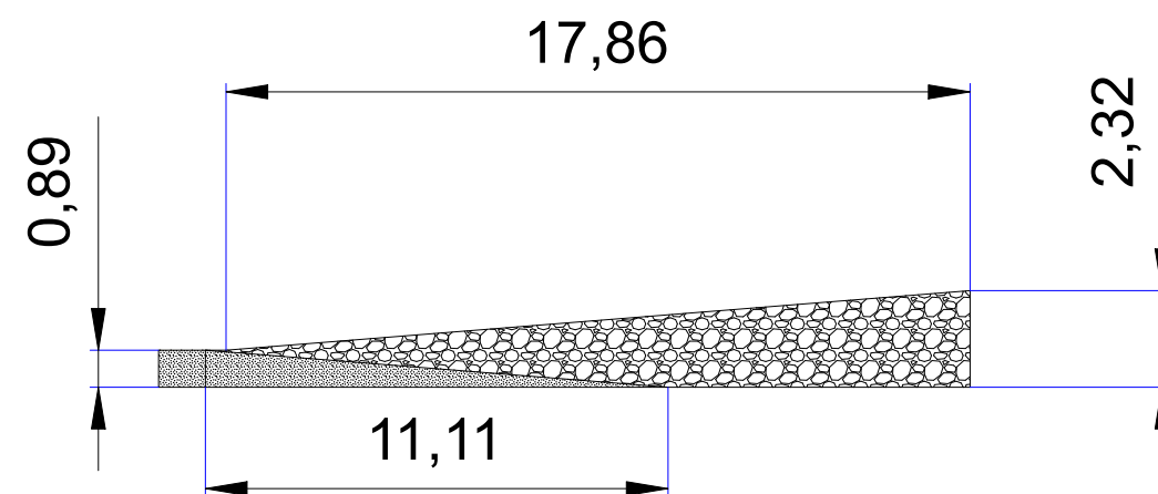
SECCIÓ A-A'
