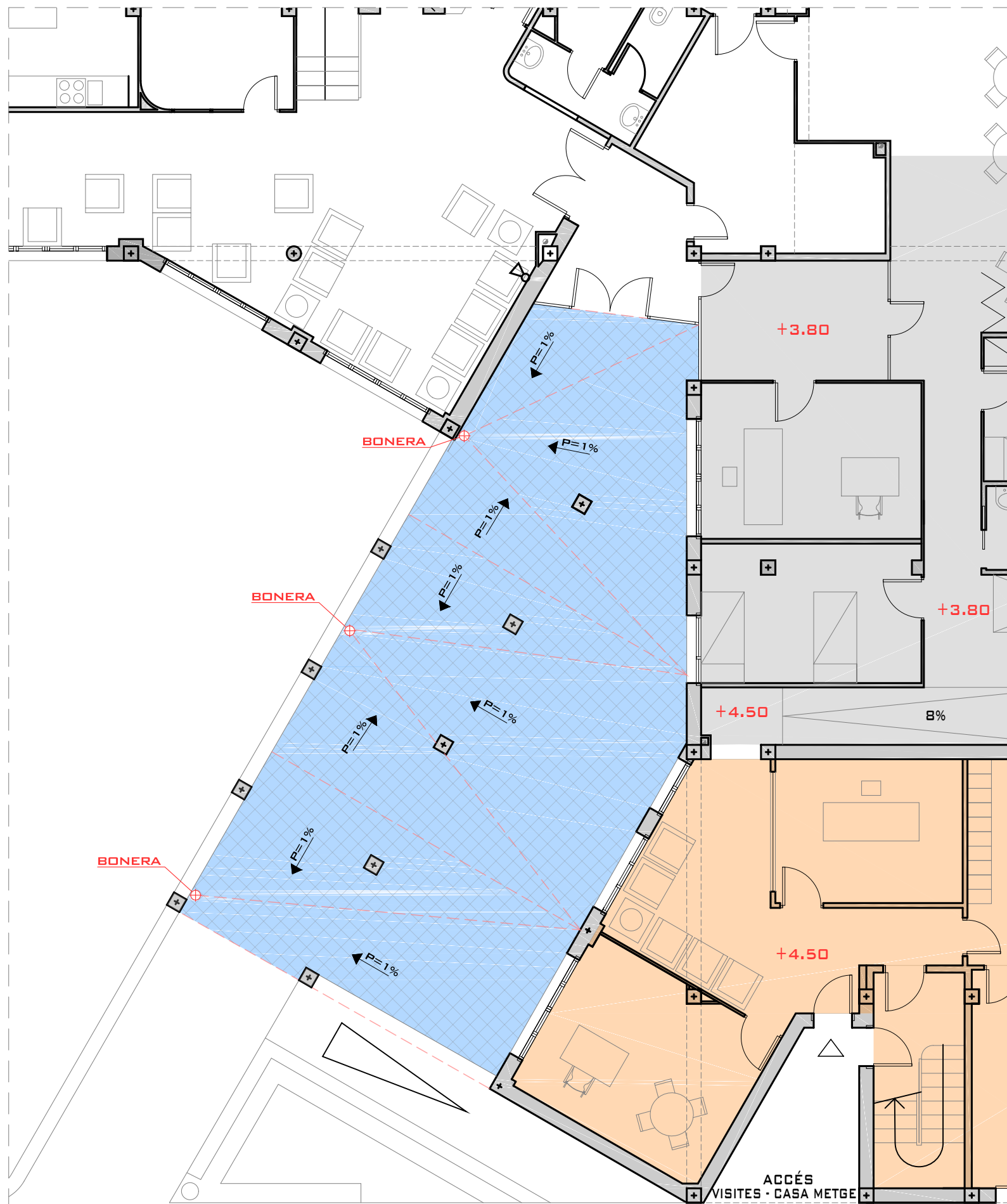
CARRER DE LA FONT ESTAT PROPOSTA - P.PRIMERA/COBERTA - REPARACIÓ DE COBERTA PLANA
