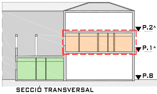
SECCIÓ TRANSVERSAL
