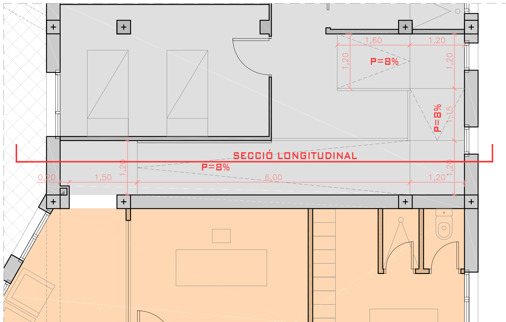
ESTAT PROPOSTA - RAMPA ACCESSIBLE - PLANTA PRIMERA (E:1/50)
