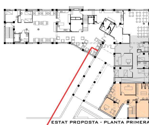
ESTAT PROPOSTA - PLANTA PRIMERA
