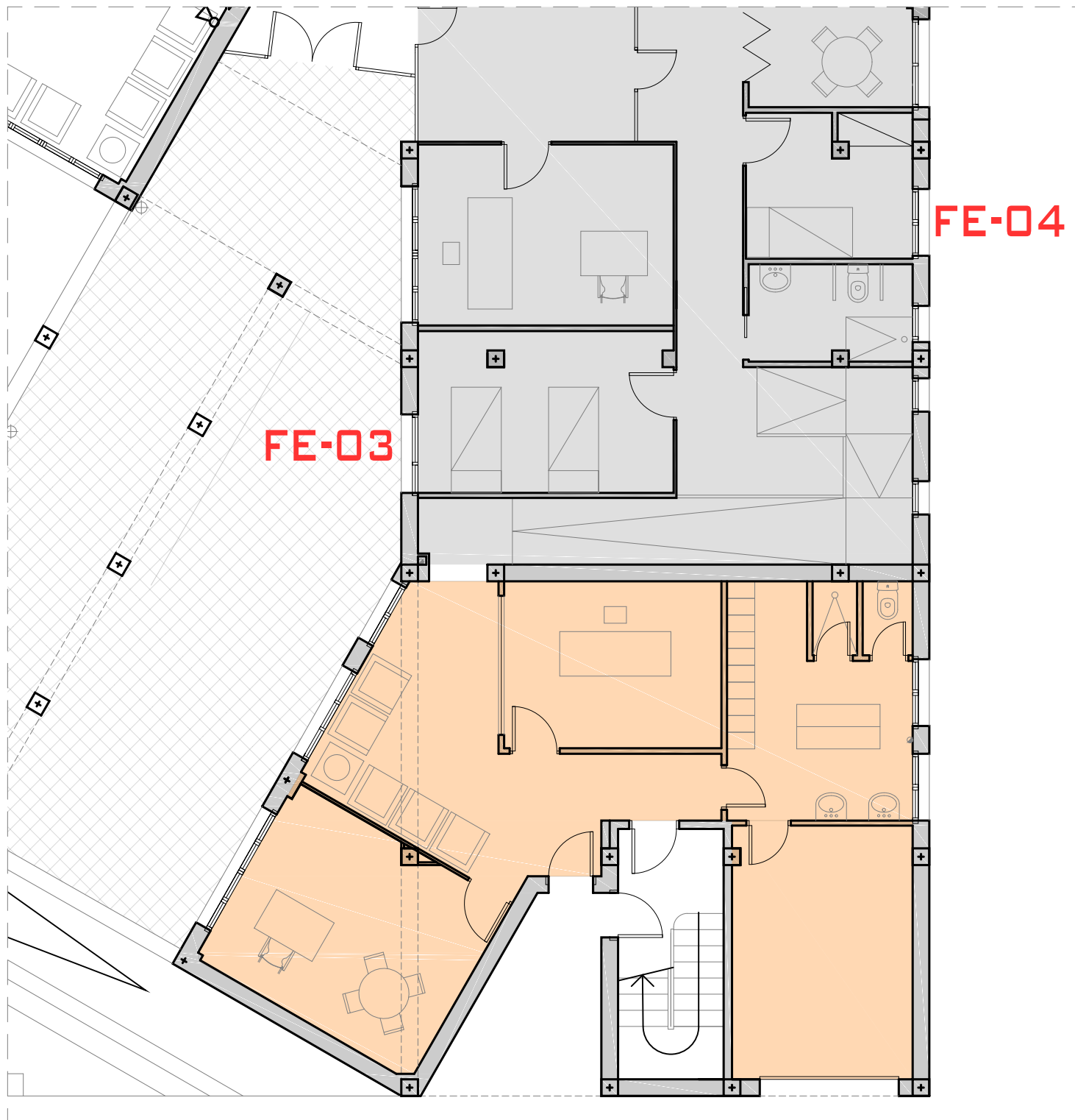
FUSTERIES EXTERIORS - ESTAT PROPOST - PLANTA PRIMERA
