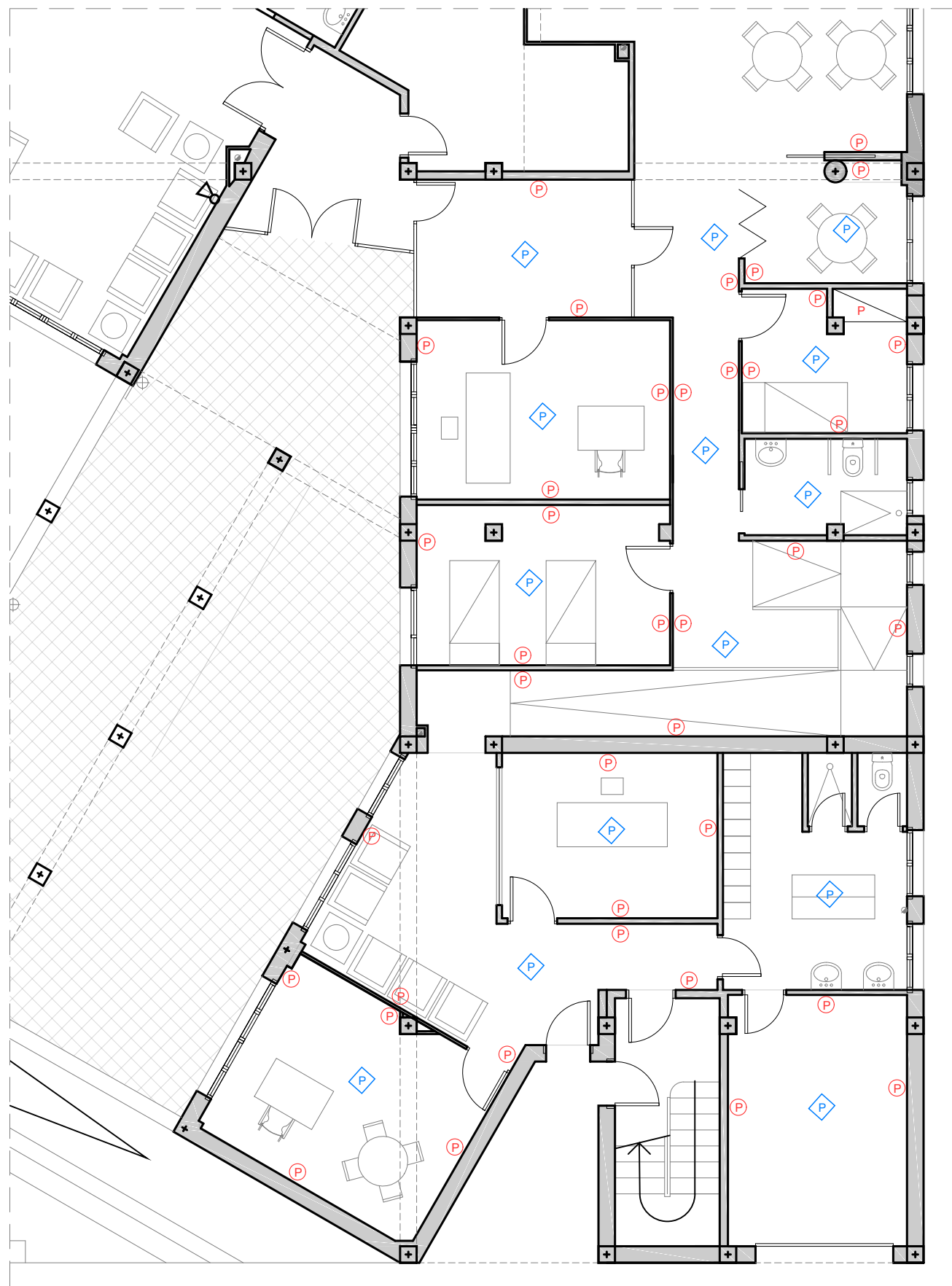
ESTAT PROPOSTA - REVESTIMENT DE PARETS I SOSTRES - P.PRIMERA
