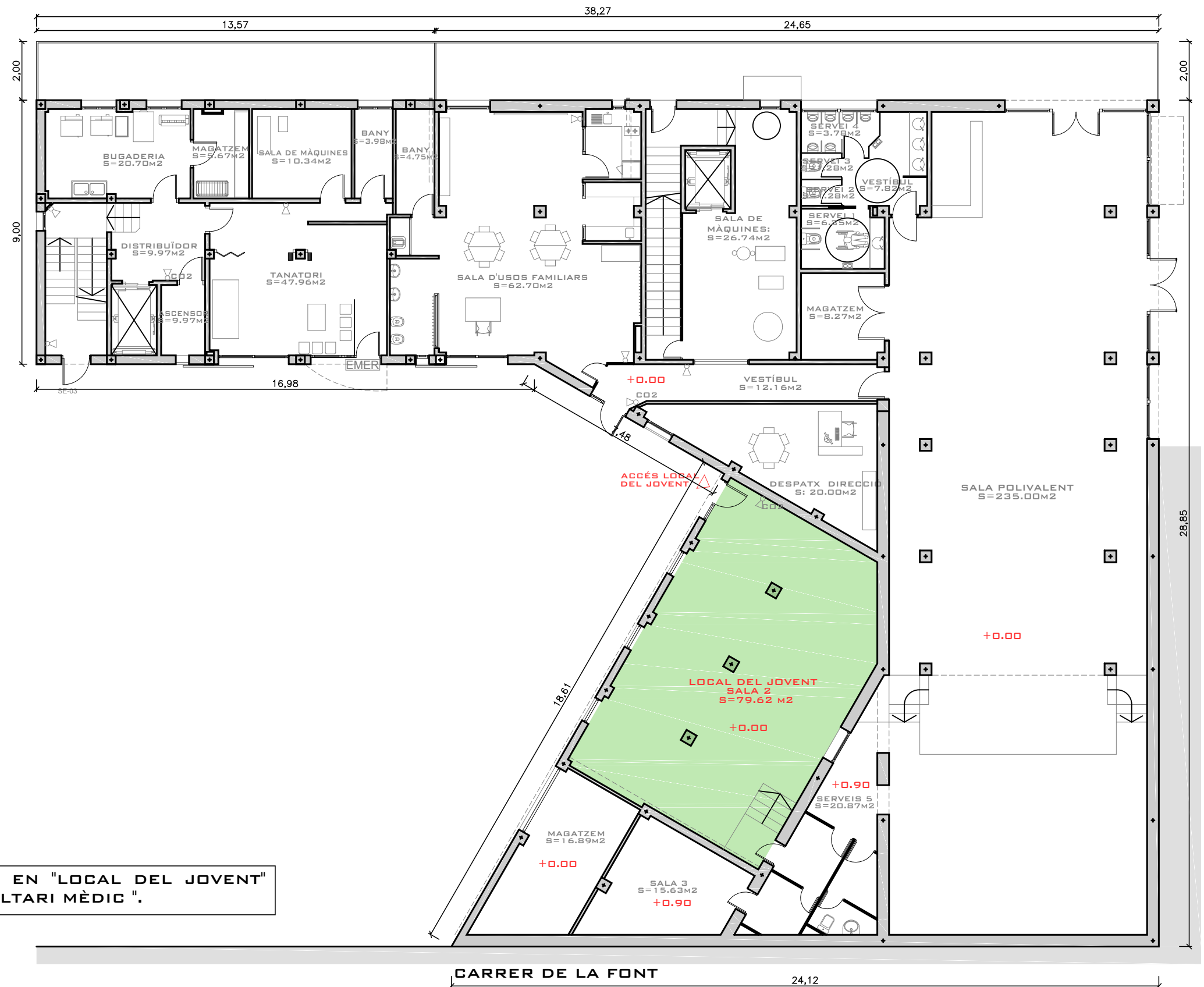
ESTAT ACTUAL - PLANTA BAIXA
