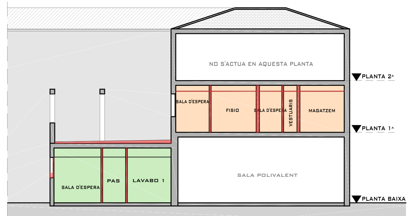
OBRA NOVA - ESTAT PROPOSTA - SECCIÓ TRANSVERSAL
