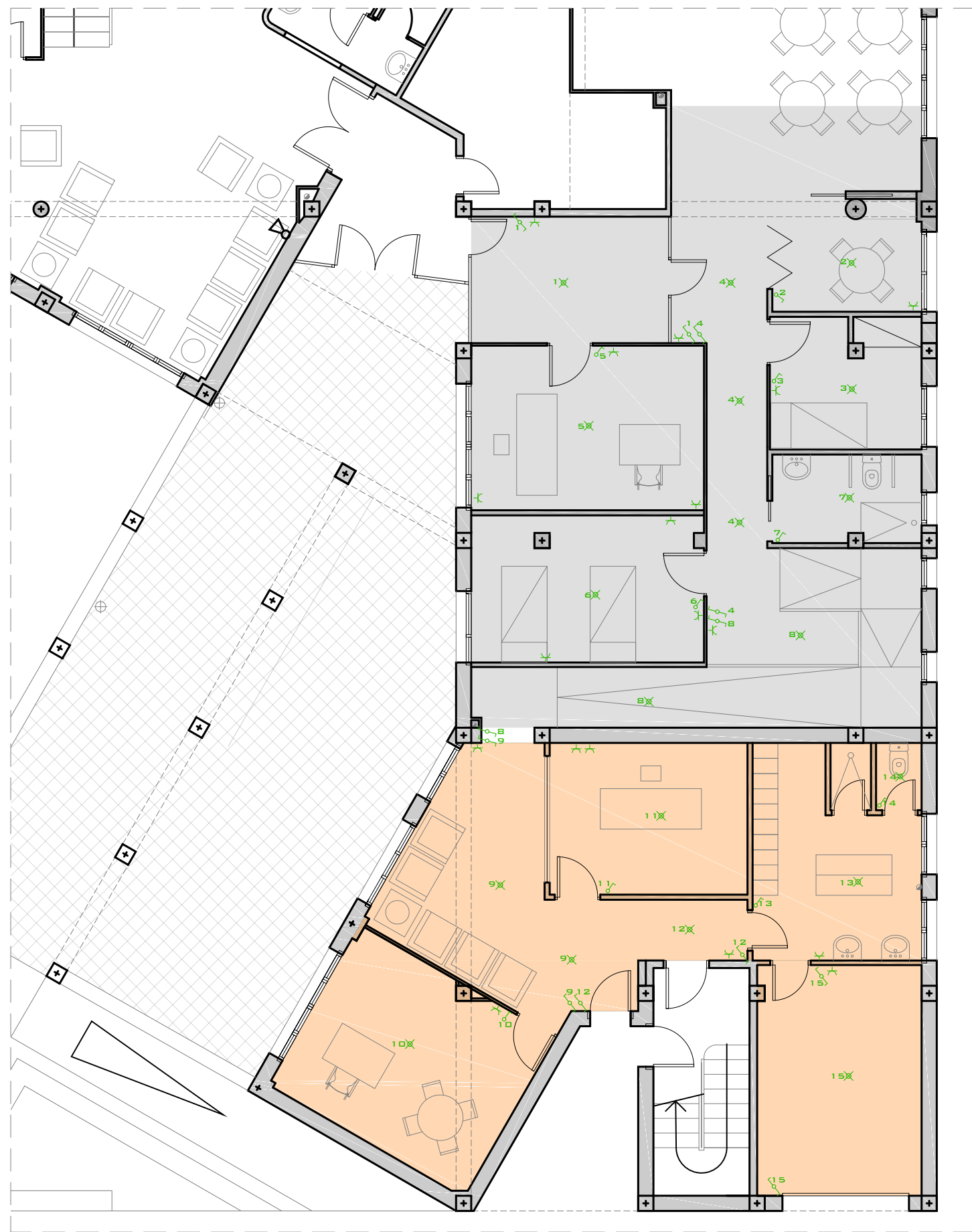
ELECTRICITAT I IL.LUMINACIÓ - PLANTA PRIMERA
