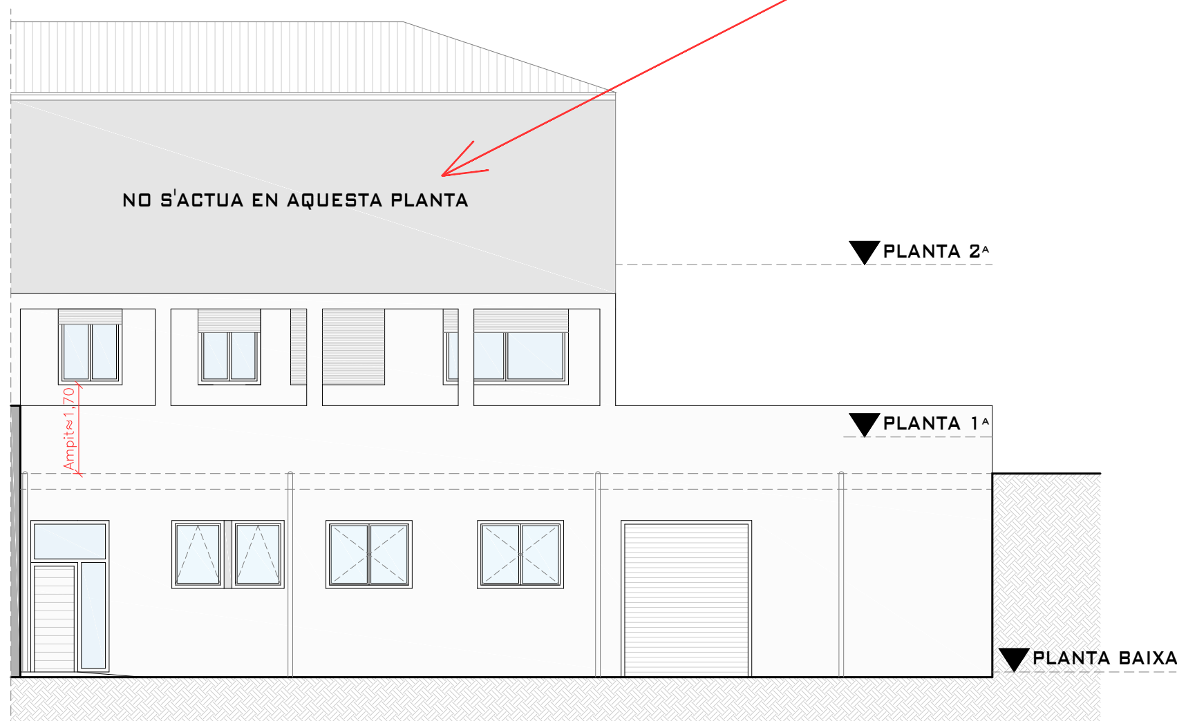
ESTAT PROPOSTA - ALÇAT FAÇANA EN ZONA D'ACTUACIÓ
