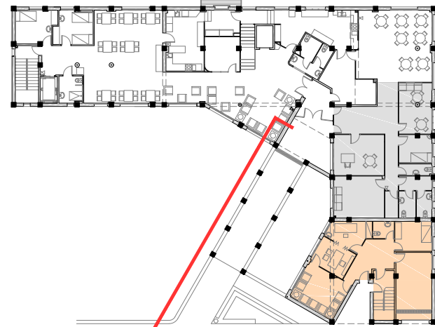
ESTAT ACTUAL - PLANTA PRIMERA
