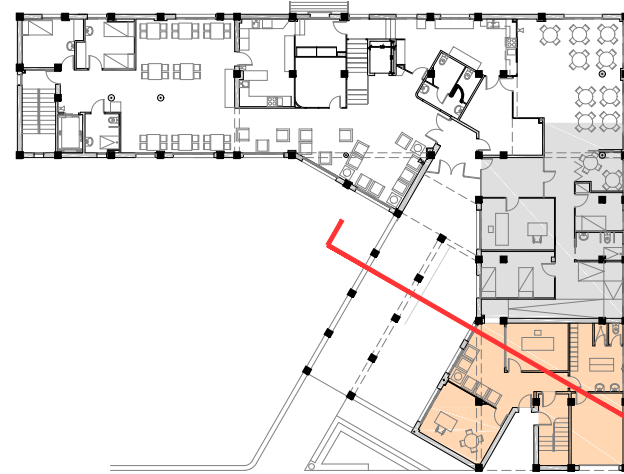
ESTAT PROPOSTA - PLANTA PRIMERA
