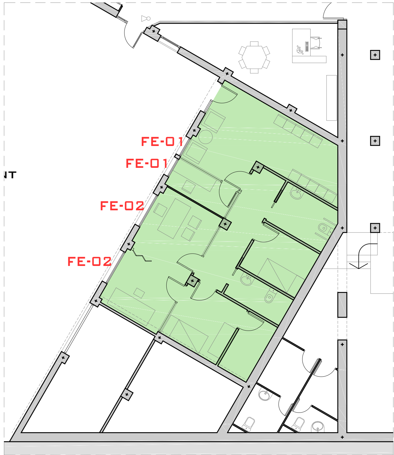
FUSTERIES EXTERIORS - ESTAT PROPOST - PLANTA BAIXA
