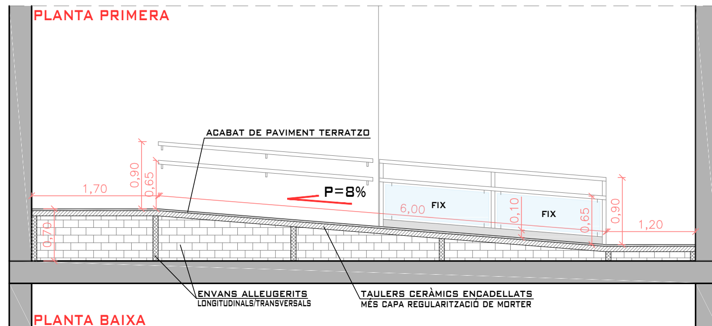
ESTAT PROPOSTA - RAMPA ACCESSIBLE (E:1/50) SECCIÓ LONGITUDINAL
