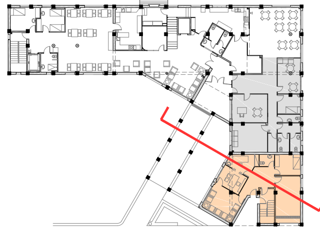
ESTAT ACTUAL - PLANTA PRIMERA
