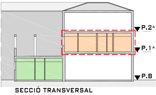
SECCIÓ TRANSVERSAL
