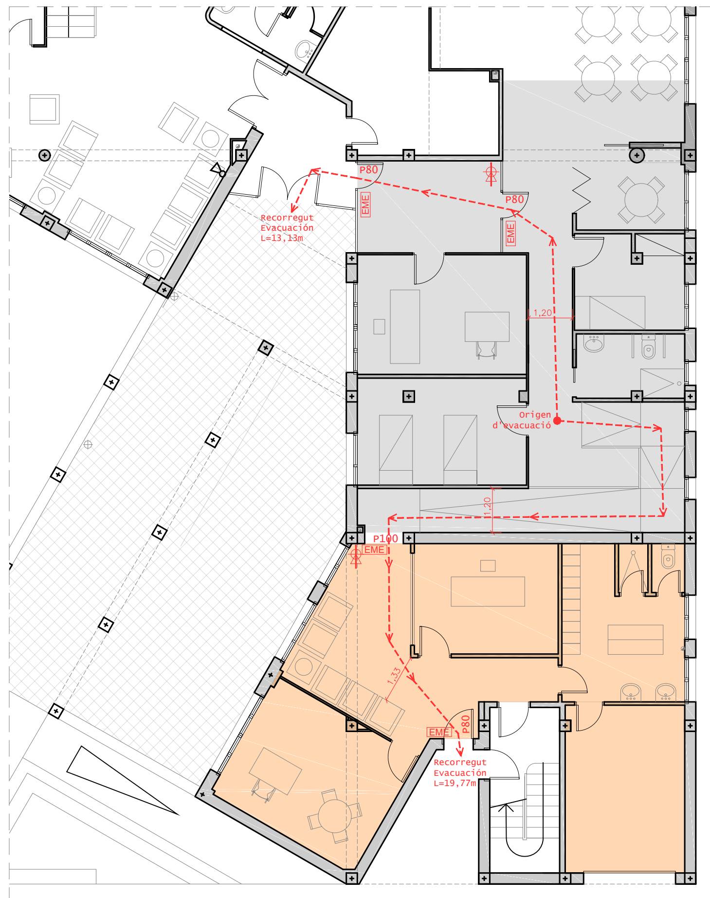
PROTECCIÓ CONTRA INCENDIS - ESTAT PROPOSTA - PLANTA PRIMERA
