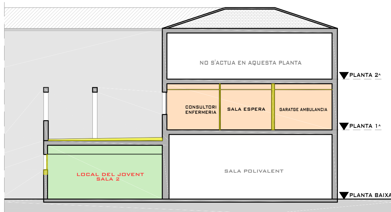
ENDERROCS - ESTAT ACTUAL - SECCIÓ TRANSVERSAL
