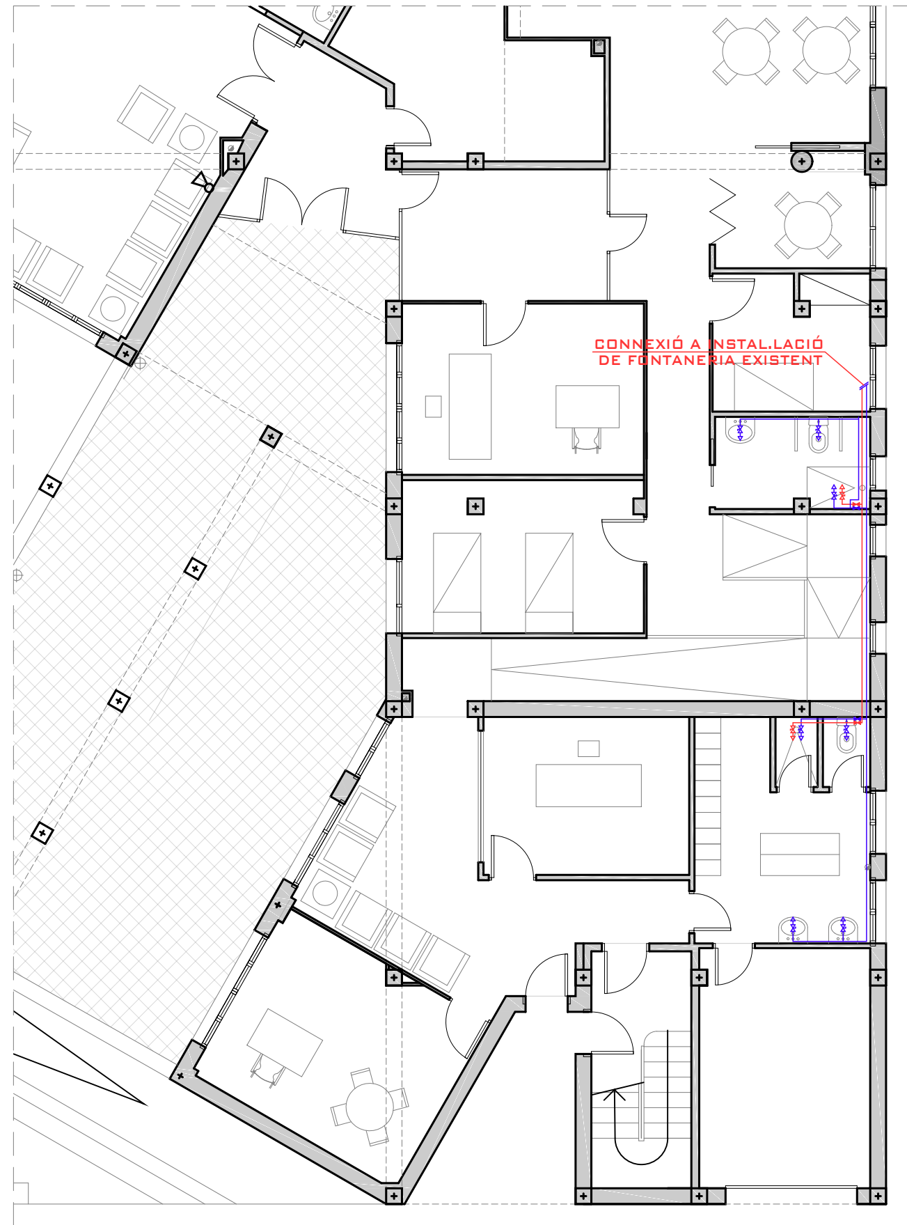
FONTANERIA - ESTAT PROPOSTA - PLANTA PRIMERA
