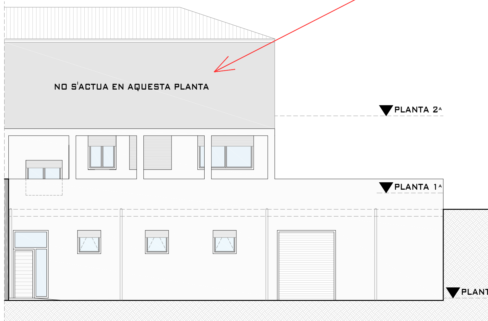
ESTAT ACTUAL - ALÇAT FAÇANA EN ZONA D'ACTUACIÓ
