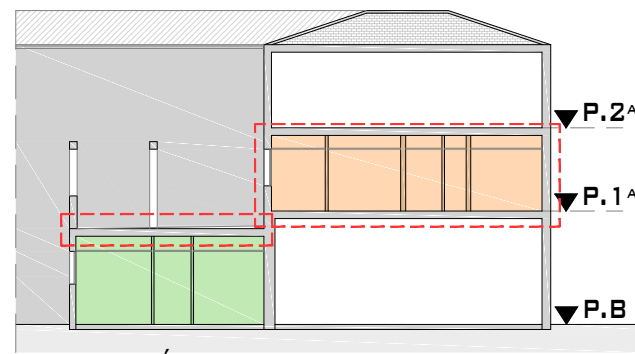
SECCIÓ TRANSVERSAL
