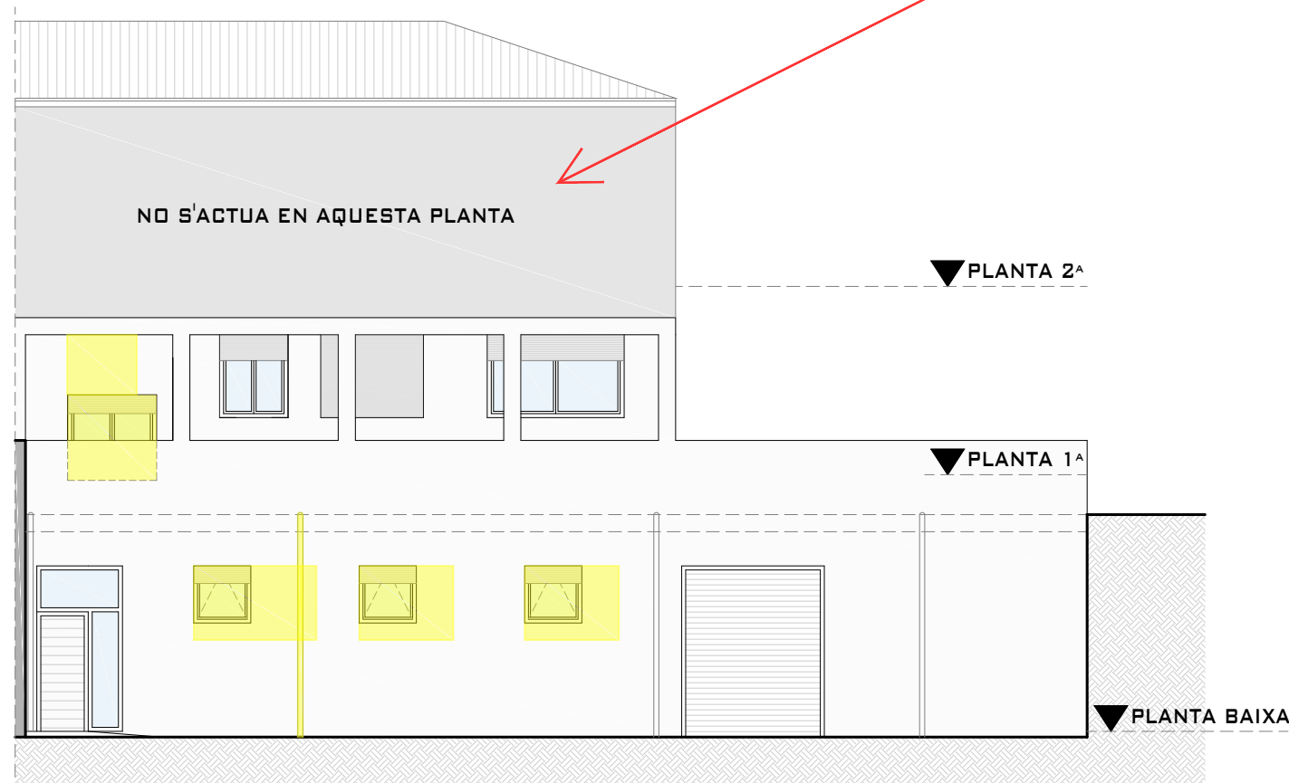
ENDERROC - ESTAT ACTUAL - ALÇAT FAÇANA EN ZONA D'ACTUACIÓ
