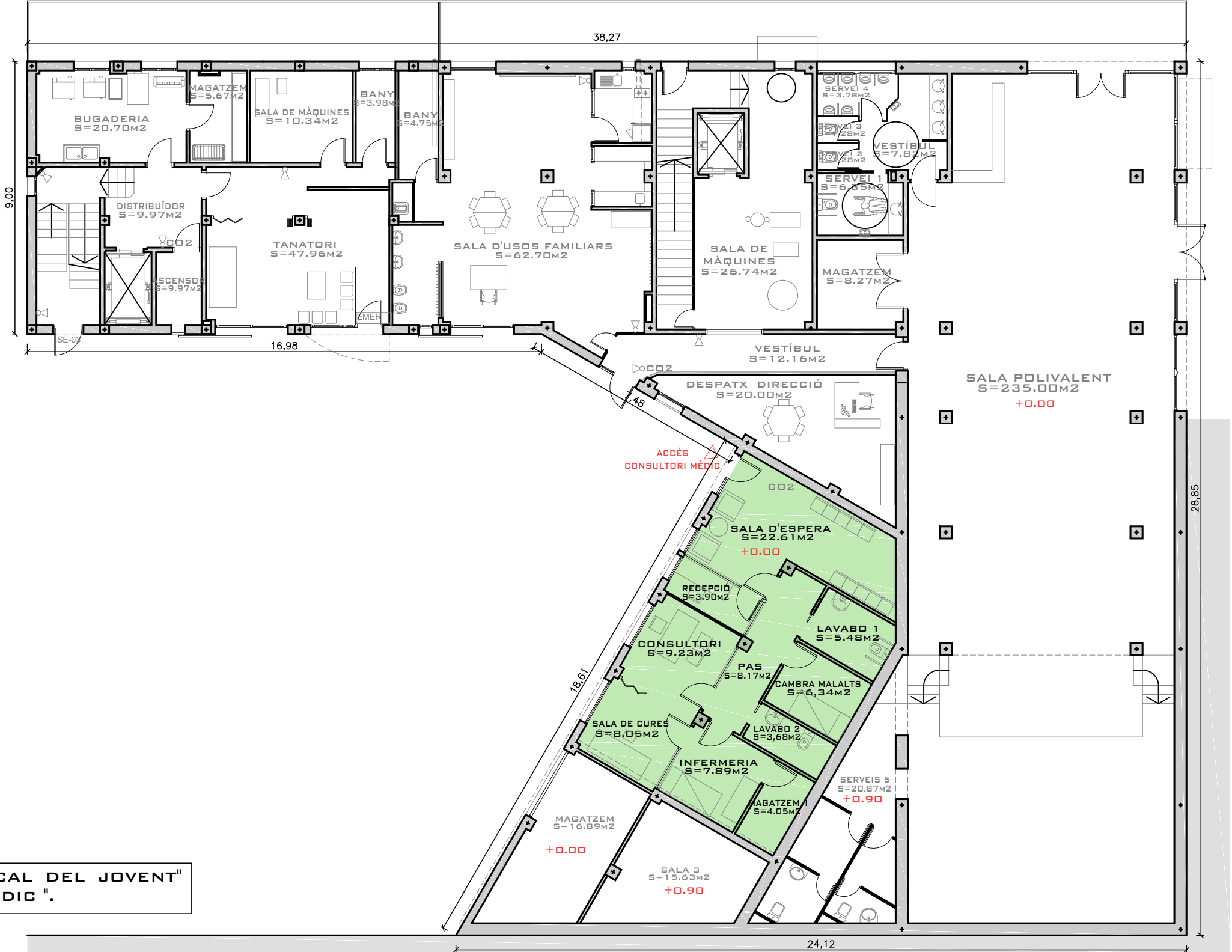
ESTAT PROPOSTA - PLANTA BAIXA COMPLETA
