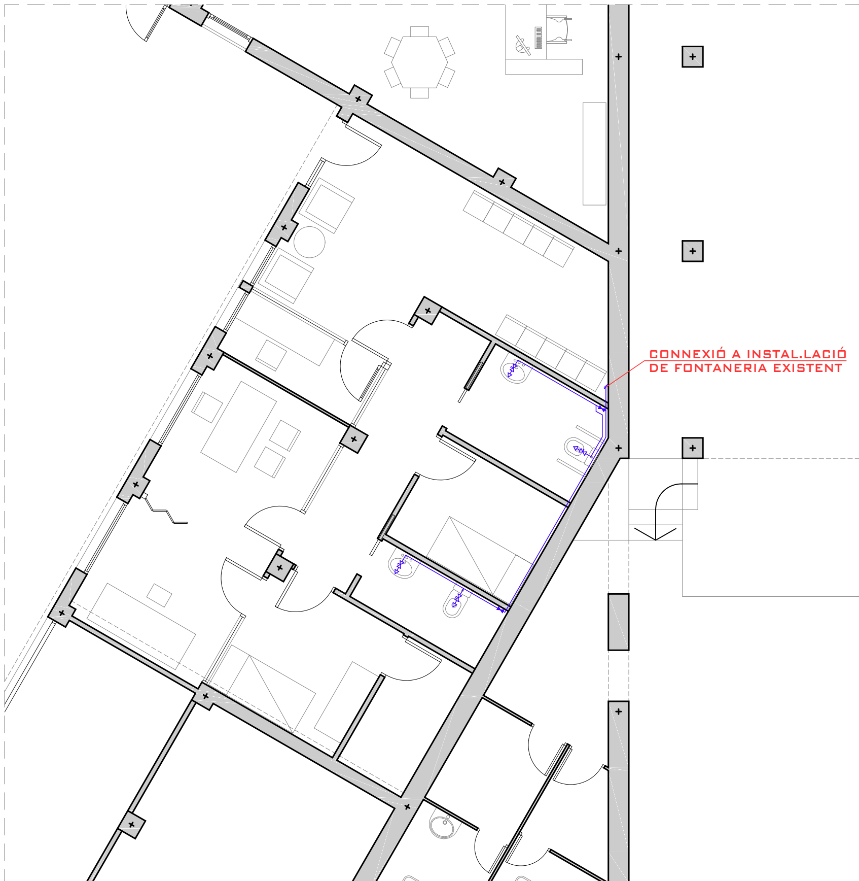
FONTANERIA - ESTAT PROPOSTA - PLANTA BAIXA
