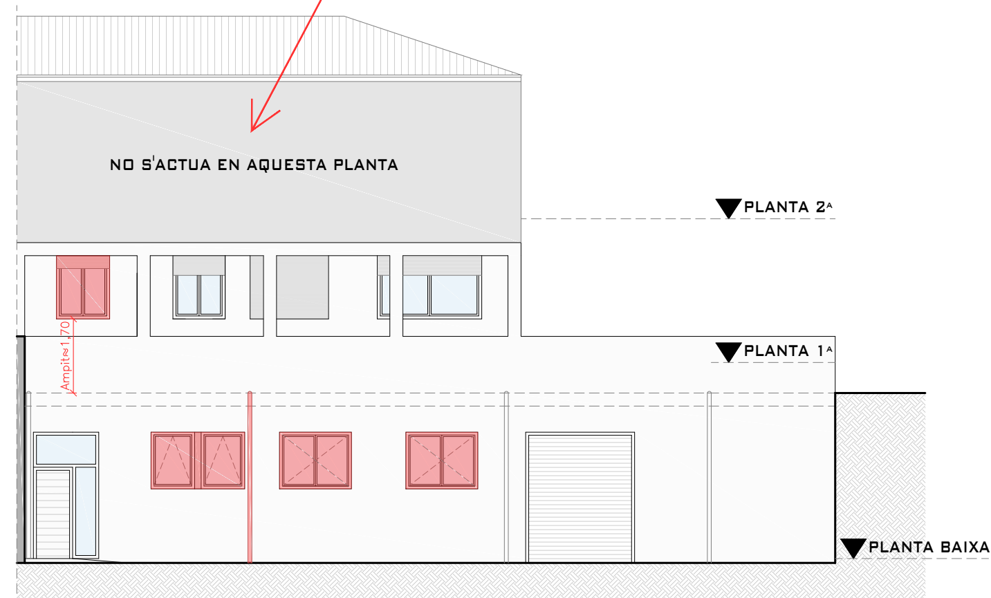
OBRA NOVA - ESTAT PROPOSTA - ALÇAT FAÇANA EN ZONA D'ACTUACIÓ
