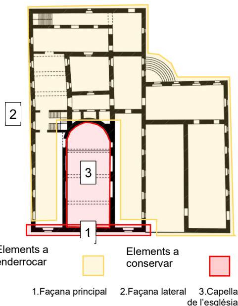
Planta Baixa de l'edifici
