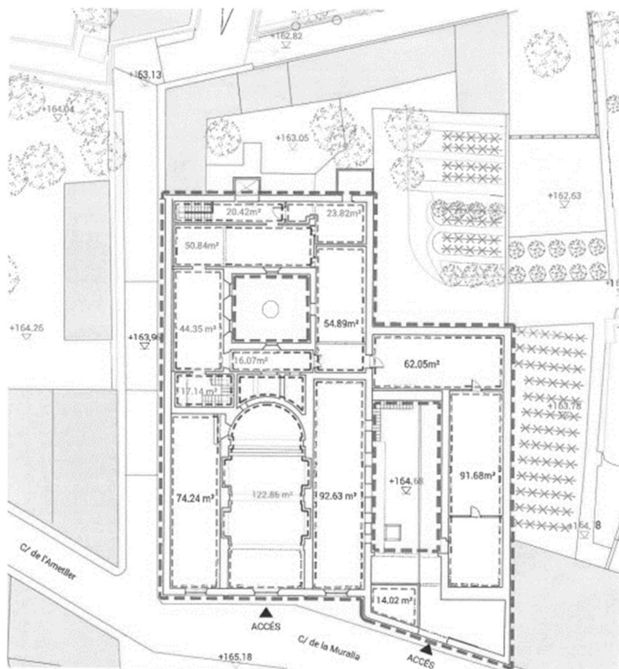
Planta Baixa
