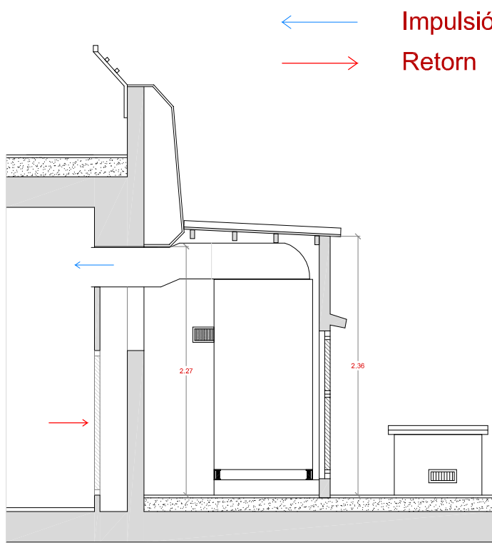
SECCIÓ A-A'
