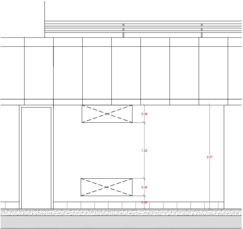
Secció B-B'
