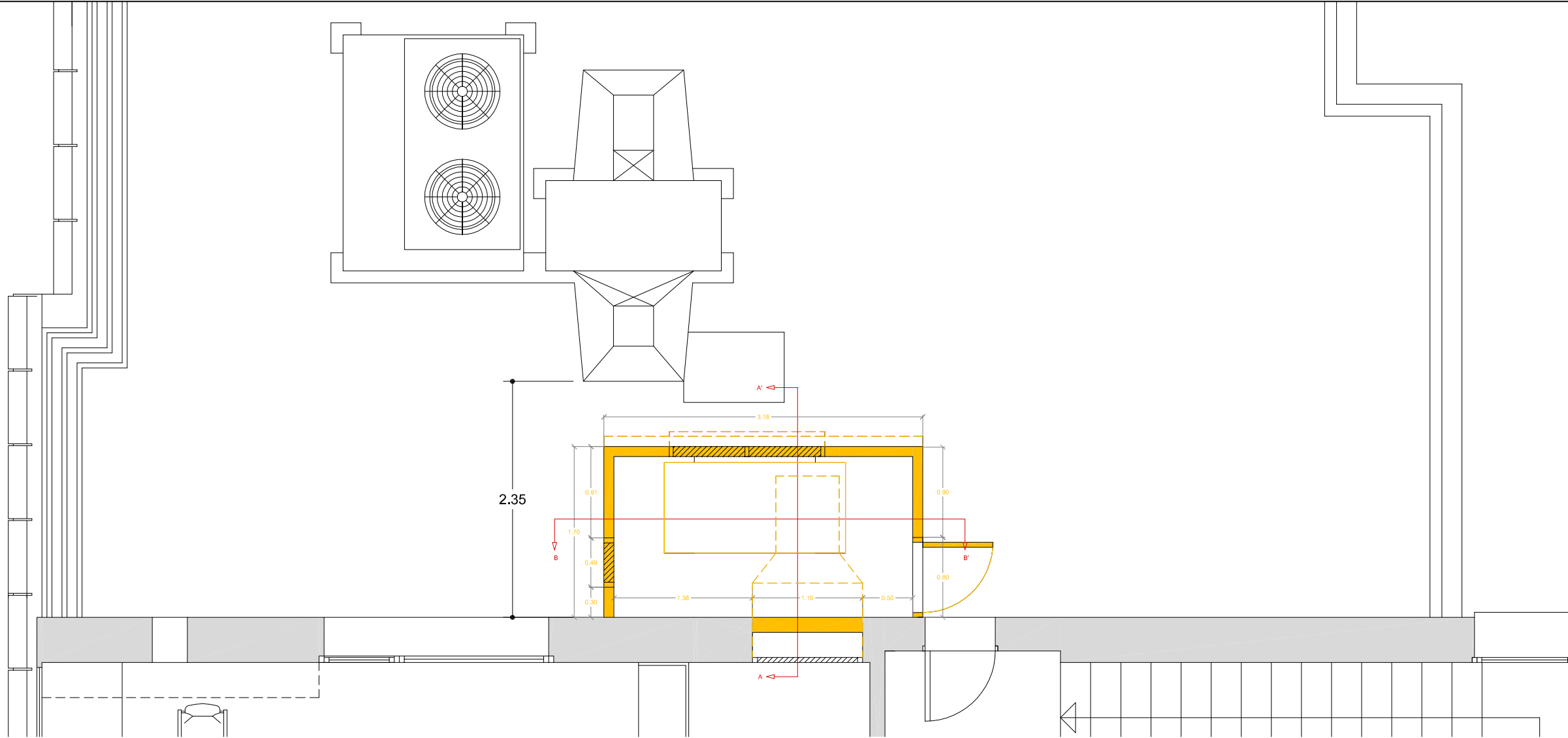
PLANTA
