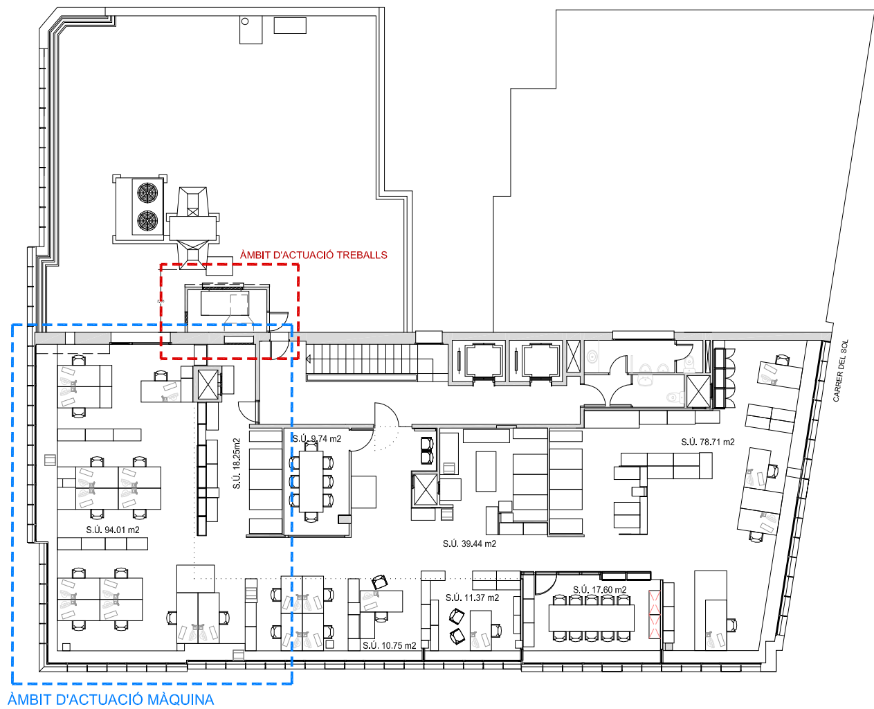
PLANTA 6ª
