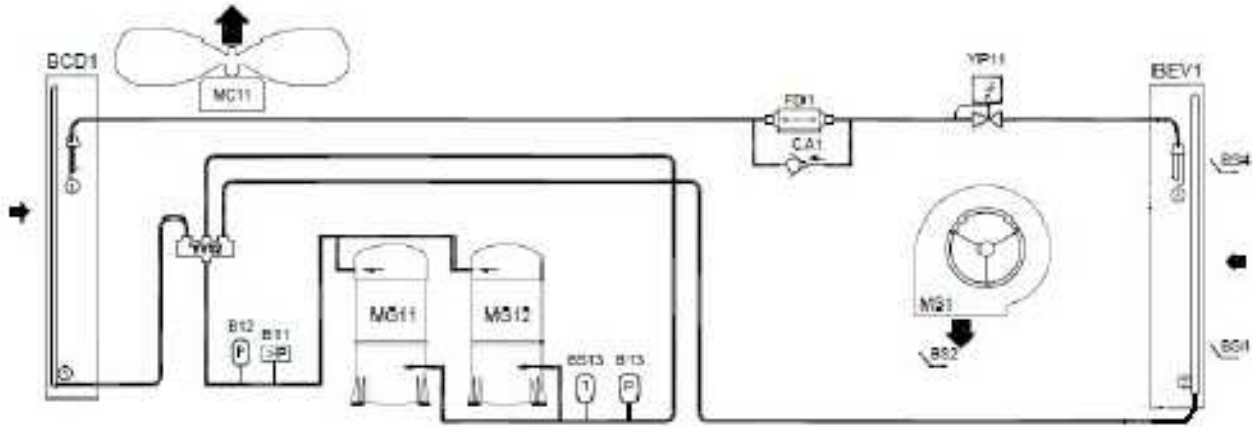
Circuit frigorífic
