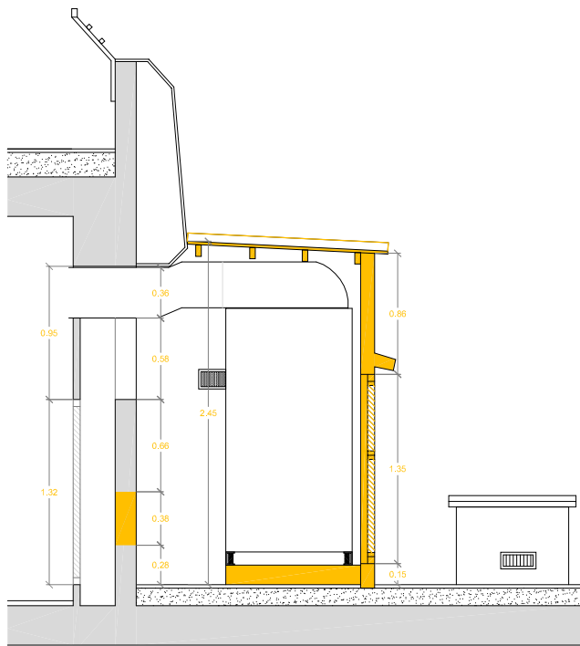
SECCIÓ A-A'
