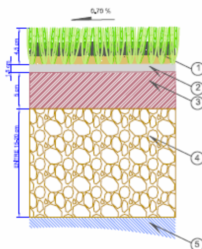
DETALLE SECCION DEL CAMPO DE FUTBOL SOCCER PRO MAX "S" 45 mm y Base elástica de 15 mm
