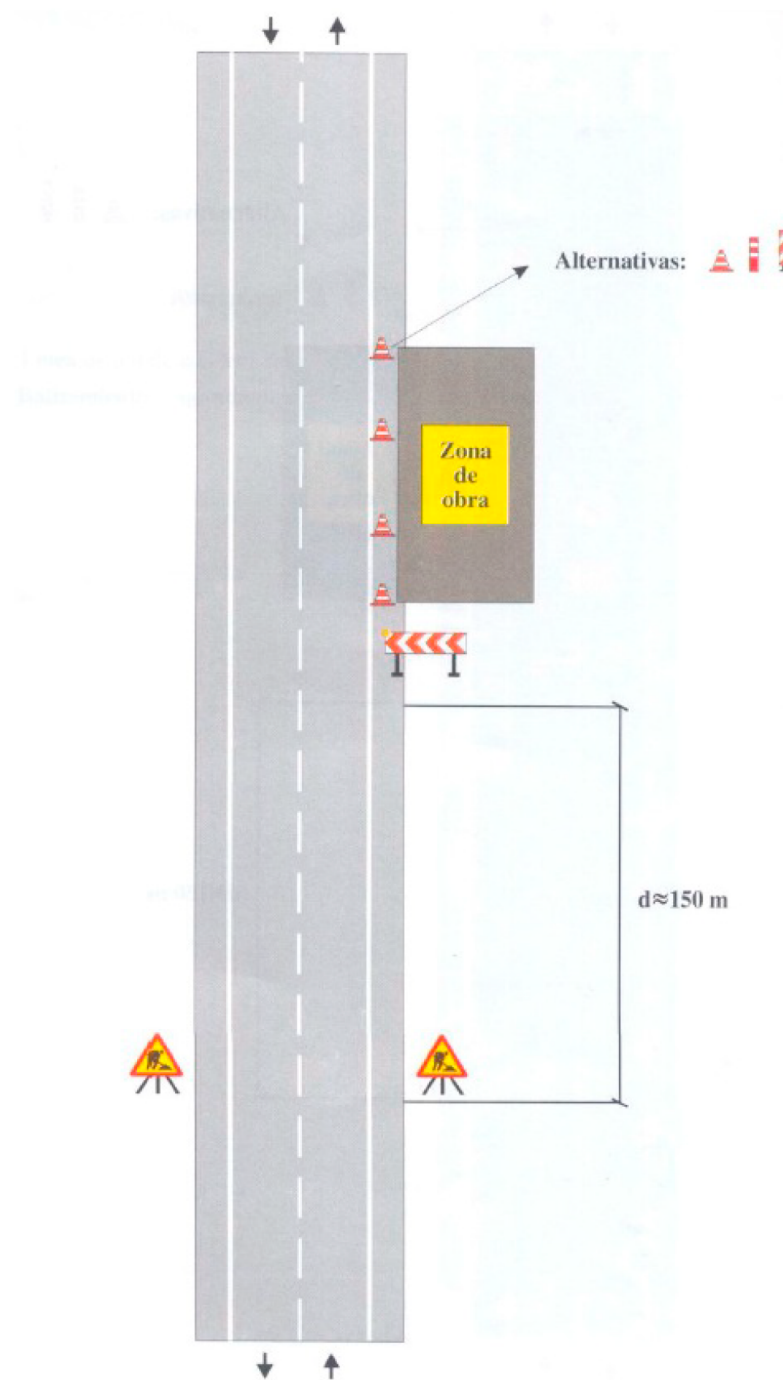
DETALL VIA DE DOBLE SENTIT DE CIRCULACIÓ CALÇADA ÚNICA AMB 2 CARRILS. ZONA DE L'OBRA EN VORERA
