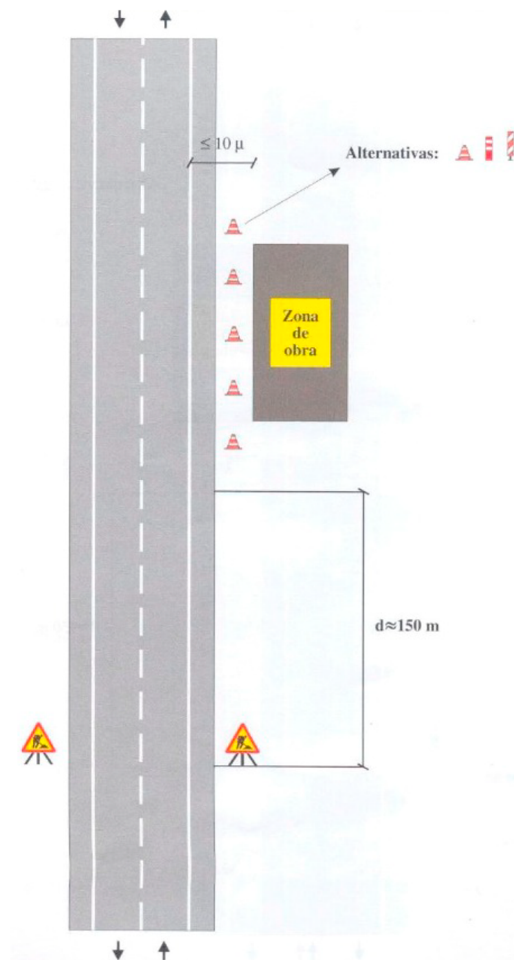
DETALL VIA DE DOBLE SENTIT DE CIRCULACIÓ CALÇADA ÚNICA AMB 2 CARRILS. ZONA DE L'OBRA EXTERIOR A LA PLATAFORMA
