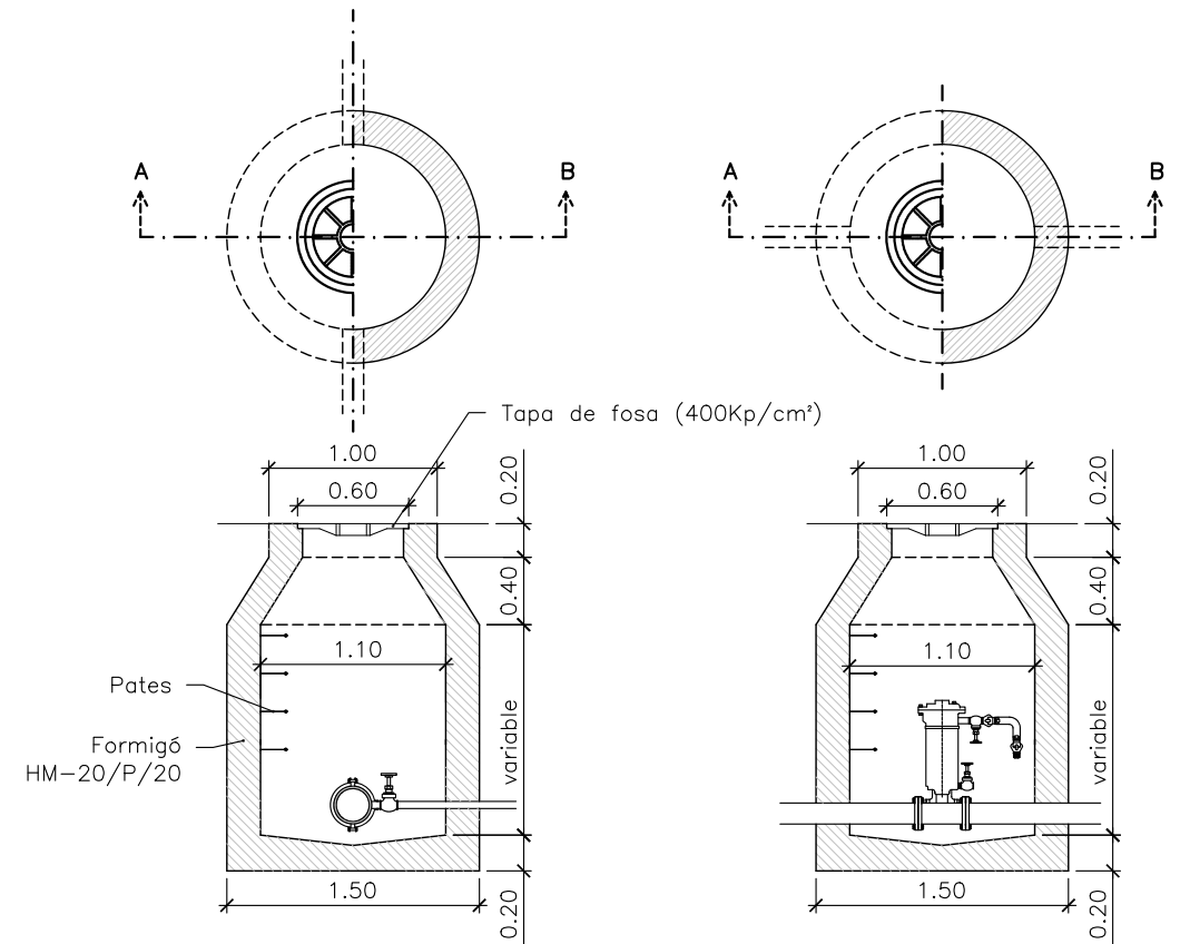
ARQUETA DESGUÀS E: 1/50
