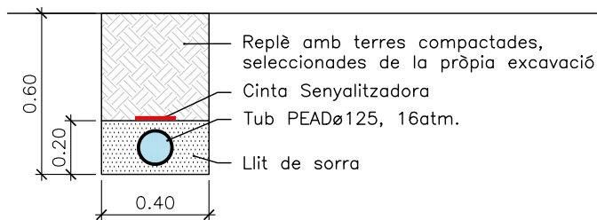
RASA TIPUS EN TERRENY NATURAL E: 1/25
