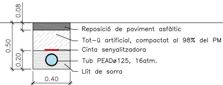
RASA TIPUS A EIX DE VIAL
