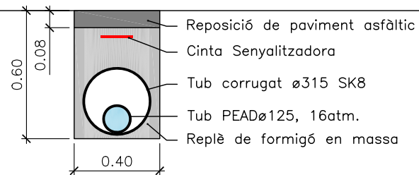
RASA TIPUS EN CREUAMENTS VIAL
