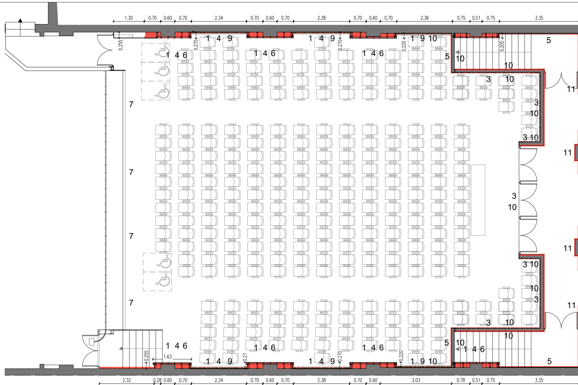
Planta platea
