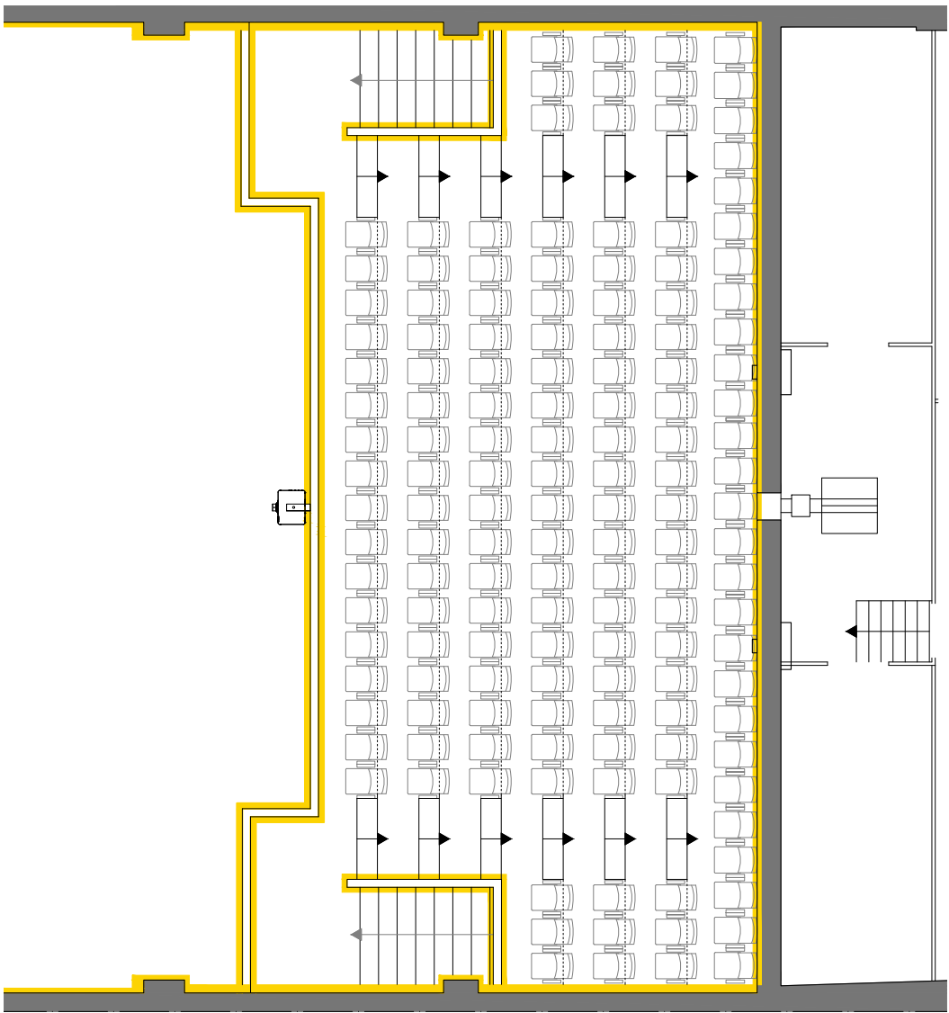
Planta amfiteatre
