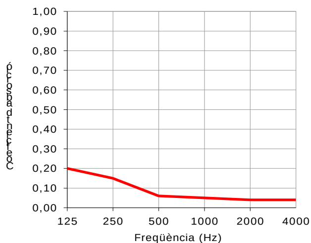
Figura 5.5: Coeficients d'absorció acústica dels laterals superior de la sala
