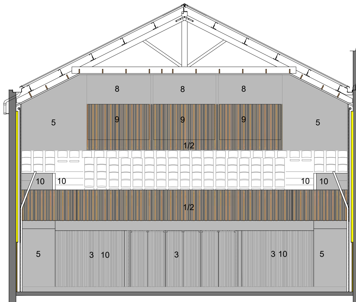
Secció vista amfiteatre
