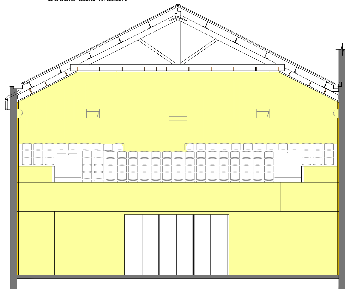
Secció vista posterior sala
