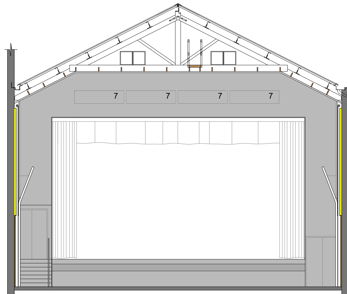
Secció vista escenari
