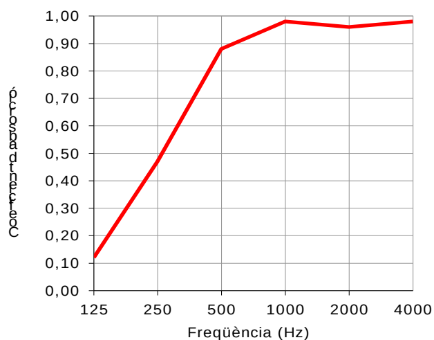
Figura 5.3: Coeficients d'absorció acústica dels laterals inferiors de la sala
