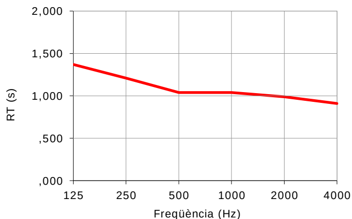
Figura 3.1: Valors del temps de reverberació mesurats amb la sala buida
