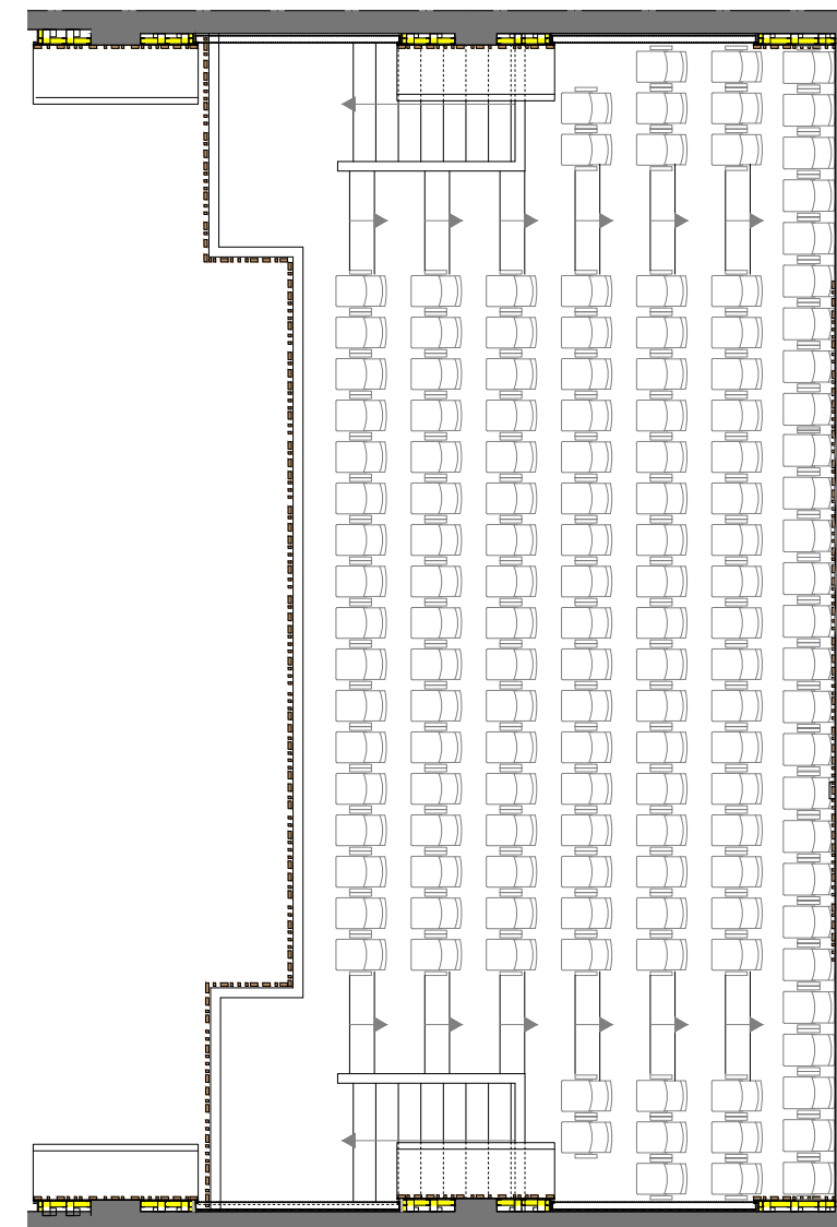
Planta amfiteatre
