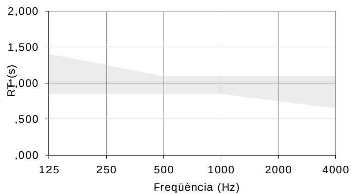
Figura 4.2: Interval recomanat de variació dels valors del temps de reverberació (Cinema). Configuració sala amb cortines.
