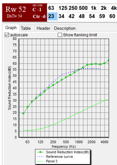
Figura 5.14: Aïllament acústic solució coberta
