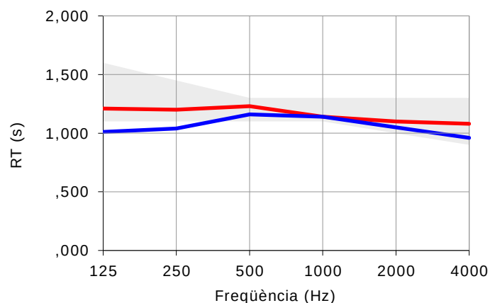
Figura 7.1: Temps de reverberació i marges recomanats dels valors del temps de reverberació (Teatre – Música).
