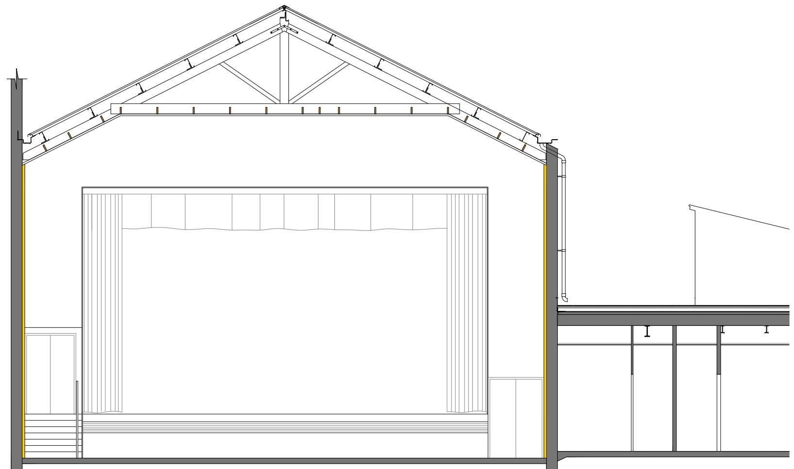
Secció vista frontal sala
