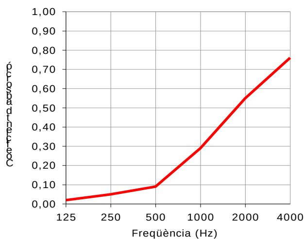
Figura 5.4: Coeficients d'absorció acústica de les parets posteriors de la sala
