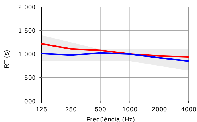
Figura 7.2: Temps de reverberació i marges recomanats dels valors del temps de reverberació (cinema – conferències). Configuració sala amb cortines.
