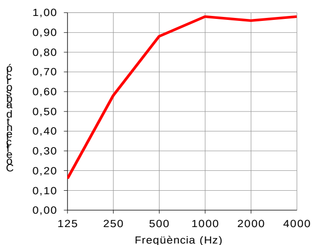
Figura 5.11: Coeficients d'absorció acústica de les parets posteriors de la sala
