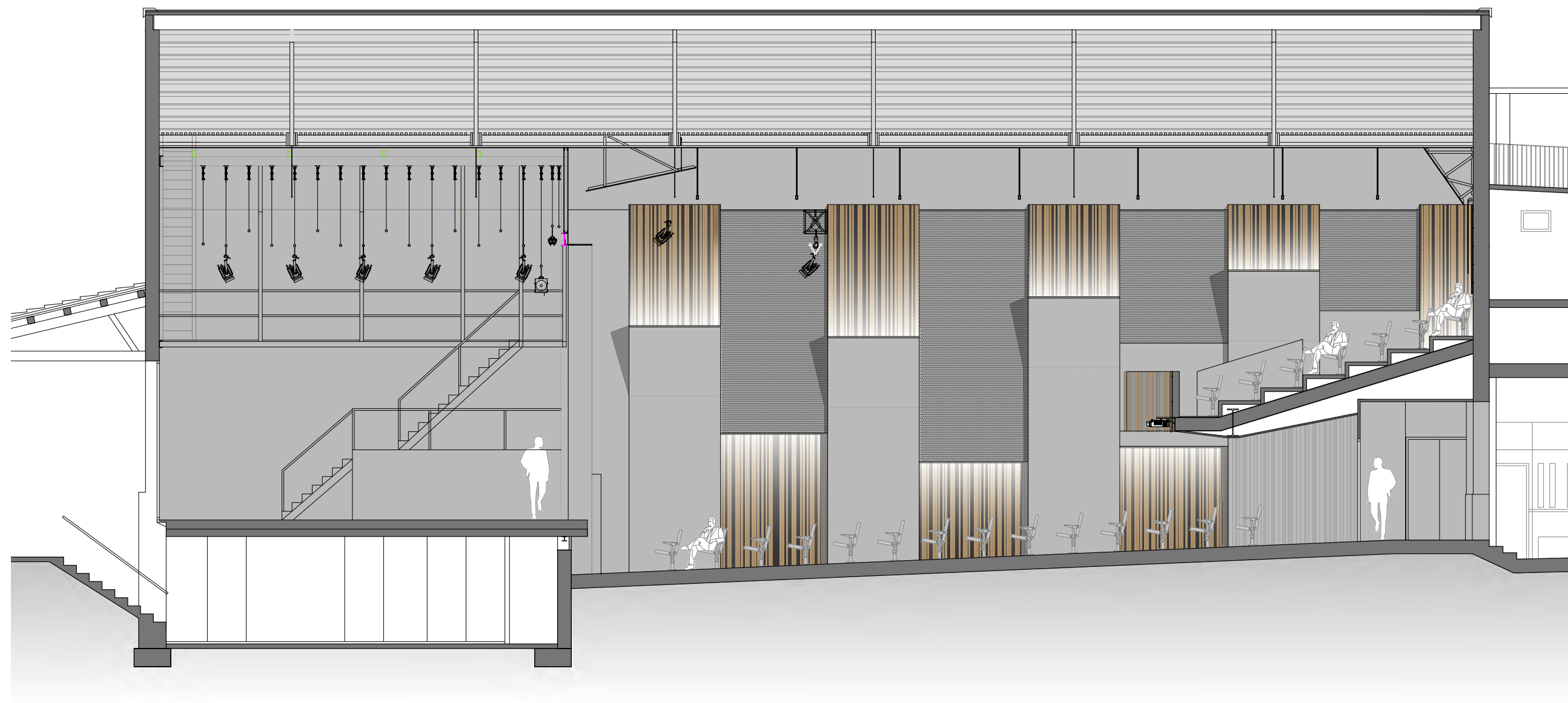
Alçat interior sala Mozart
