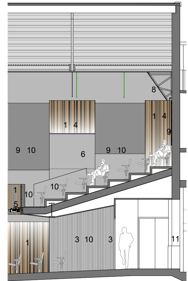
Secció per l'amfiteatre i el vestíbul
