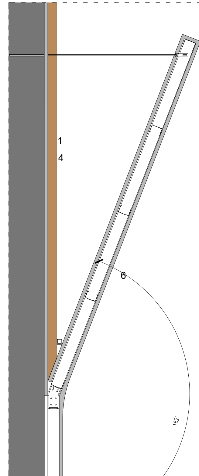
Detall tipus reflector acústic parets sala e: 1/10
