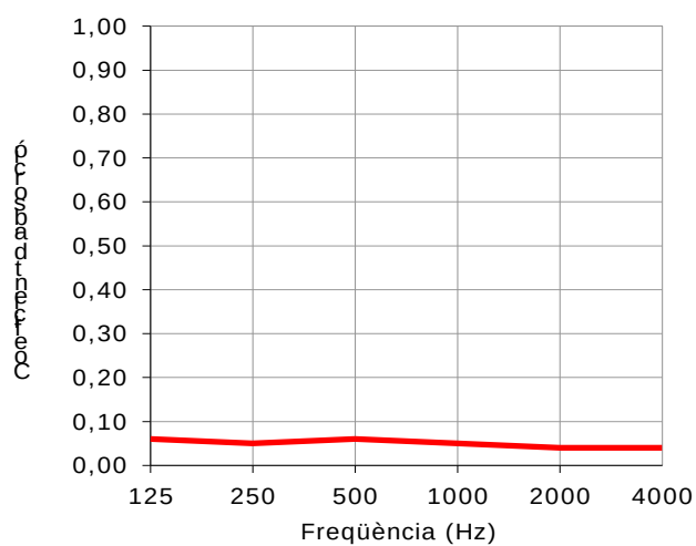
Figura 5.9: Coeficients d'absorció acústica dels panells reflectors de la sala
