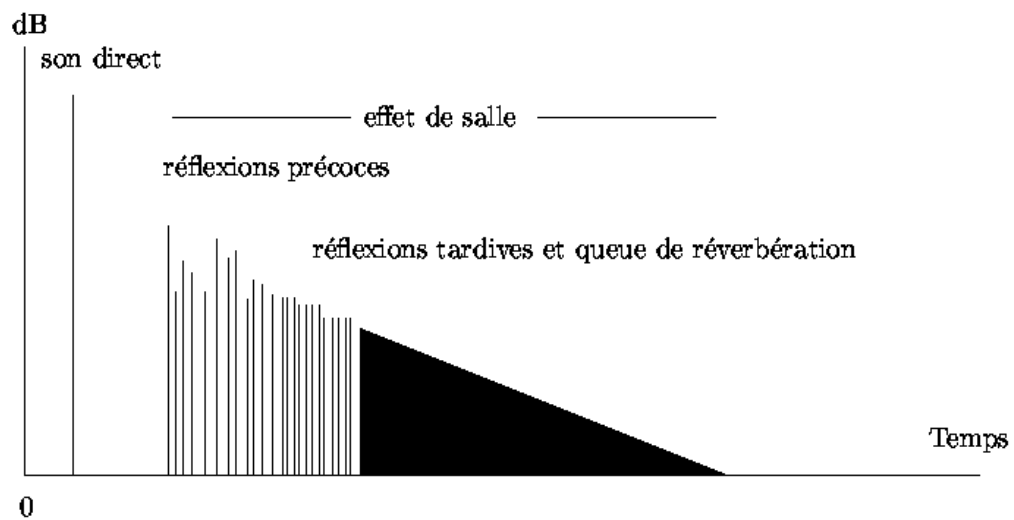
Figura 2.1: Resposta impulsional tipus d'una sala
