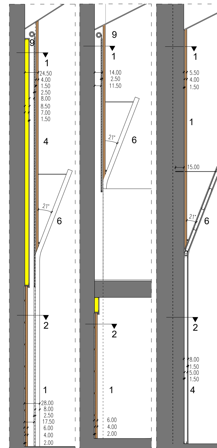
Secció A
