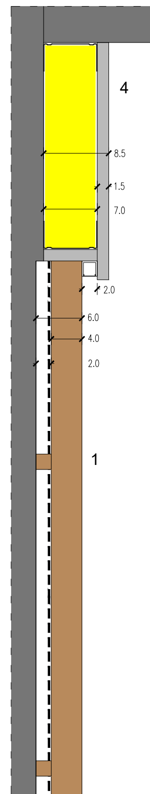
Detall tipus rastrells amb llistons e: 1/5
