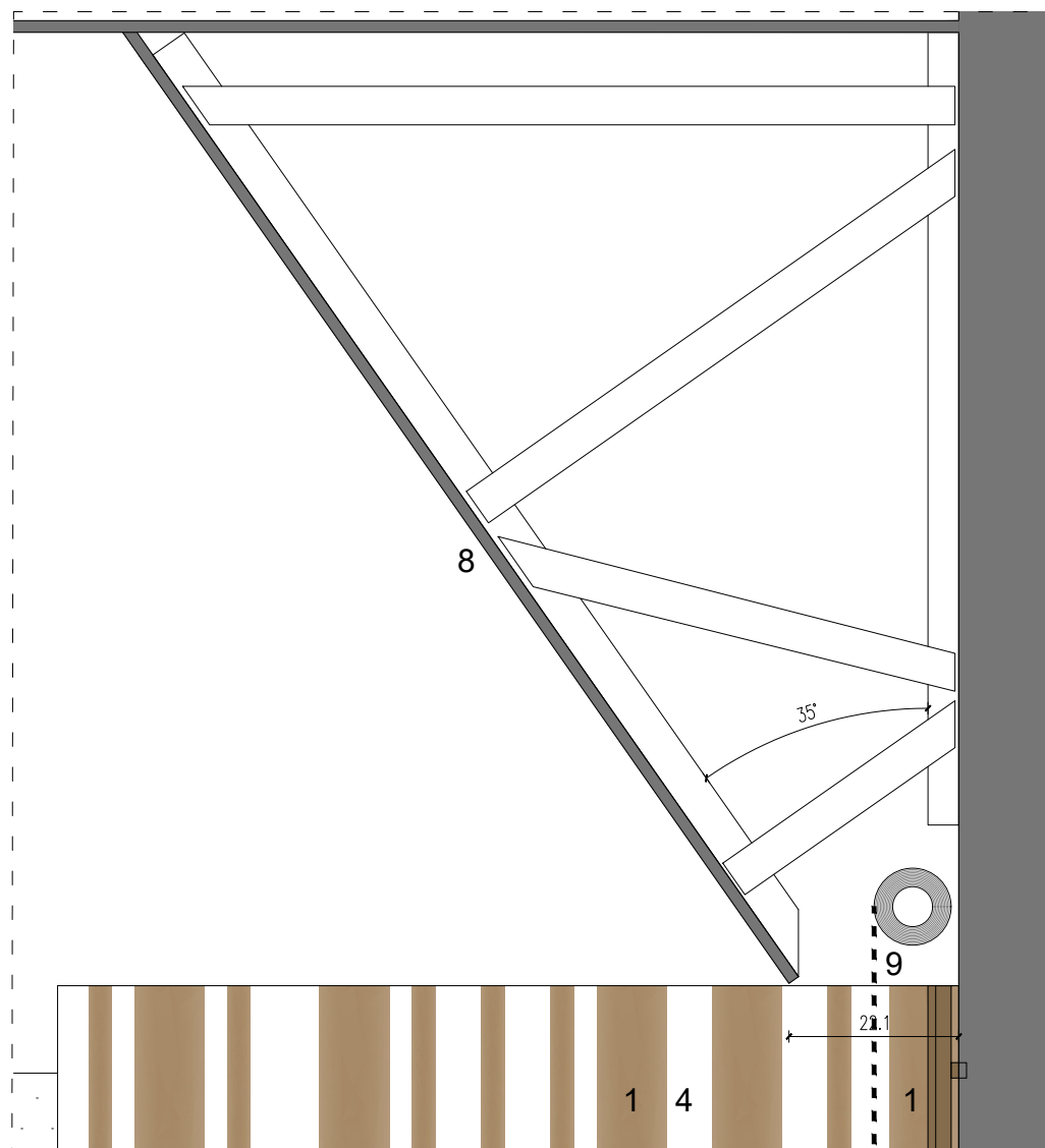
Detall reflector acústic fons de la sala
