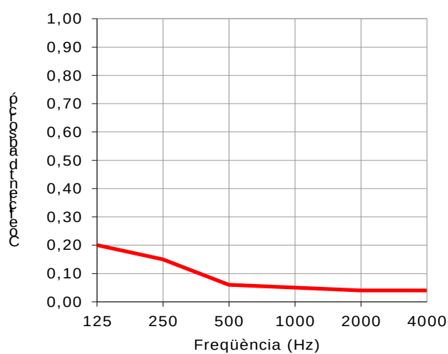
Figura 5.13: Coeficients d'absorció acústica dels laterals superior de la sala
