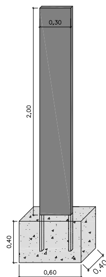
Instal·lació totem vertical d'alumini
