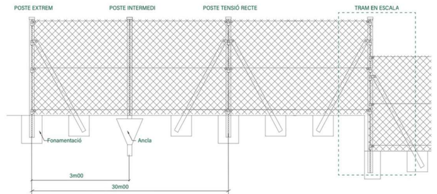
Esquema general de muntatge tanca malla metàl·lica
