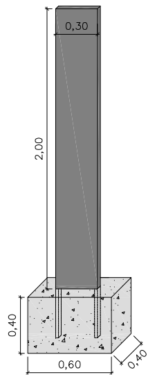
Reubicació totem vertical d'alumini
