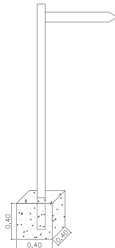
Senyal direccional 1 direcció
