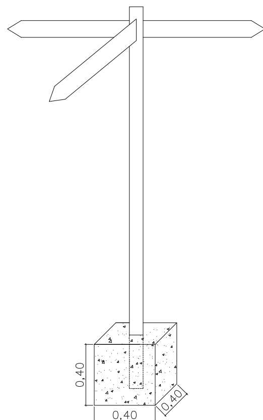
Senyal direccional 3 direccions
