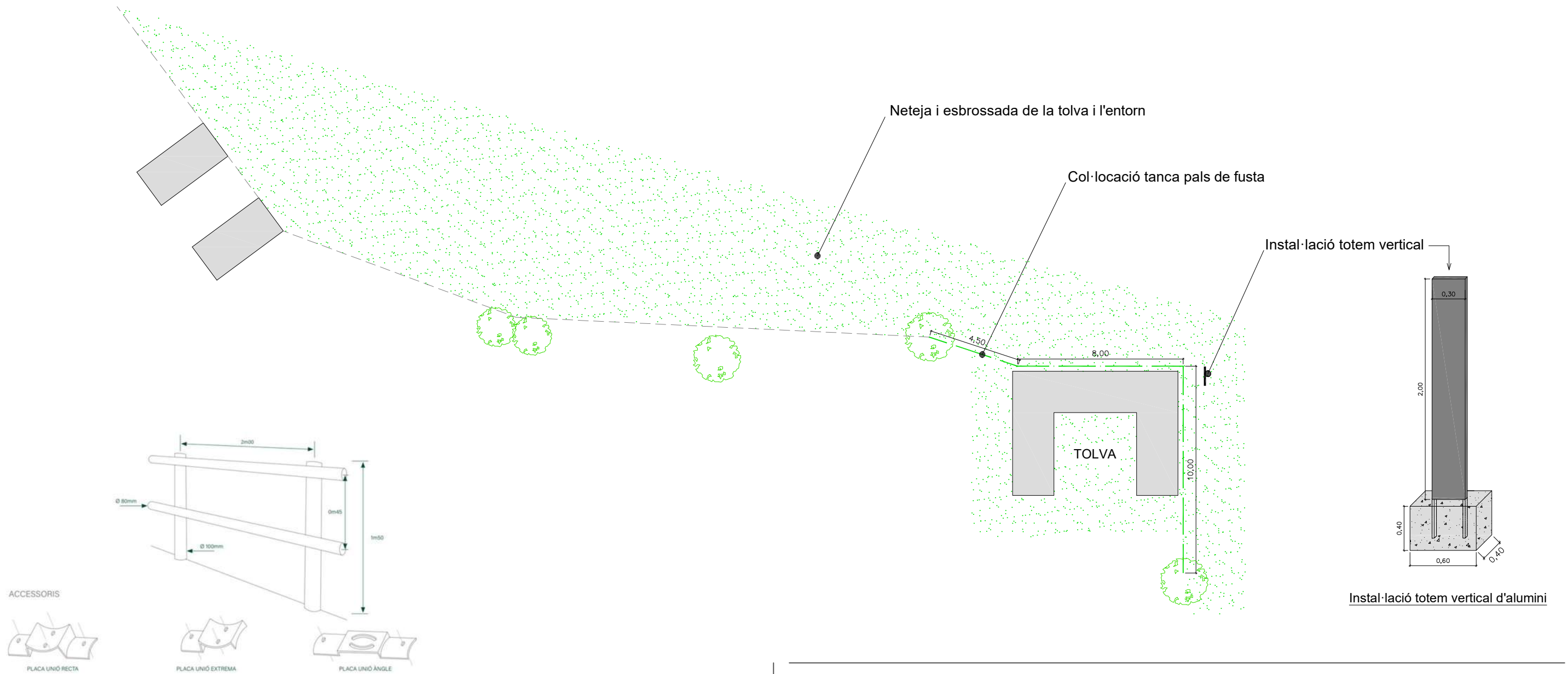
Esquema general de muntatge tanca pals de fusta
