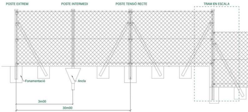
Esquema general de muntatge tanca malla metàl·lica
