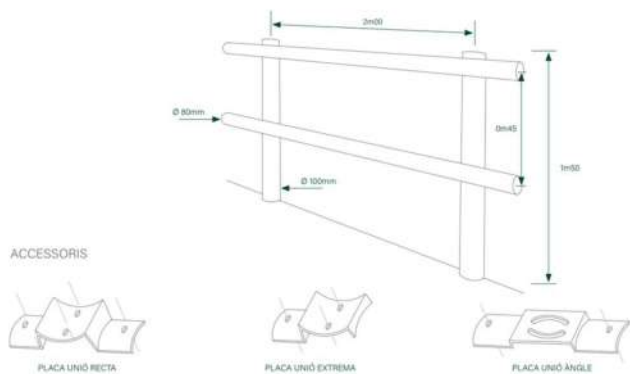
Esquema general de muntatge tanca pals de fusta
