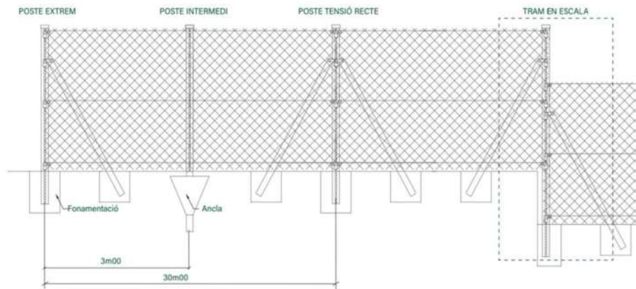
Esquema general de muntatge tanca malla metàl·lica
