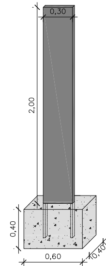
Totem vertical d'alumini
