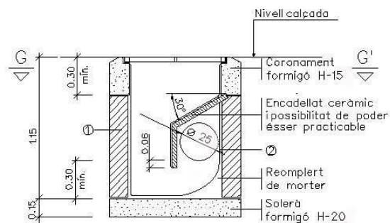
SECCIÓ F-F'
