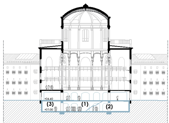
Fig. 8 Secció esquemàtica B-B' – Proposta
