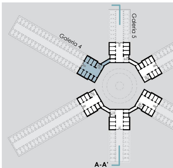
Fig. 5 Planta sotterrani – Estat actual
