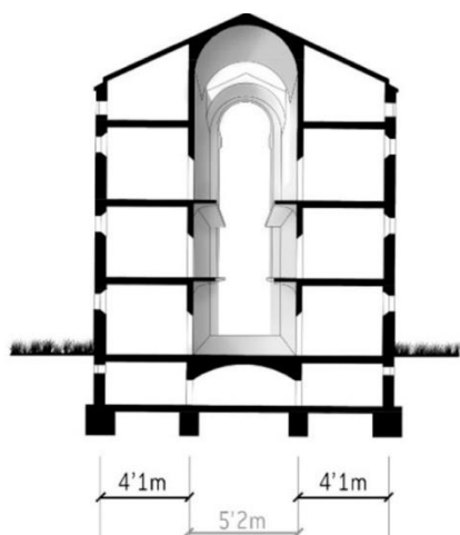
Fig. 2 Secció d'una galeria tipus. Estat actual
