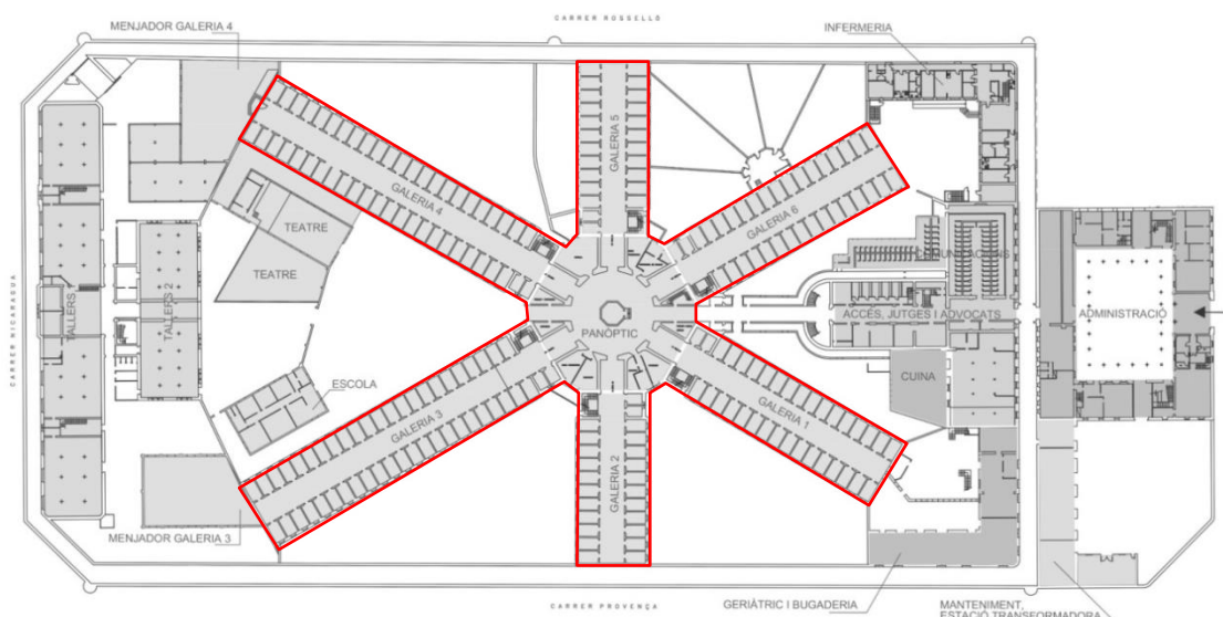
Fig. 1 Esquema de l'edifici. Dècada del 2000
