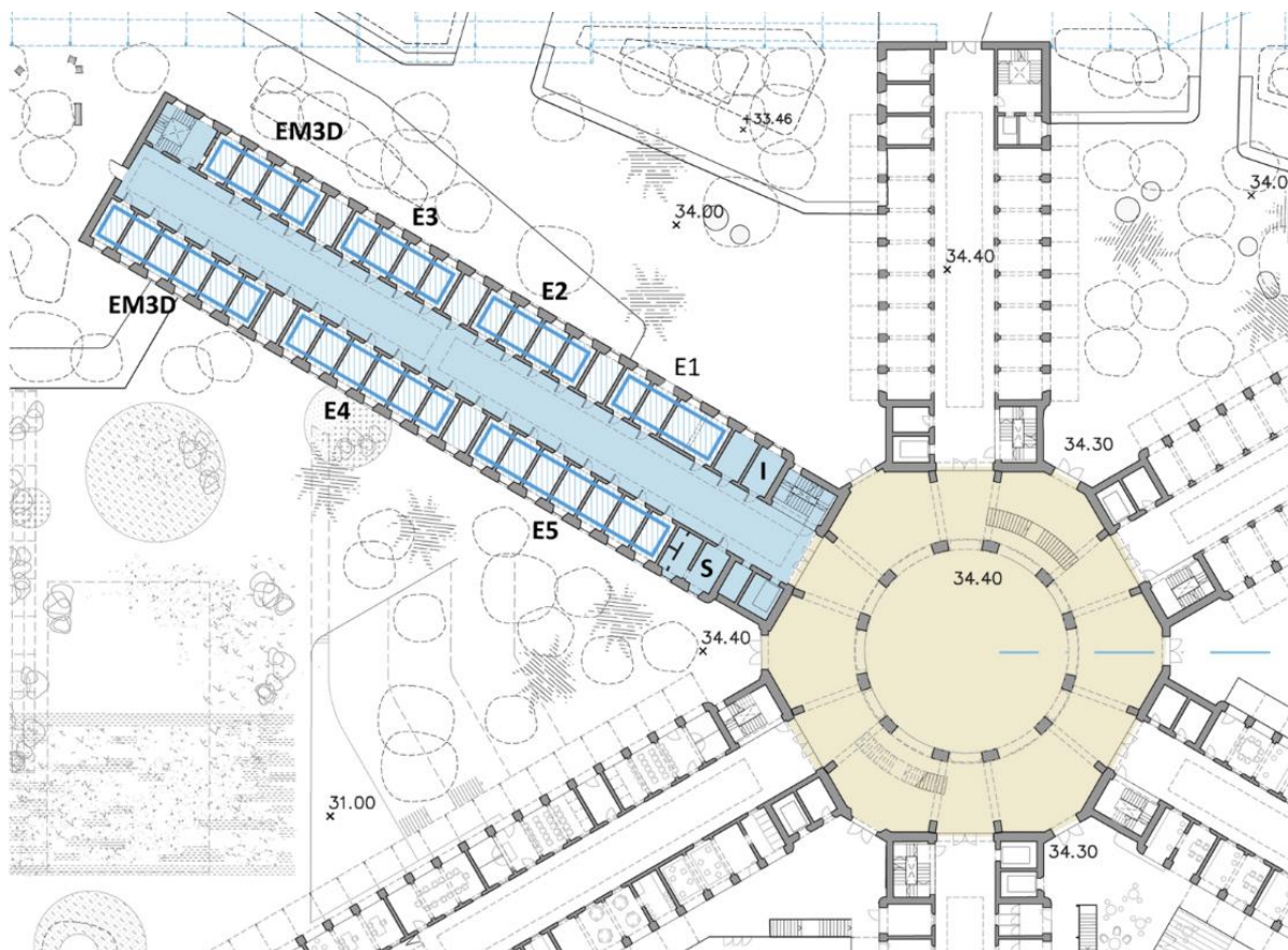
Planta primera proposta +36,10m
