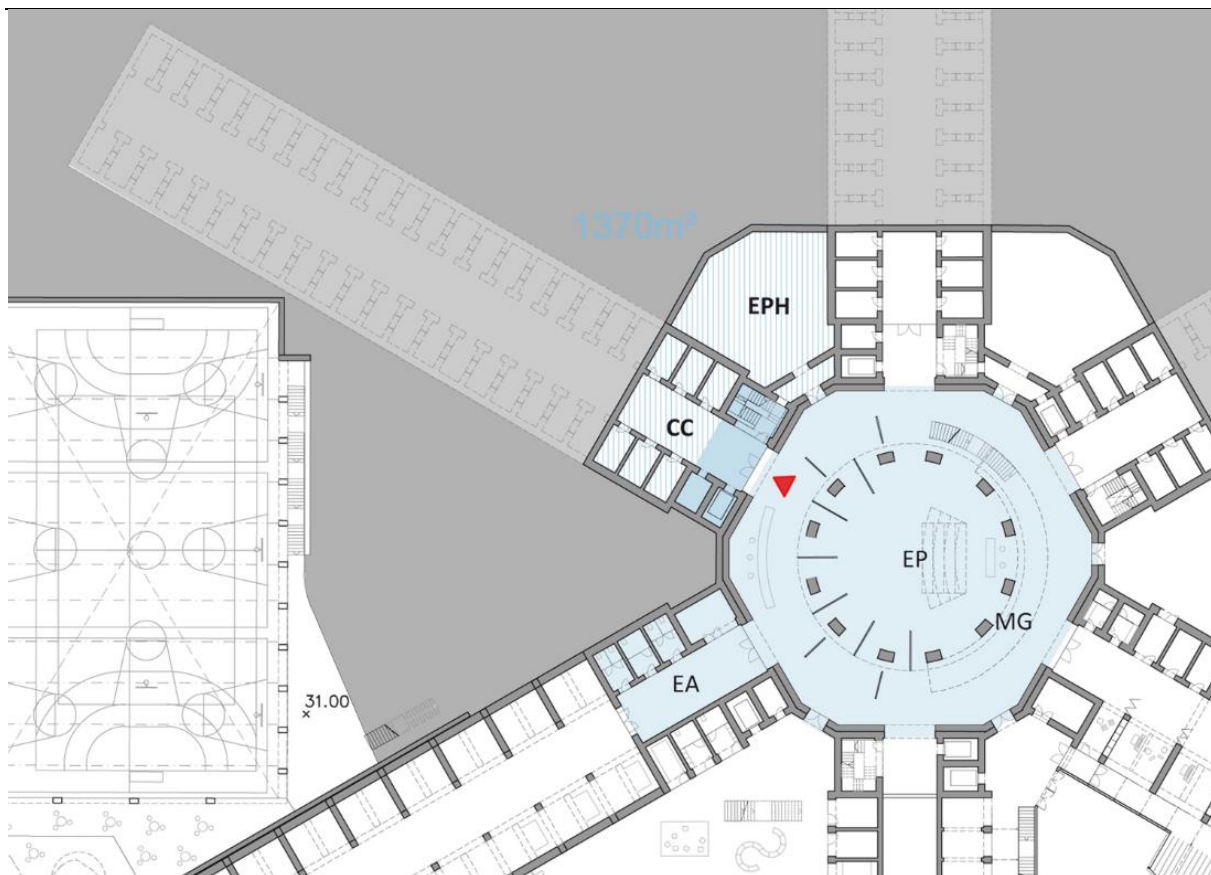
Planta sotterrani proposta +31,00m
