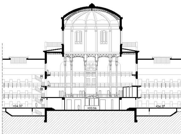
Fig. 7 Secció A-A' - Estat actual
