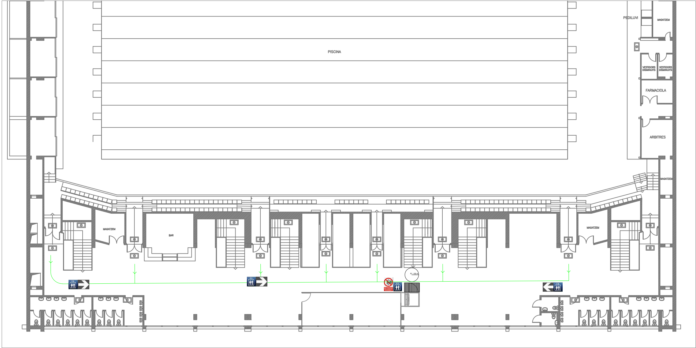
Planta primera. Recorreguts fins l'elevador. E: 1/250
