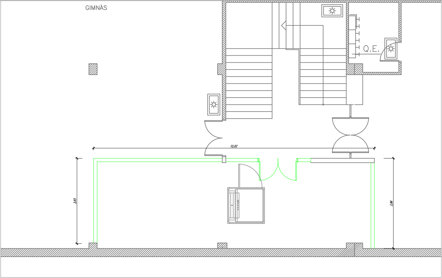
P. Soterrània. E: 1/100
