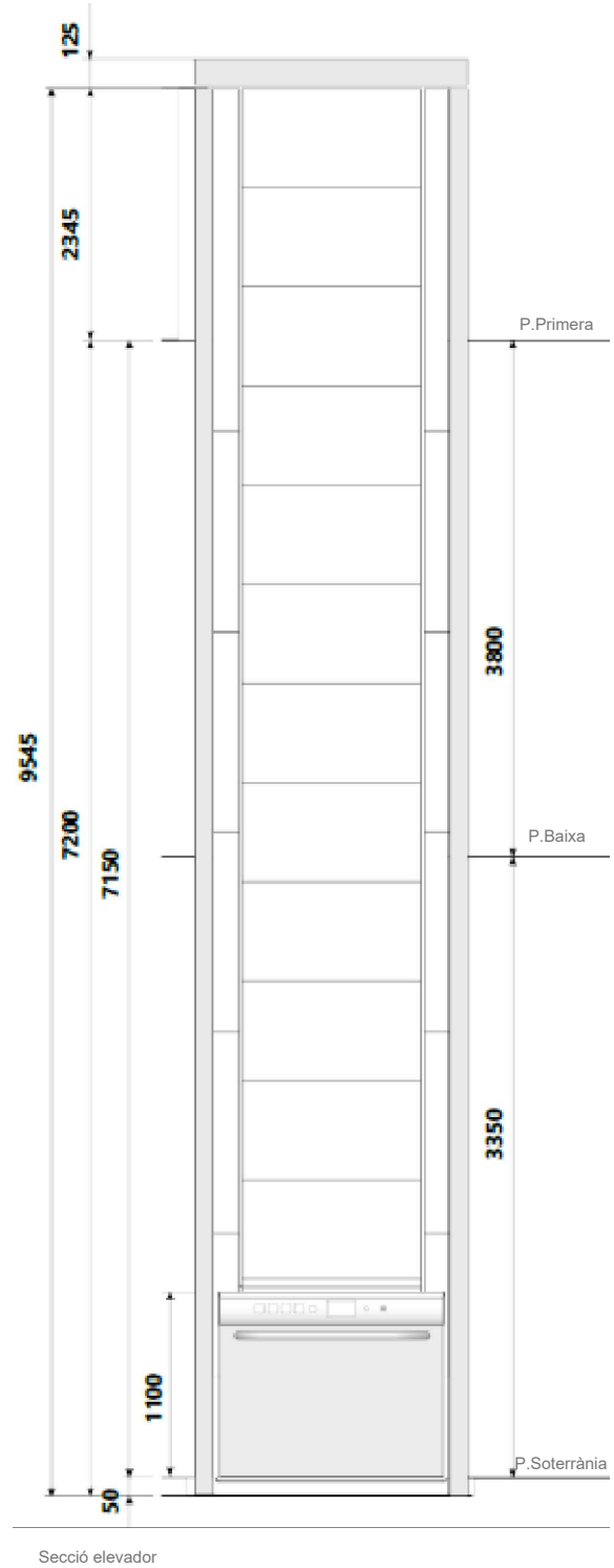
Secció elevador
