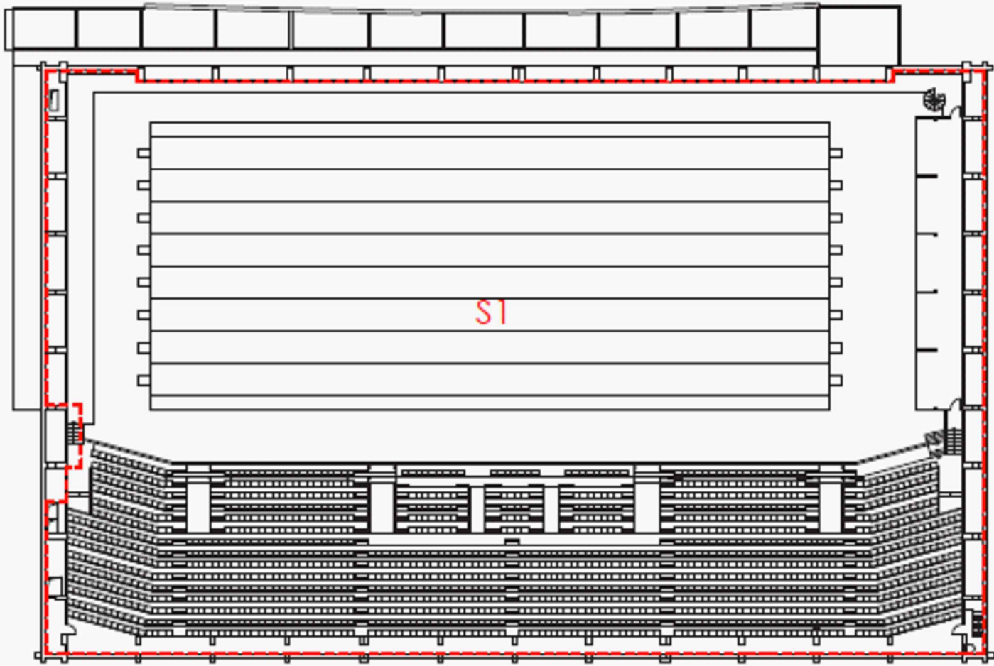
Aquest plànol de planta grades de base és el facilitat per la gestora del Centre que forma part del seu Pla d'Autoprotecció
