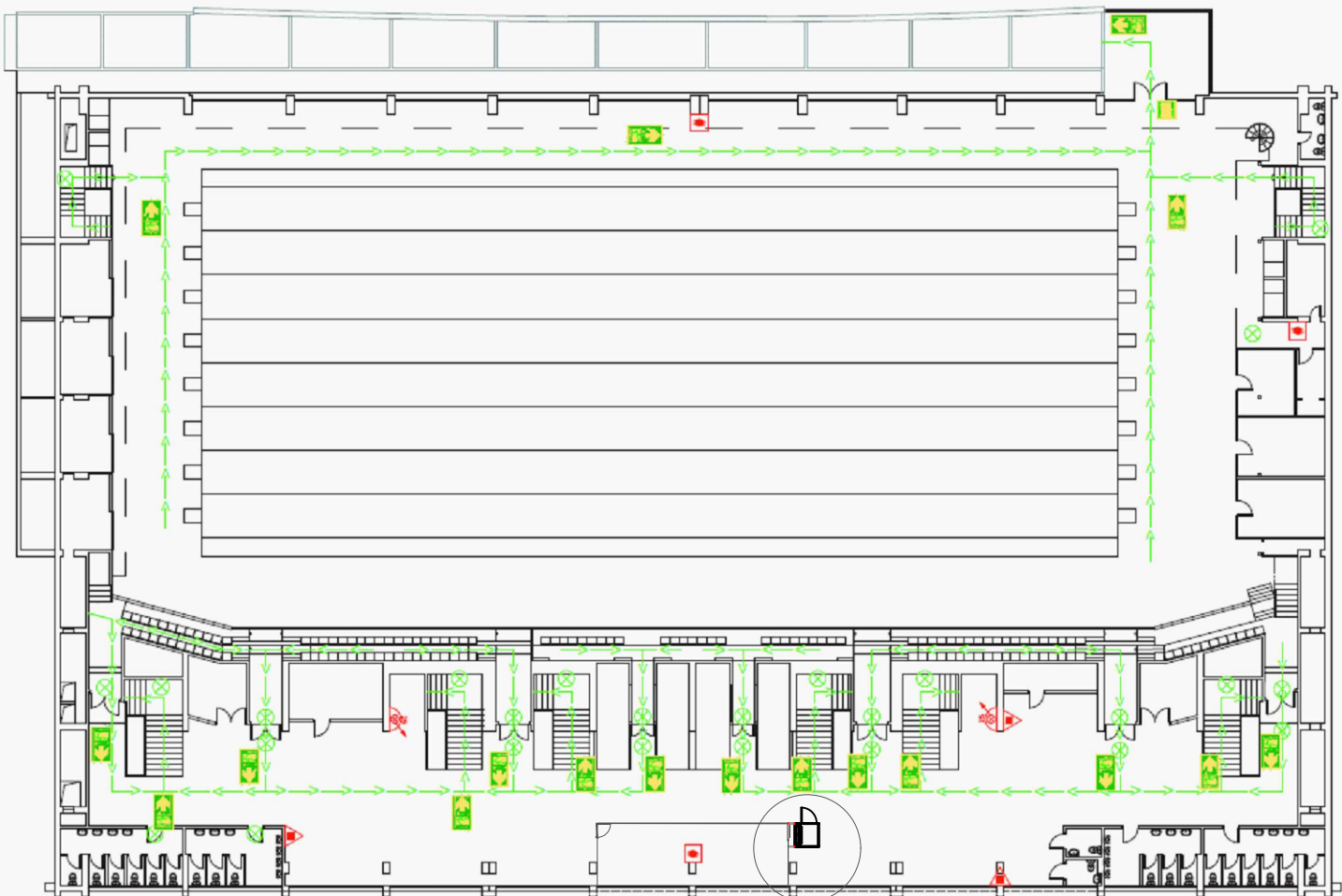
Plànol planta primera. Aquest plànol de base, és el facilitat per la gestora del Centre que forma part del seu Pla d'Autoprotecció
