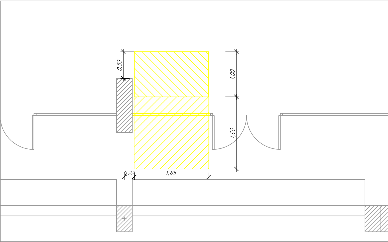
Planta baixa
