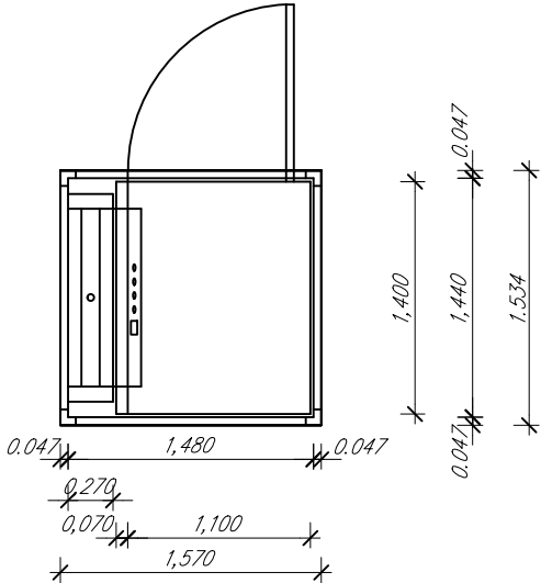
Dimensions elevador
