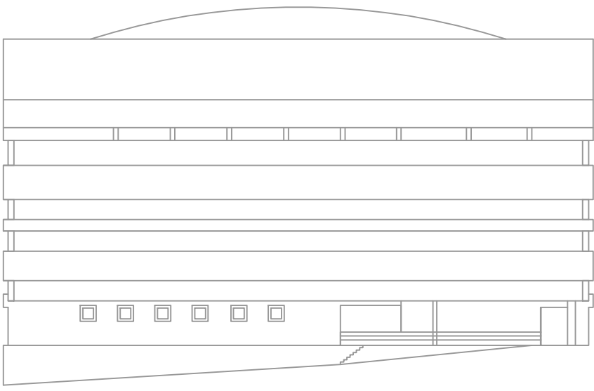
Façana nord-est (lateral), pati interior d'illa. E: 1/400
