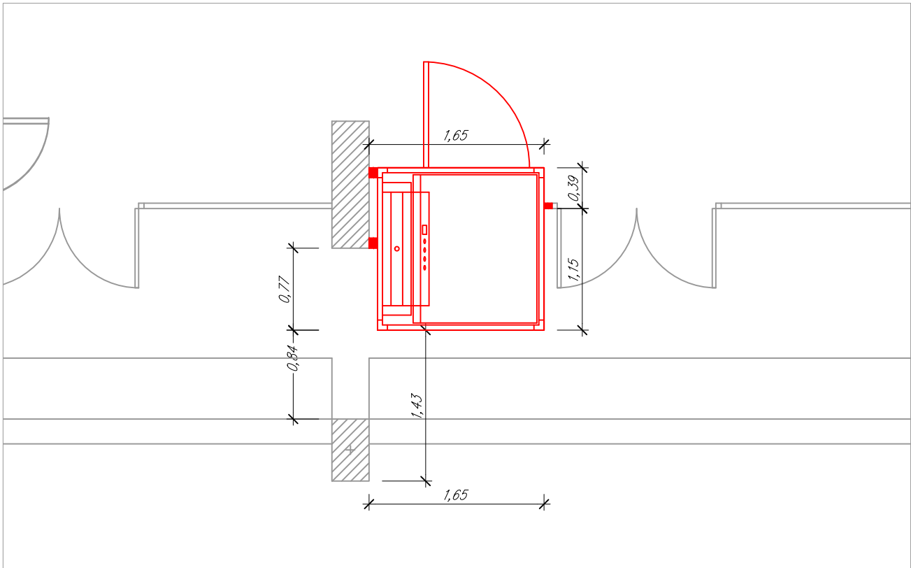
Planta baixa
