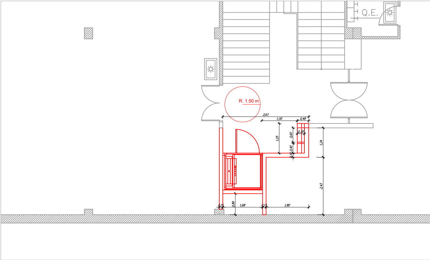
Planta soterrània. Proposta estat final
