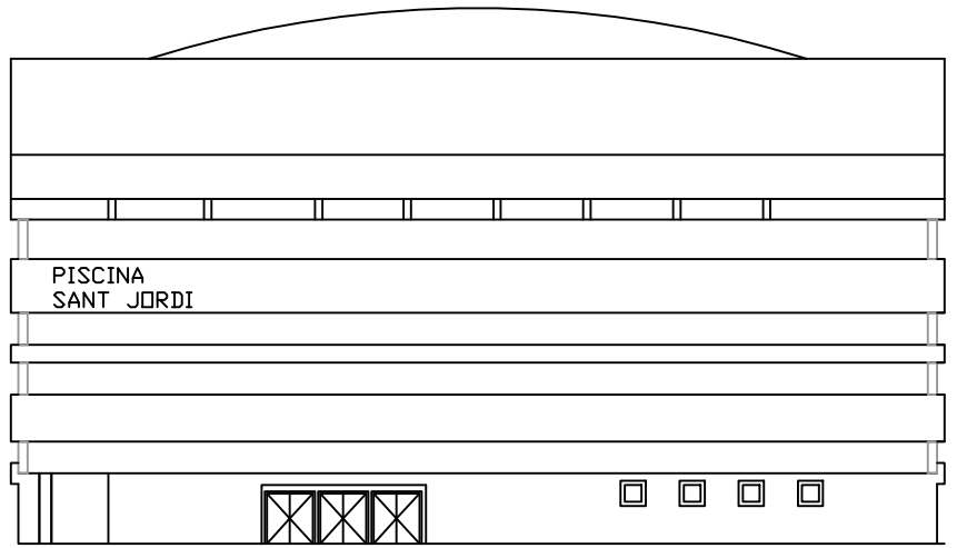
⌚ N Façana sudoest
