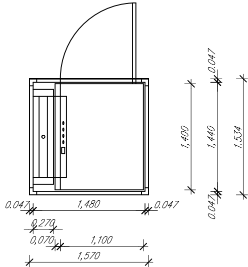
Dimensions elevador
