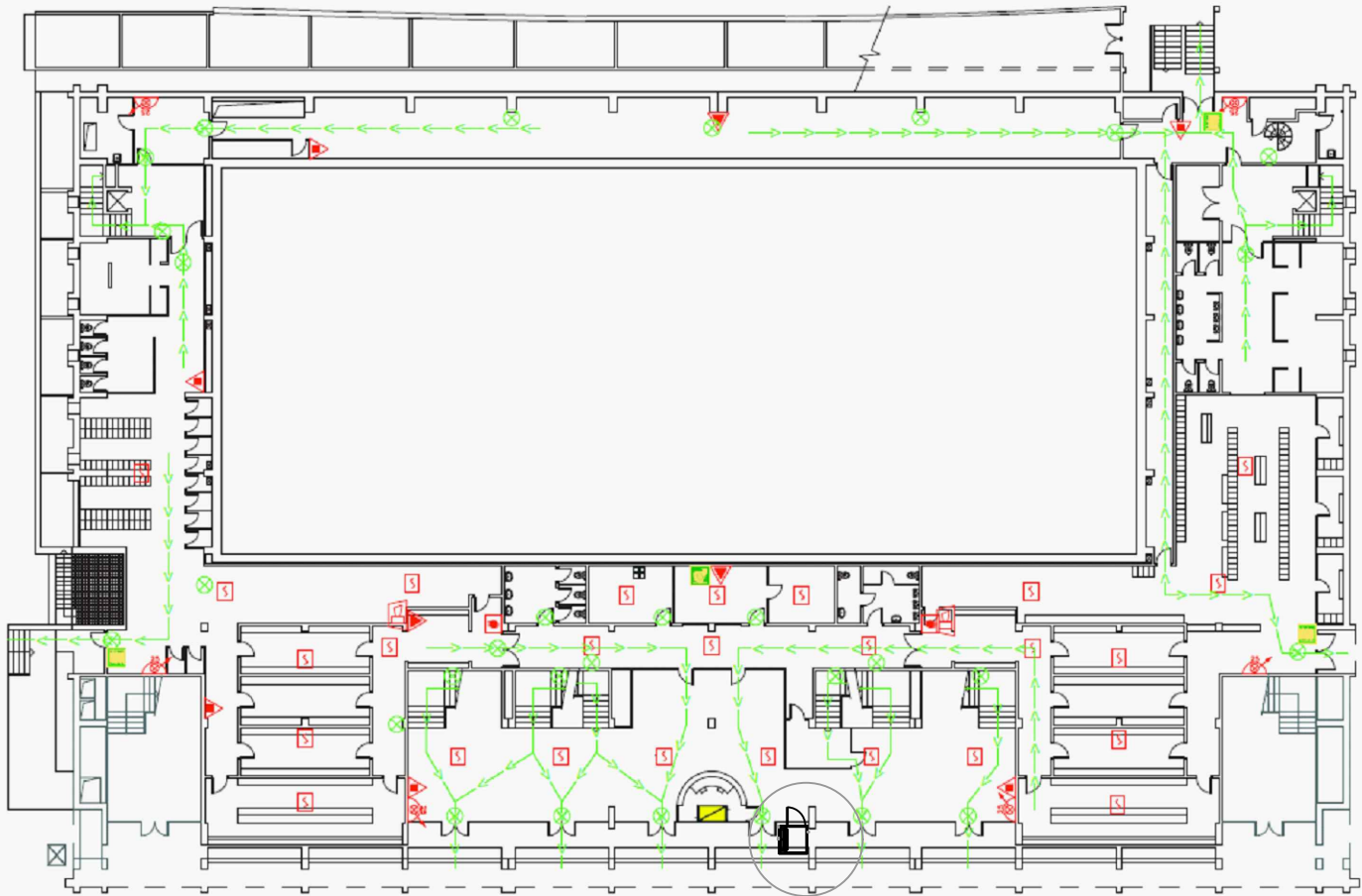
Plànol planta baixa. Aquest plànol de base, és el facilitat per la gestora del Centre que forma part del seu Pla d'Autoprotecció
