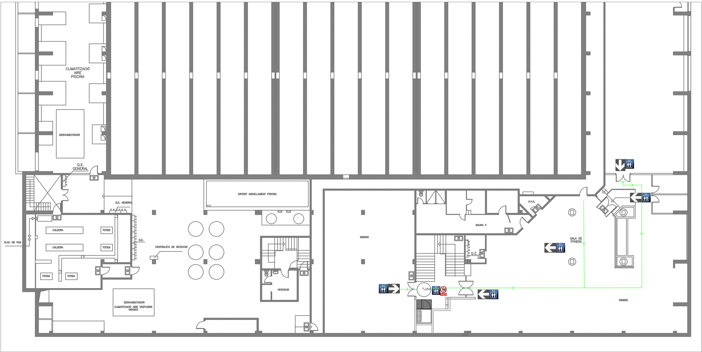
P. Soterrània. Situació elevador. E: 1/250
