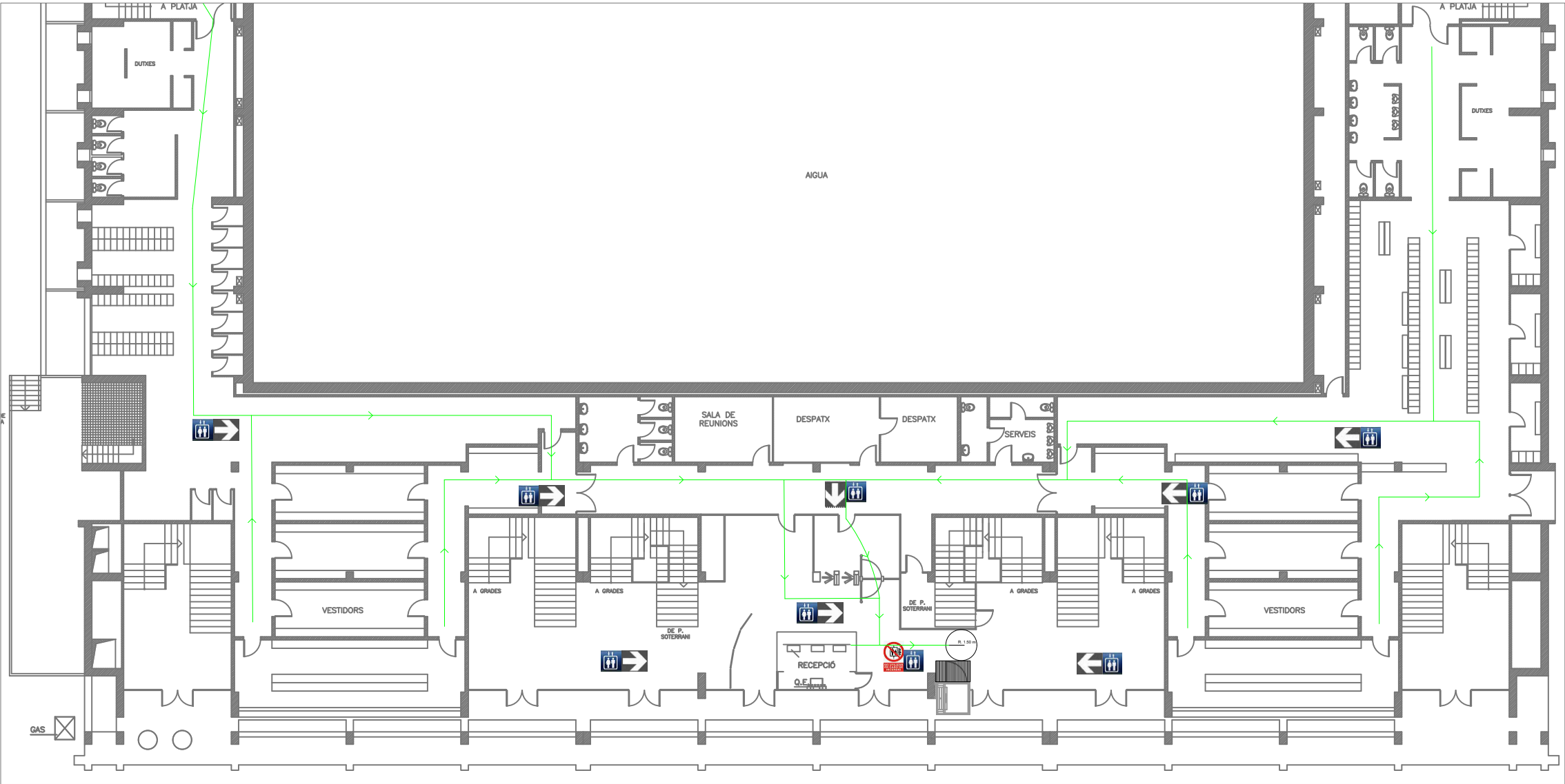
Planta baixa. Recorreguts fins l'elevador. E: 1/250
