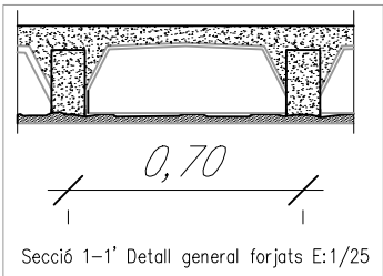
Secció 1-1' Detall general forjats E:1/25
