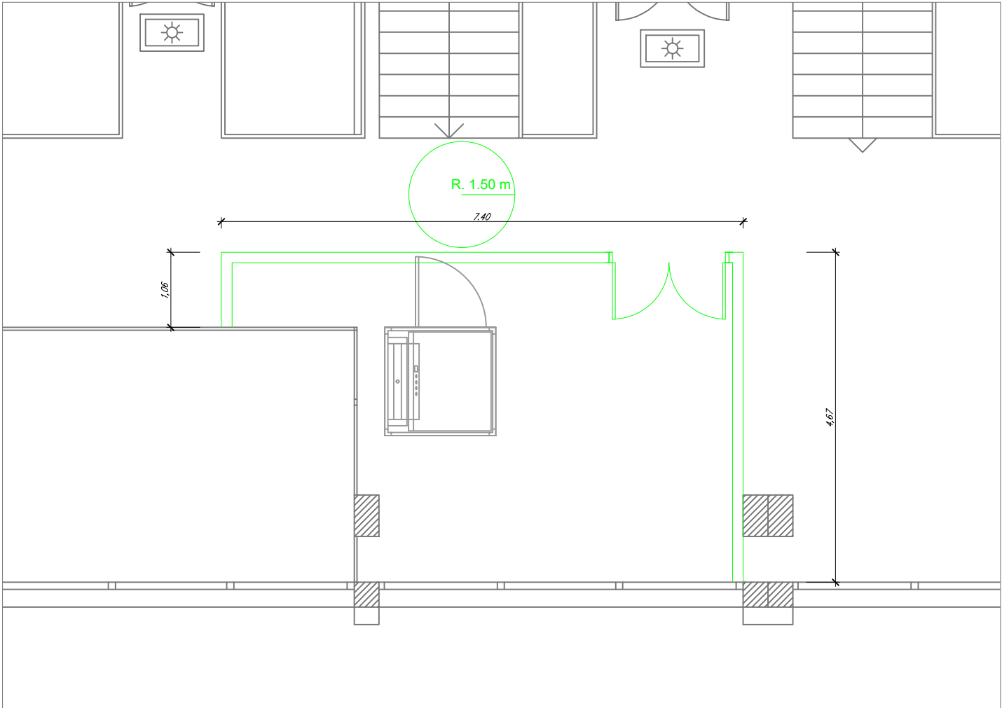
Planta primera. E: 1/75
