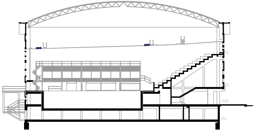
Secció A-A'. Estat actual
