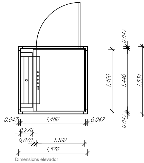
Dimensions elevador
