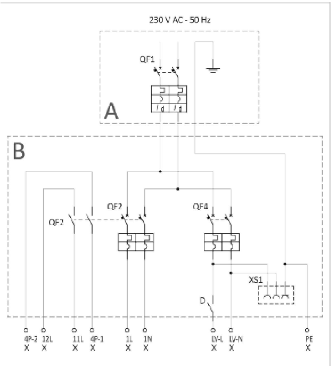
Esquema elèctric proposat per l'elevador
