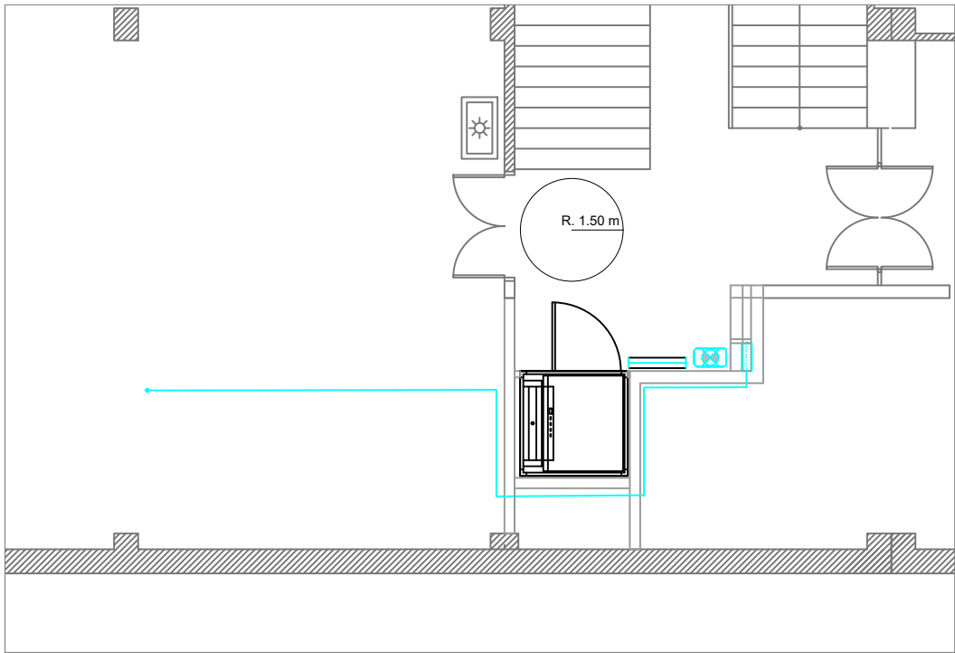
P. Soterrània
