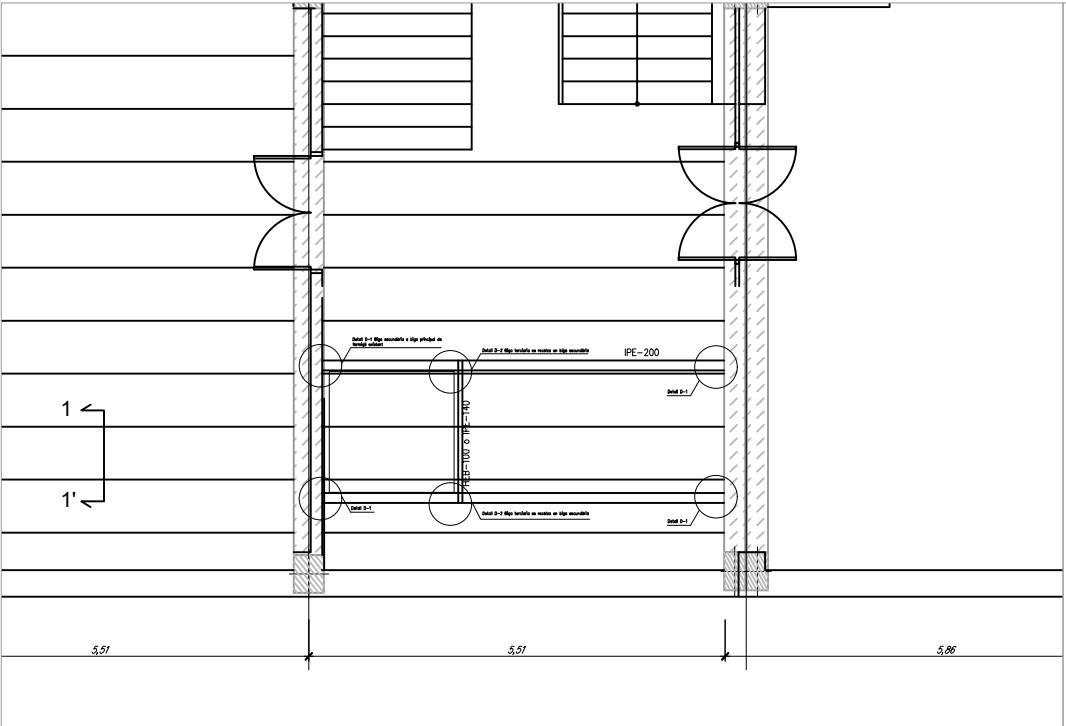
Estructura forjat sotre planta soterrània. Reforç estructura, Estat final. E: 1/100
