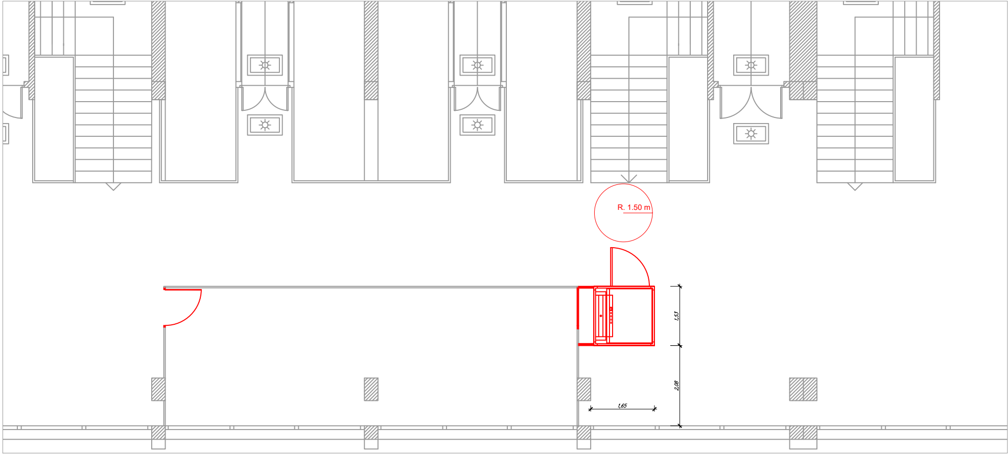
Planta primera. Proposta estat final
