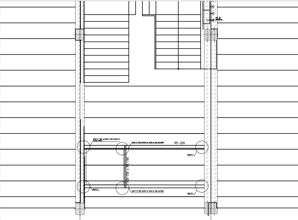
Estructura forjat sotre planta baixa. Reforç estructura, Estat final. E: 1/100
