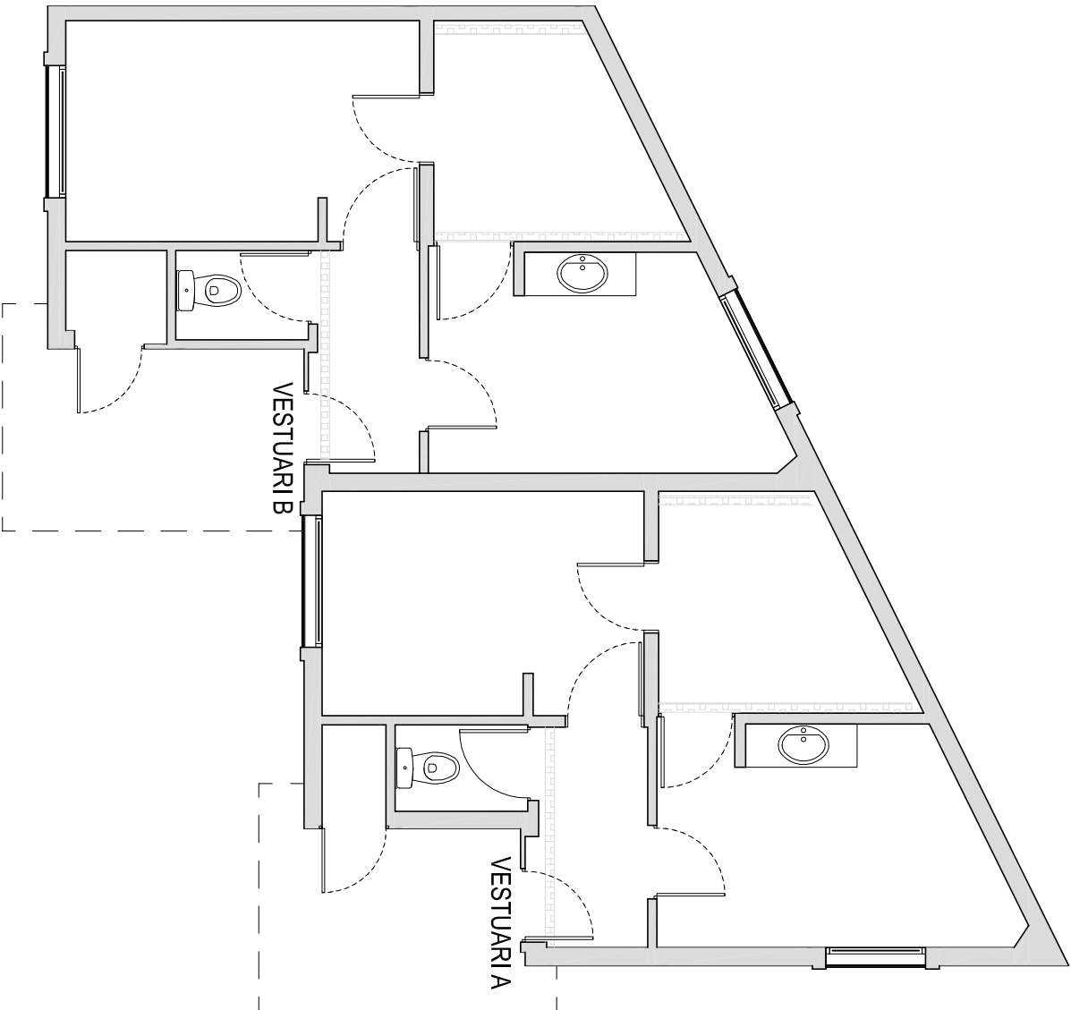
Planta E:1/75
