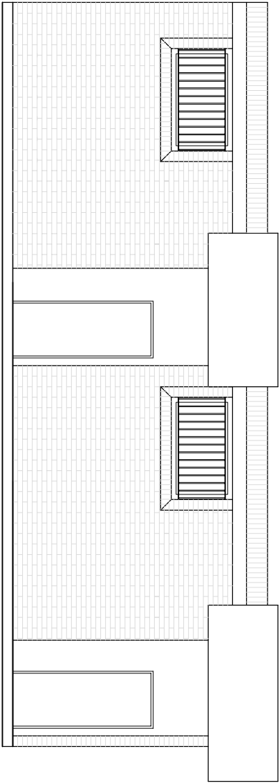
Façana Ppal E:1/75
