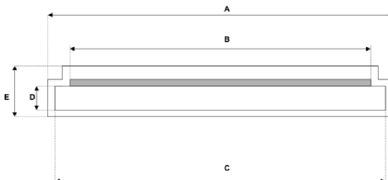
Figura 3. Esquema del protector de empalme
