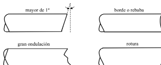
Figura 2. Corte de la fibra óptica
