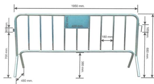
Tanca mòbil metàl·lica "d'obra" (TMM)
