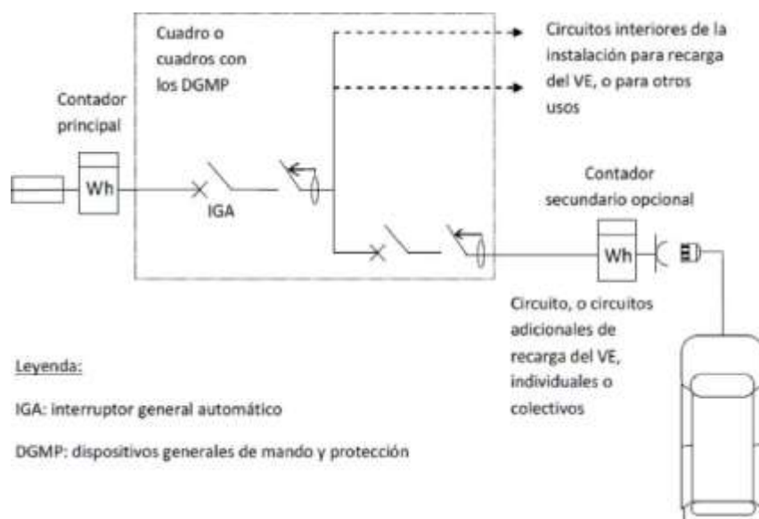
Imagen 9.1. Esquema 4b: instalación con circuito adicional
