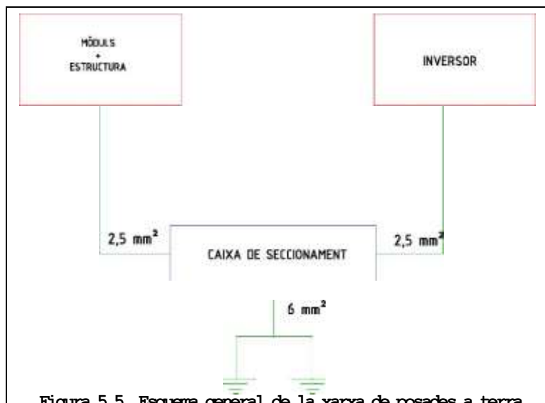
Figura 5.5. Esquema general de la red de puestas a tierra
