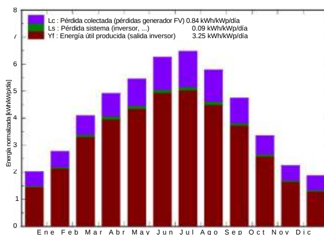
Producciones normalizadas (por kWp instalado): Potencia nominal 9.90 kWp
